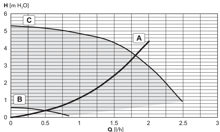
рис. 33 - Потери нагрузки/напор циркуляционного насоса SILVER 24T
