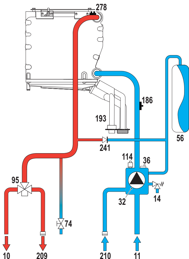
рис. 32 - Гидравлический контур
