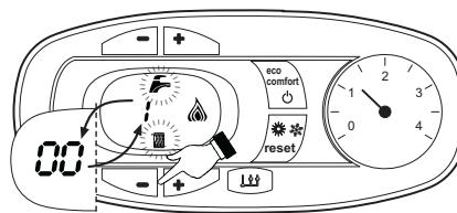
fig. 24 - Mode TEST (puissance chauffage = 100%)
