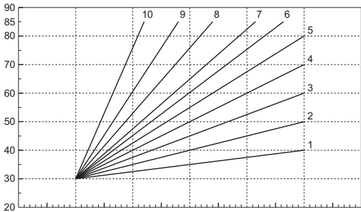
fig. 11 - Curvas de compensación
