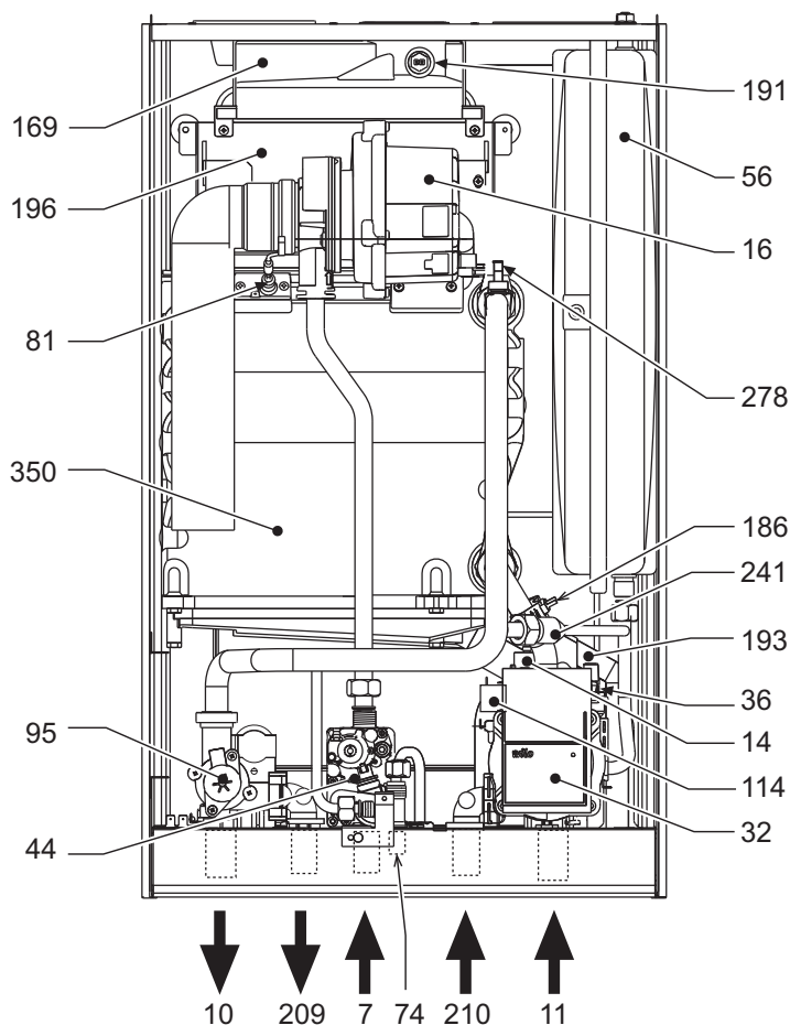
рис. 31 - Общий вид
