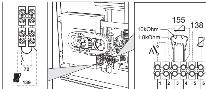
fig. 14 - Acceso a la regleta eléctrica
