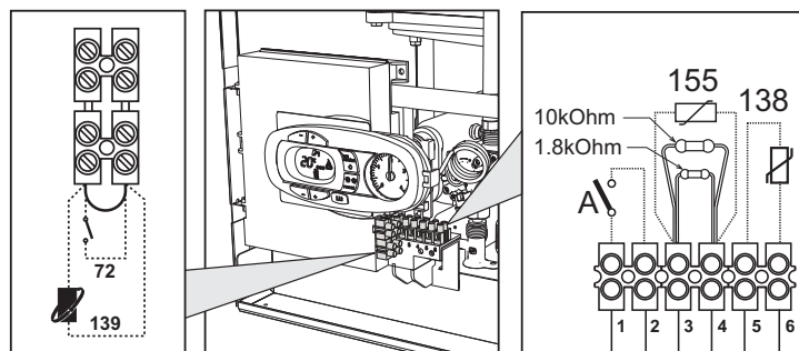
fig. 14 - Accesso alla morsettiera
