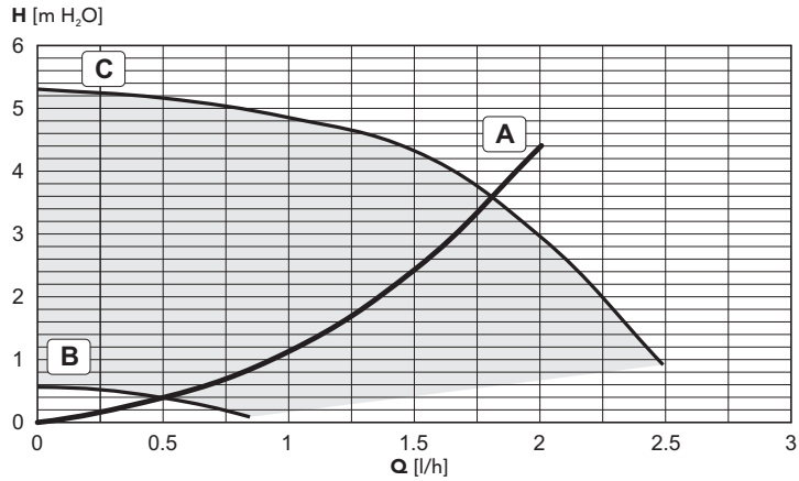
fig. 33 - Pertes de charge/pression circulateur SILVER 24T
