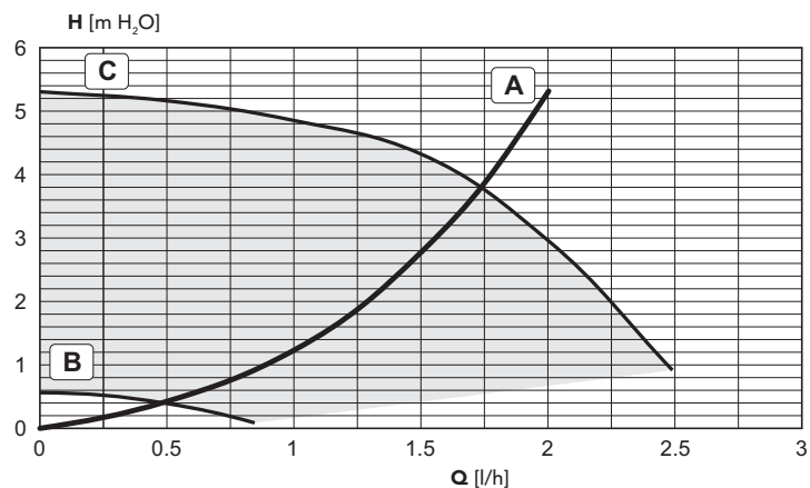
fig. 34 - Pérdidas de carga / altura de impulsión circulador SILVER 34T
