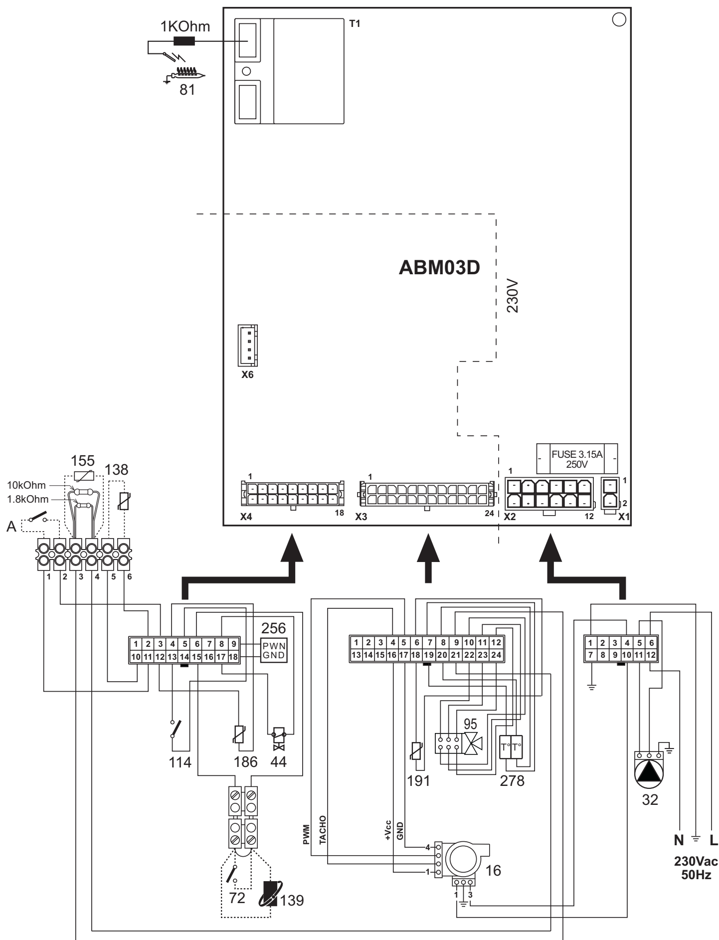
fig. 35 - Wiring diagram
