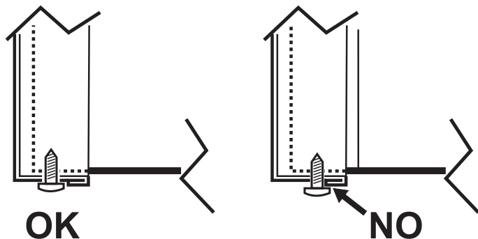
fig. 26 - Position correcte du panneau avant
