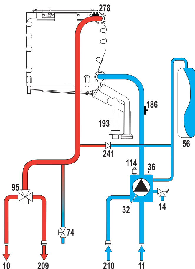
fig. 32 - Circuito idraulico
