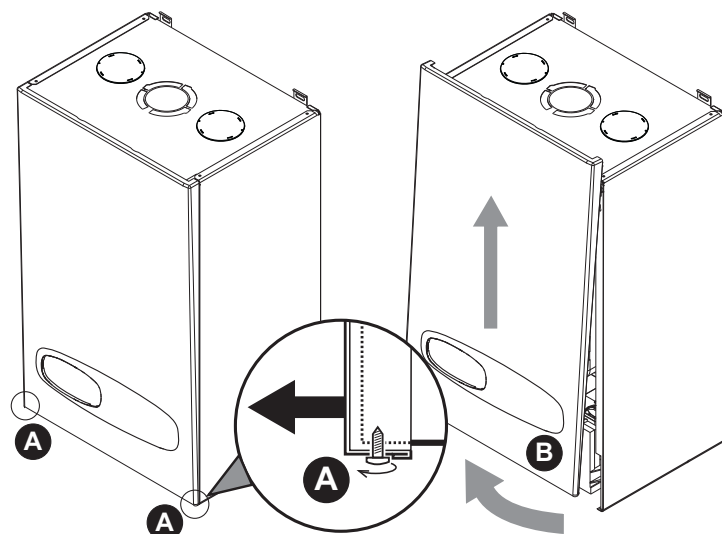
fig. 25 - Apertura pannello frontale
