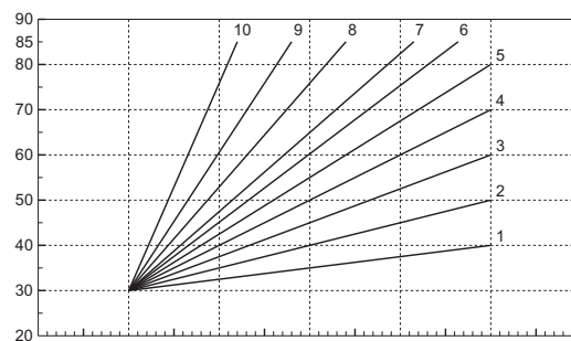
рис. 11 - Компенсационные характеристики
