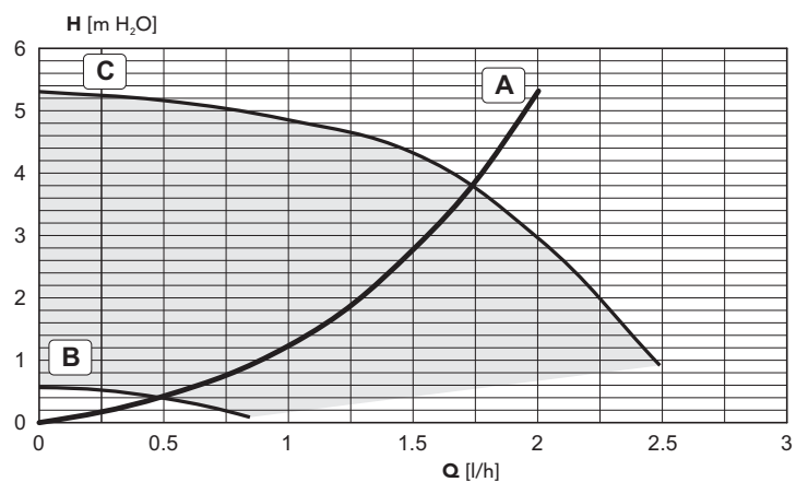
рис. 34 - Потери нагрузки/напор циркуляционного насоса SILVER 34T
