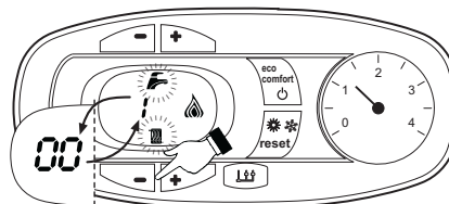
fig. 24 - Modo TEST (potencia de calefacción = 100 %)
