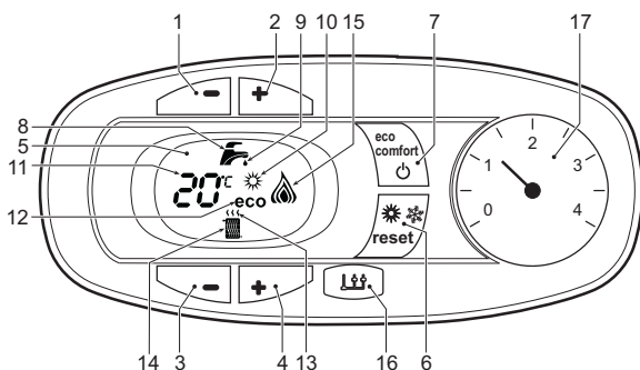
fig. 1 - Panneau de contrôle
