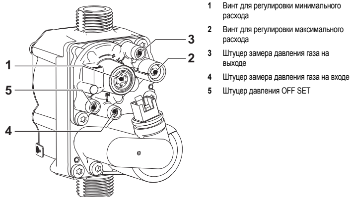
рис. 23 - Газовый клапан
