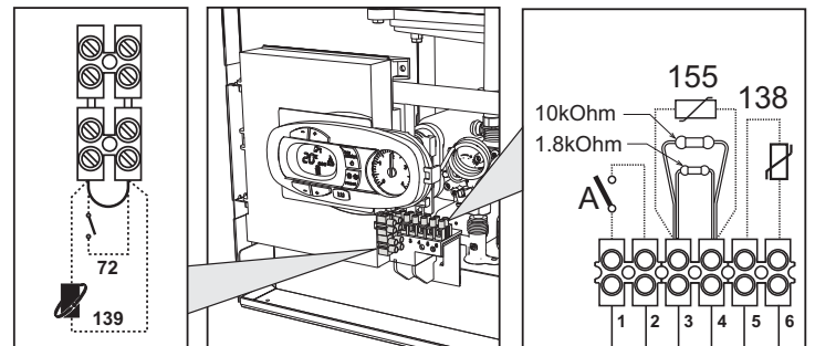
fig. 14 - Accès au bornier
