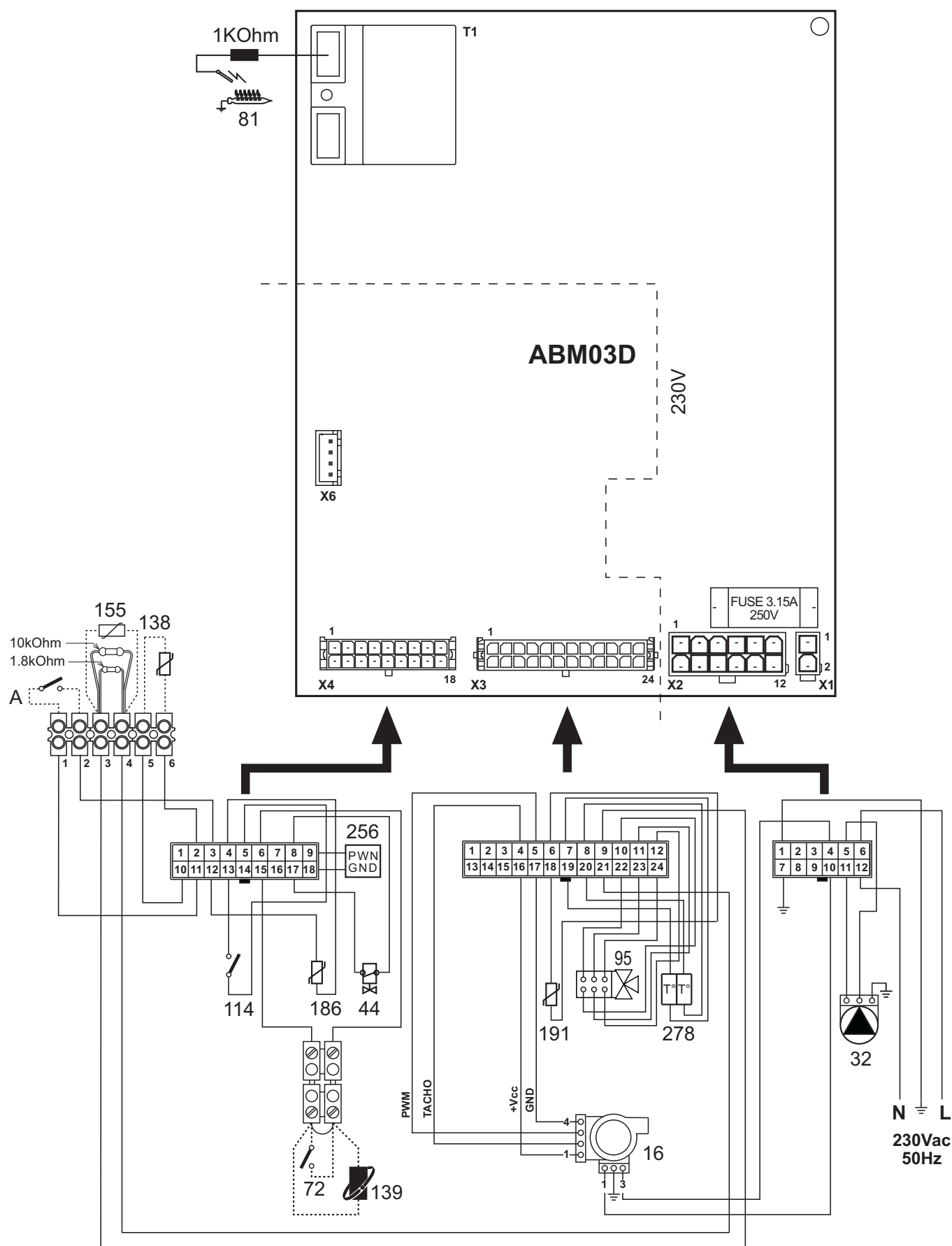
fig. 35 - Esquema eléctrico
