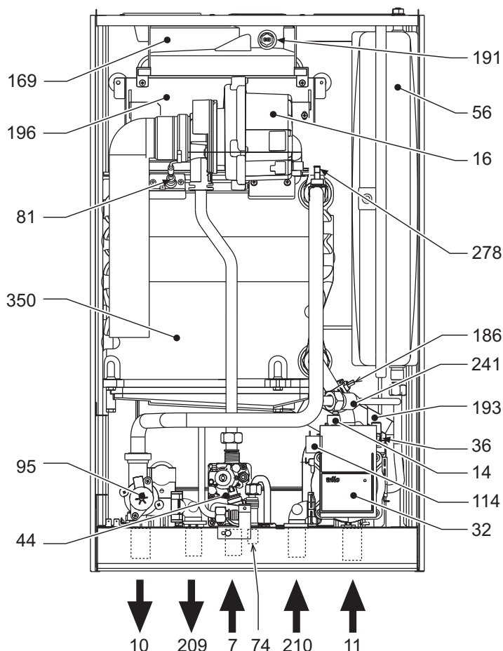
fig. 31 - Vue générale
