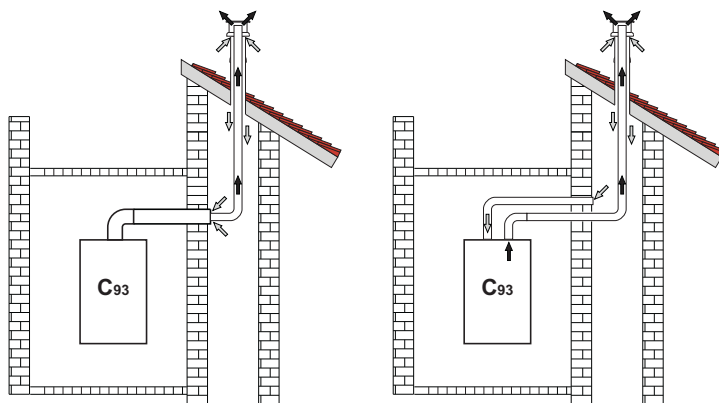
рис. 19 - Примеры подсоединения к дымоходам (→ = Воздух / → = Дымовые газы)
