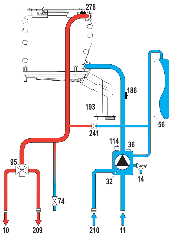
fig. 32 - Circuit hydraulique
