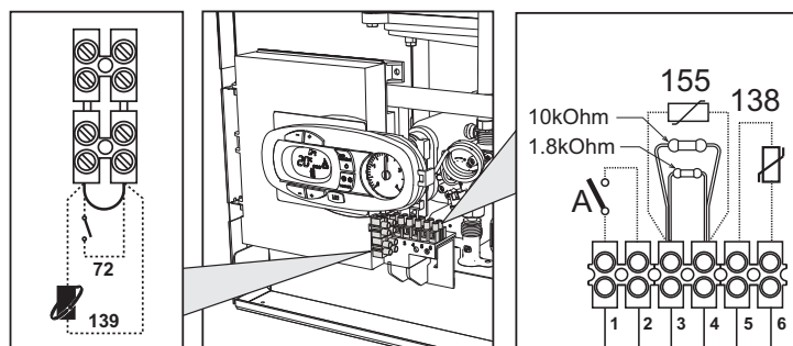
рис. 14 - Доступ к клеммной коробке
