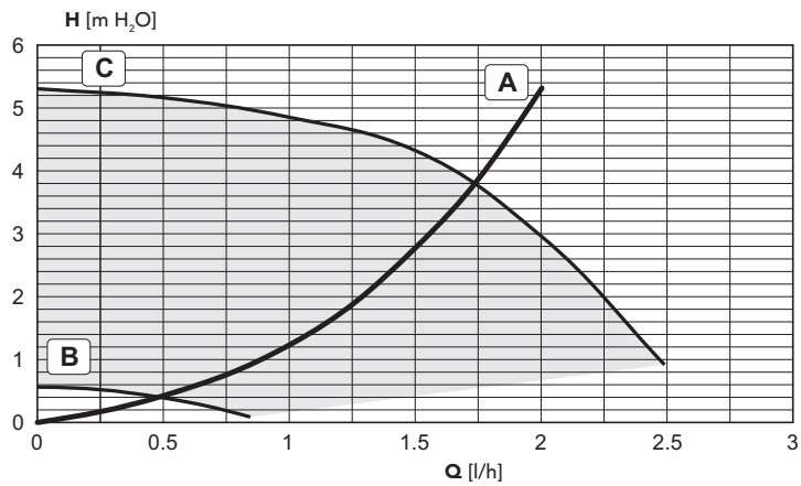
fig. 34 - Perdite di carico / prevalenza circolatore SILVER 34T
