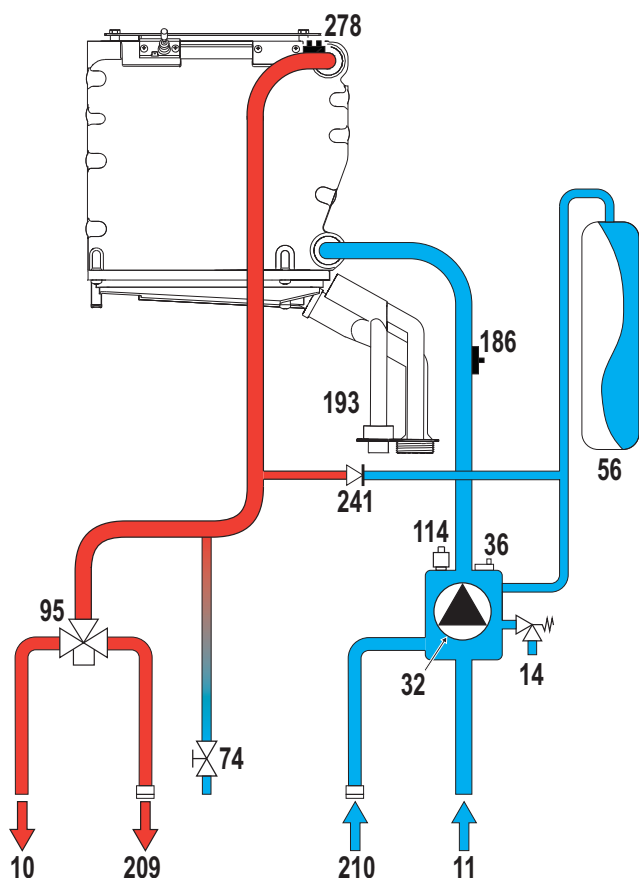
fig. 32 - Circuito de agua
