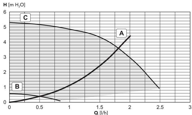
fig. 33 - Pérdidas de carga/altura de impulsión circulador SILVER 24T
