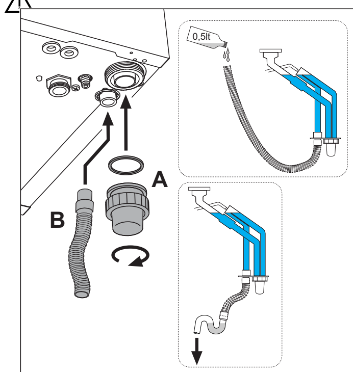
рис. 20 - Подсоединение трубы для слива конденсата
