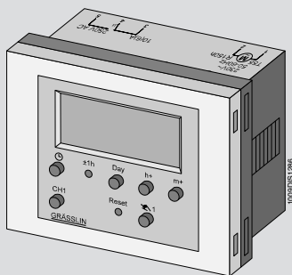
Orologio programmatore (a richiesta)
