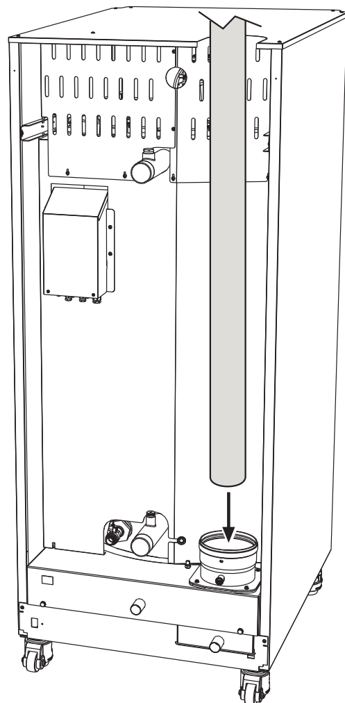
fig. 57- Fume outlet
