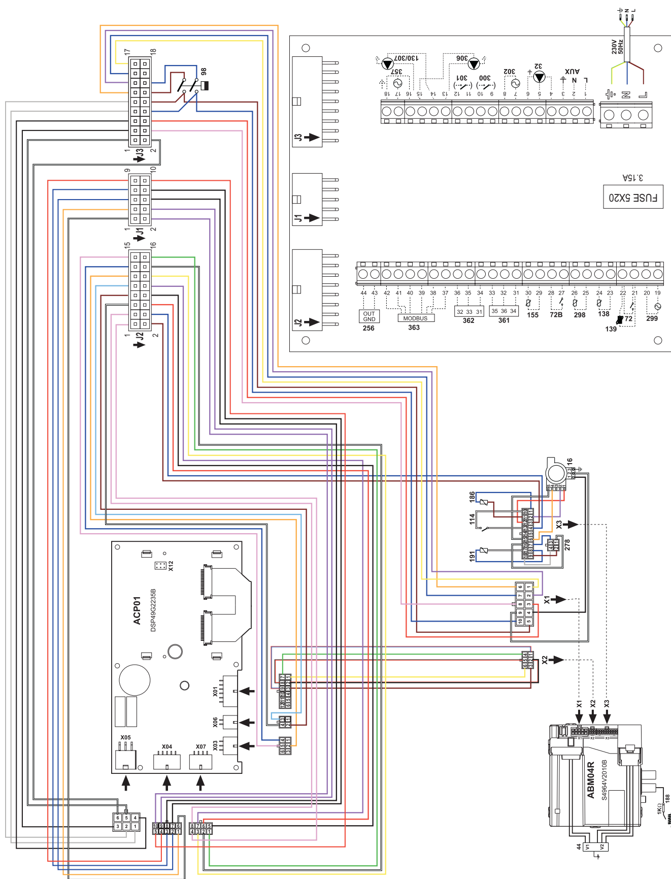
fig. 93- Schéma électrique CLOVER 125 et 160
