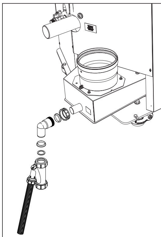
fig. 58- Raccordement de l'évacuation des condensats
