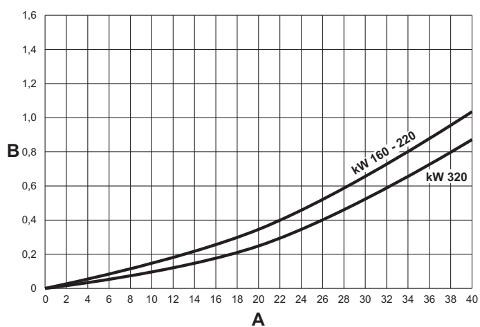
рис. 88 - Диаграмма утери напора в моделях 160, 220 и 320
