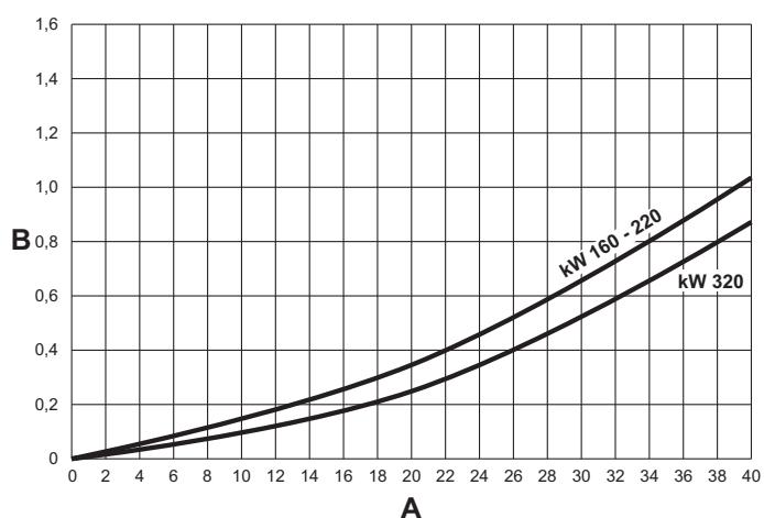
fig. 88 - Diagramma perdita di carico modelli 160, 220 e 320
