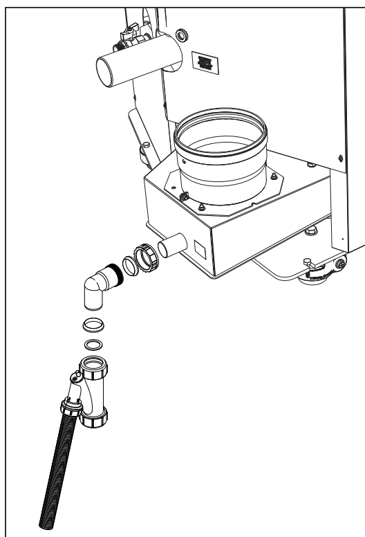
fig. 58- Conexión de la descarga de condensado
