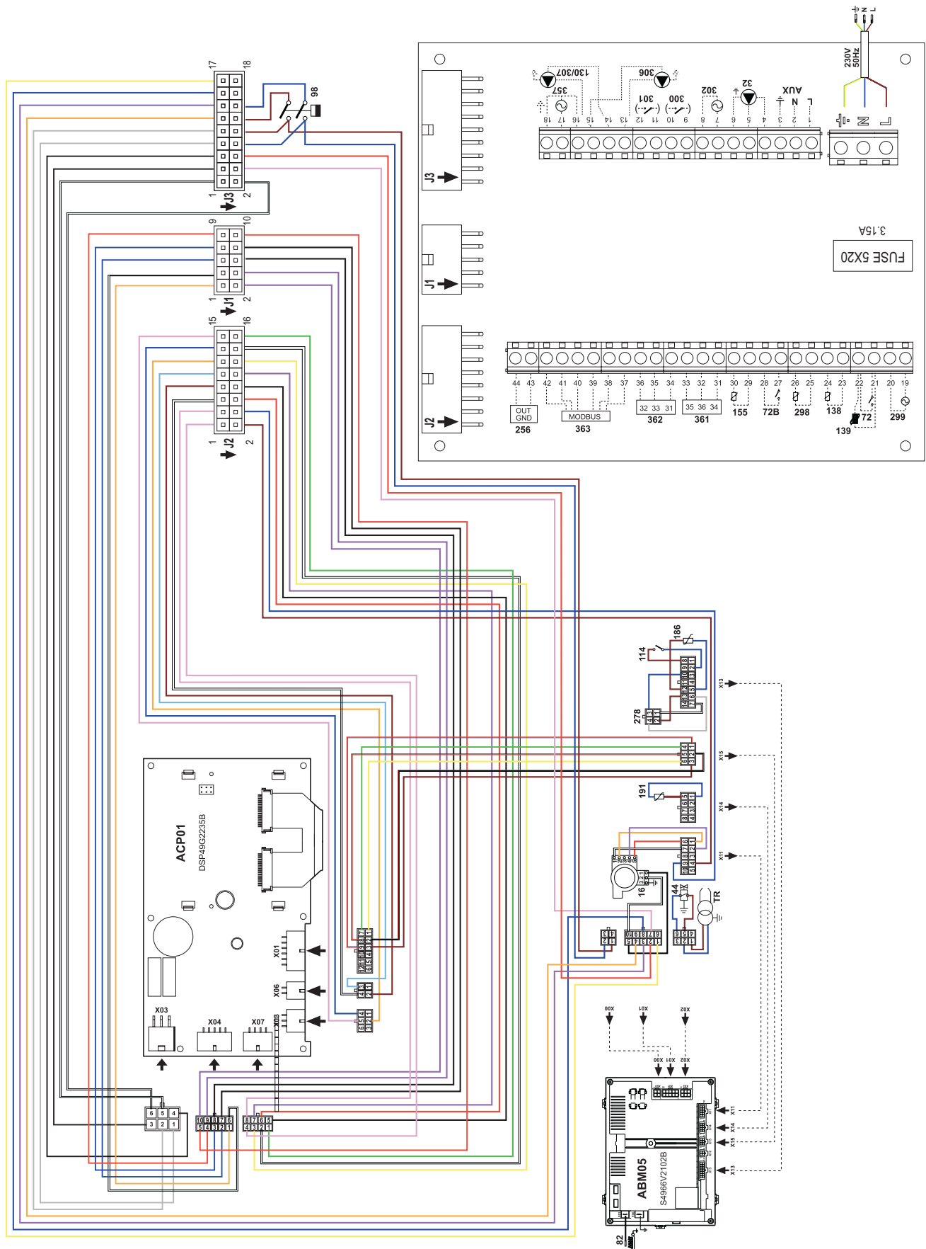
fig. 94- Schéma électrique CLOVER 220/320
