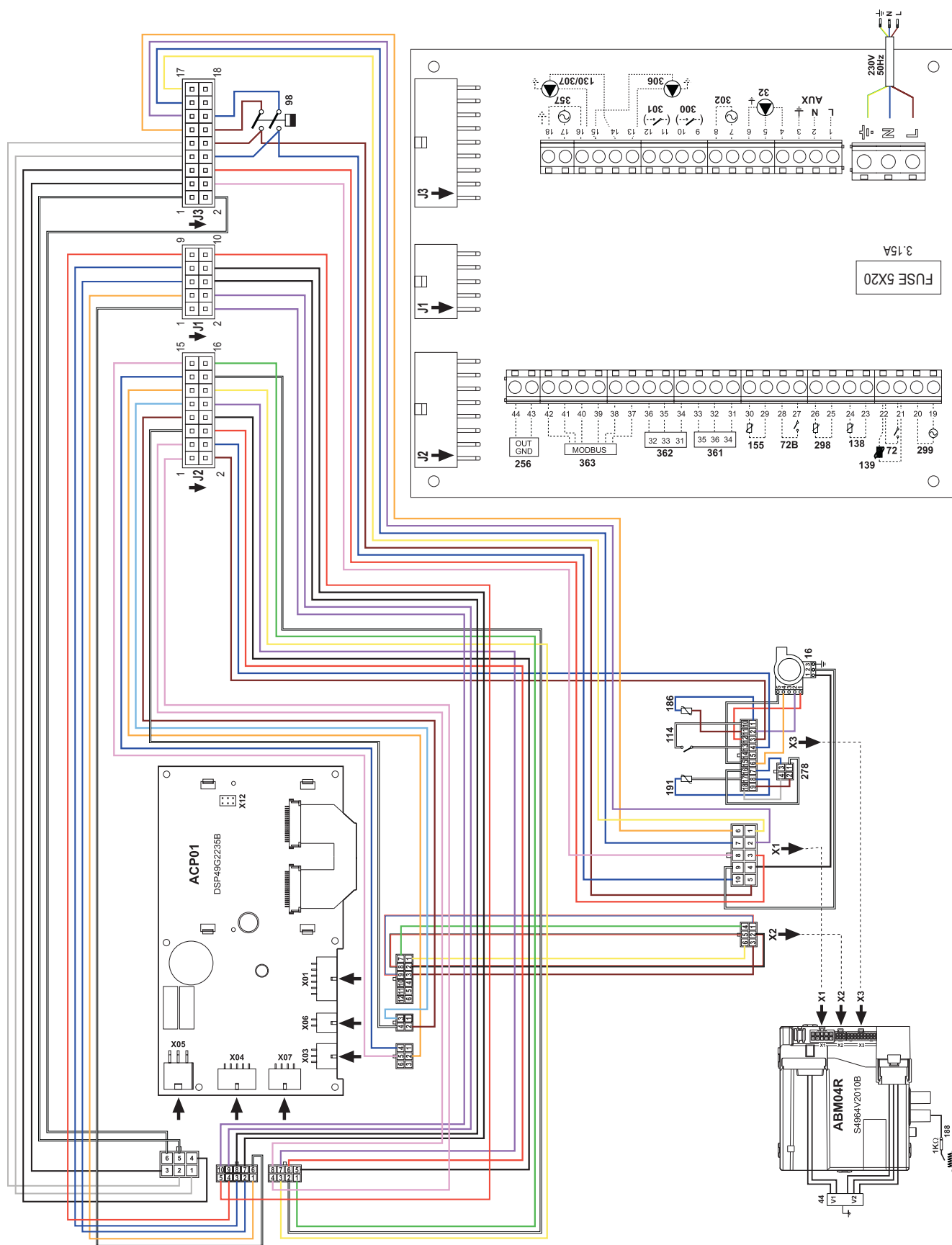
fig. 93- Esquema eléctrico CLOVER 125 y 160
