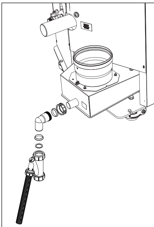
рис. 58- Подсоединение трубы для слива конденсата
