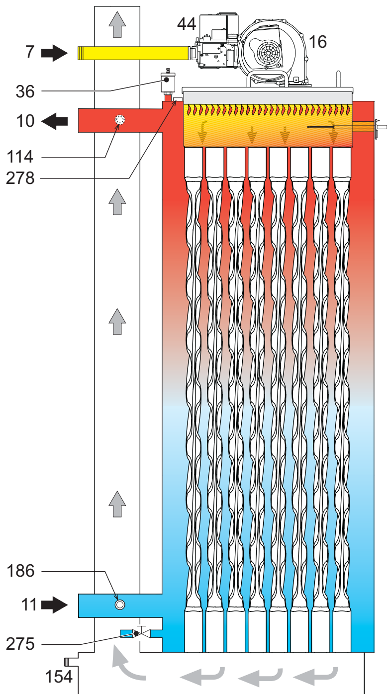
fig. 86 - Circuito idraulico
