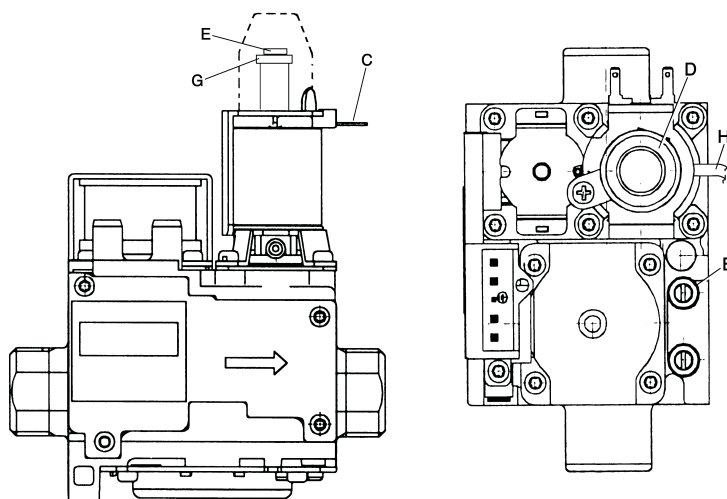
fig. 22 - Válvula de gas
