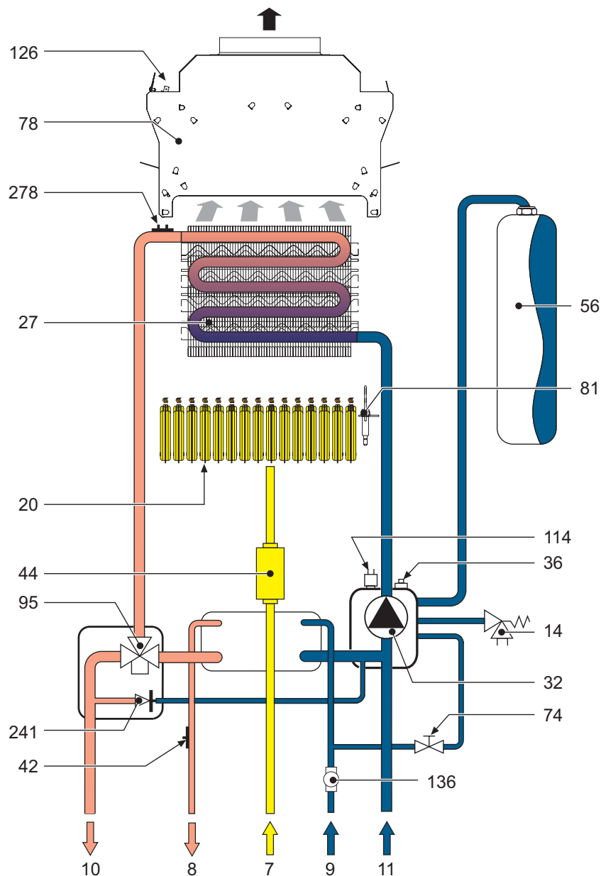
fig. 26 - Circuito idraulico
