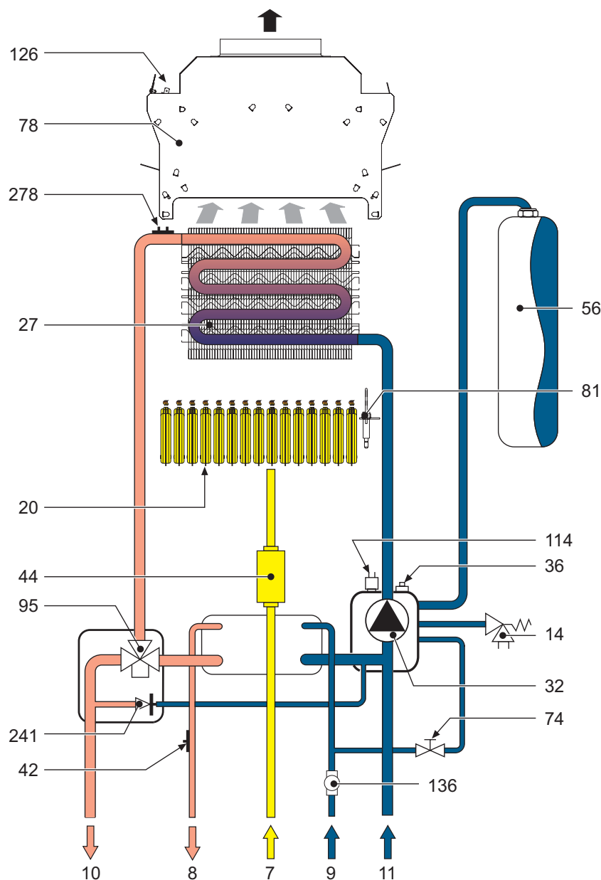
fig. 26 - Circuito hidráulico
