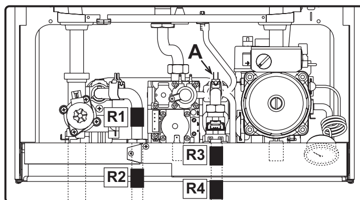
fig. 19 - Positionnement des résistances et du thermostat hors-gel
