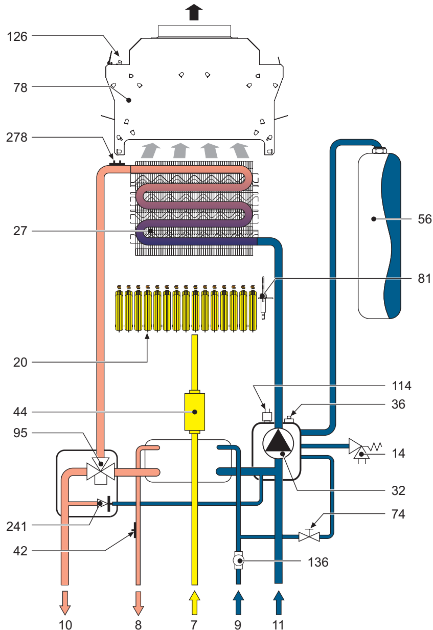
εικ. 26 - Υδραυλικό κύκλωμα
