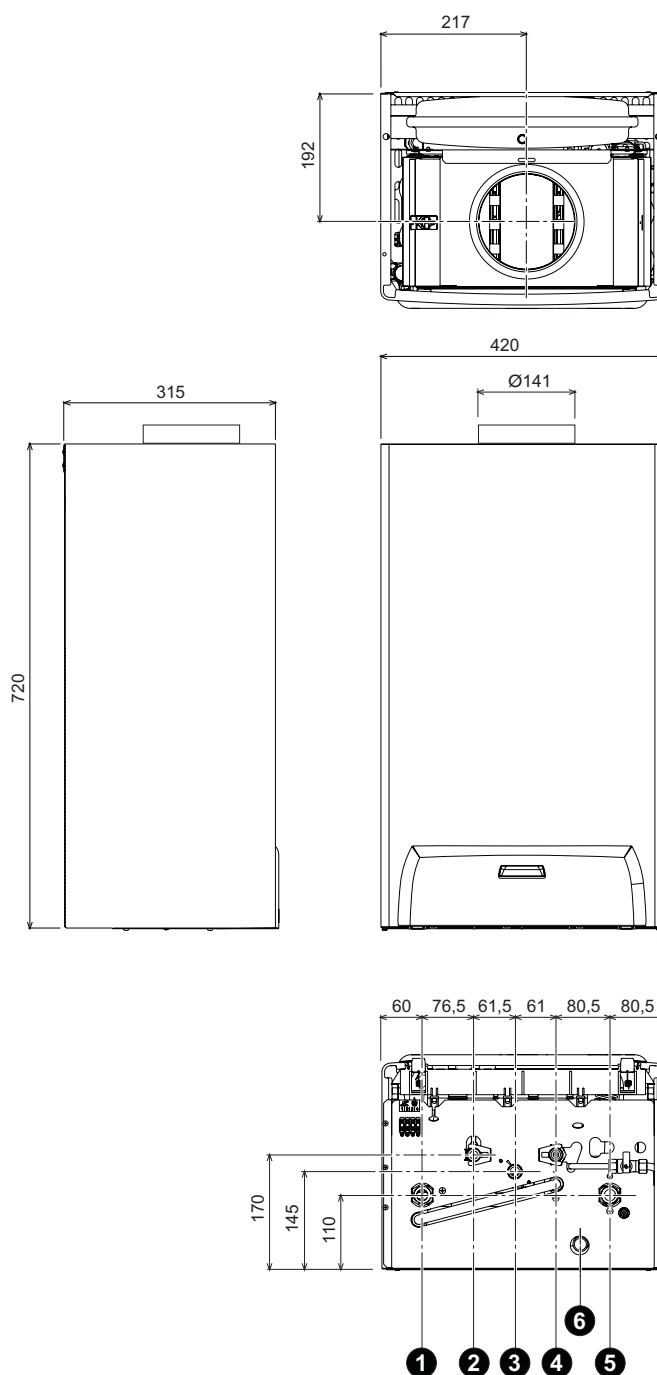
ΕΙΚ. 24 - Διαστάσεις και συνδέσεις
