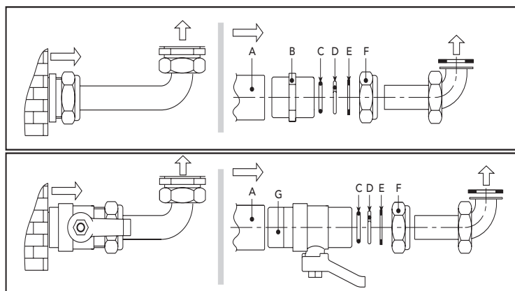
fig. 18 - Kit de raccordement
