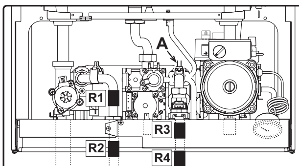
εικ. 19 - Τοποθέτηση θερμαντήρων και θερμοστάτη αντιπαγωτικού kit
