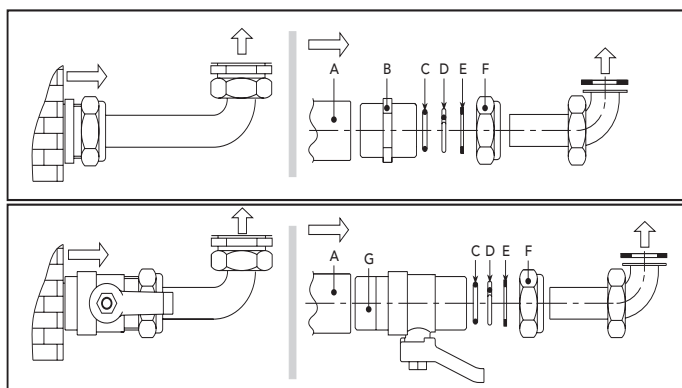
fig. 18 - Kit de conexión
