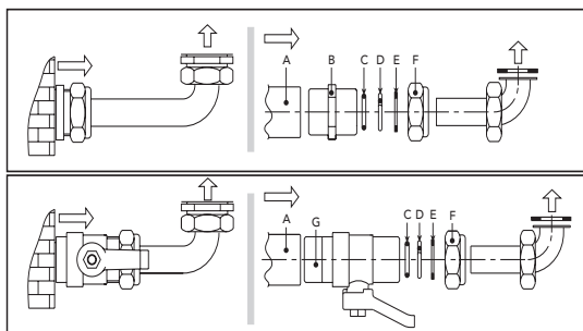
εικ. 18 - Κιτ σύνδεσης
