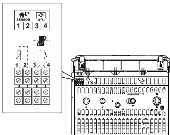
fig. 20 - Accès au bornier
