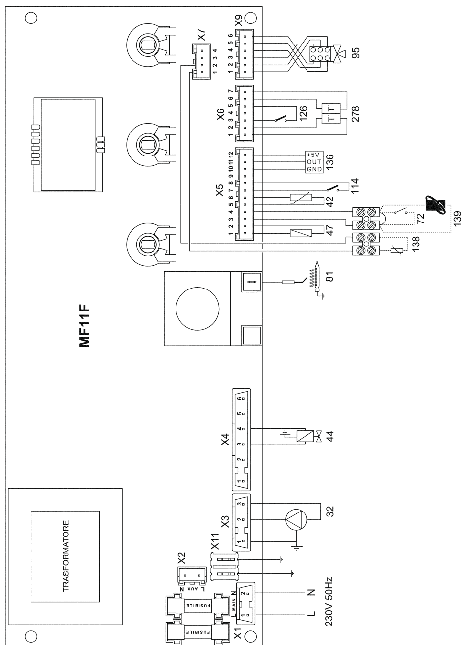
fig. 27 - Scema elettrico
