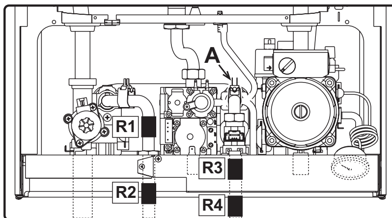
fig. 19 - Posicionamento dos aquecedores e do termostato anti-gelo
