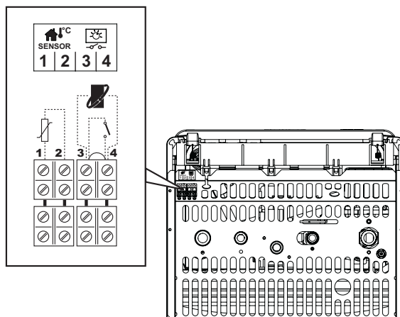
εικ. 20 - Πρόσβαση στην κλέμα σύνδεσης
