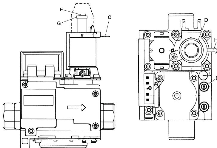
εικ. 22 - Βαλβίδα αερίου
