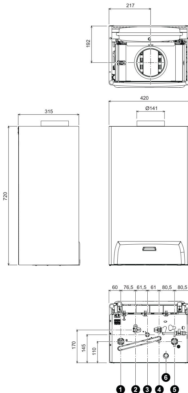
fig. 24 - Dimensiones y conexiones
