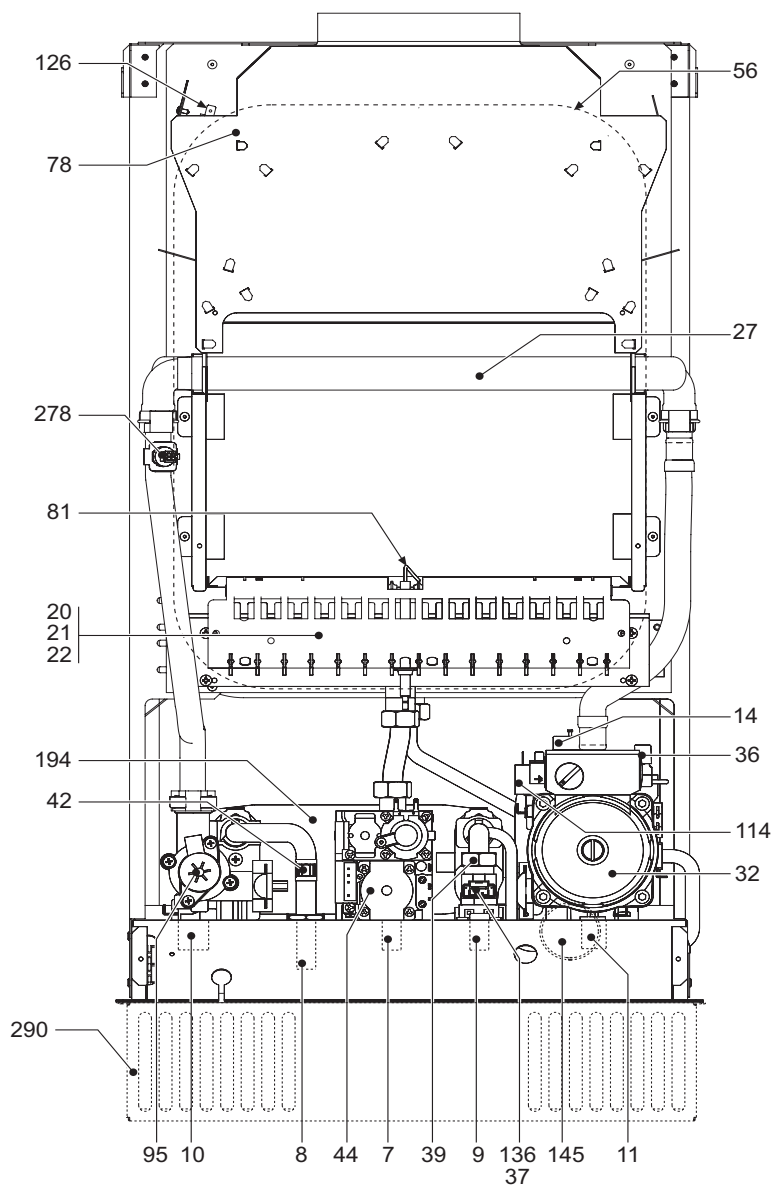
εικ. 25 - Γενική άποψη
