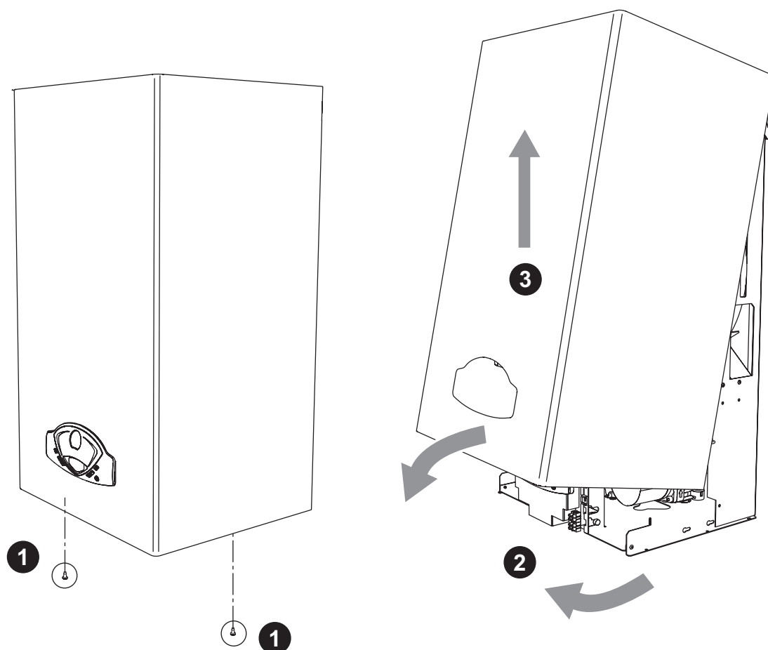
fig. 21 - Deschiderea carcasei
