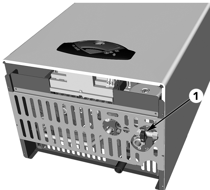
fig. 16 - Filling cock
