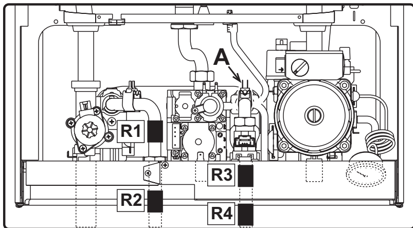
fig. 17 - Poziționarea încălzitoarelor și a termostatlui antiîngheț
