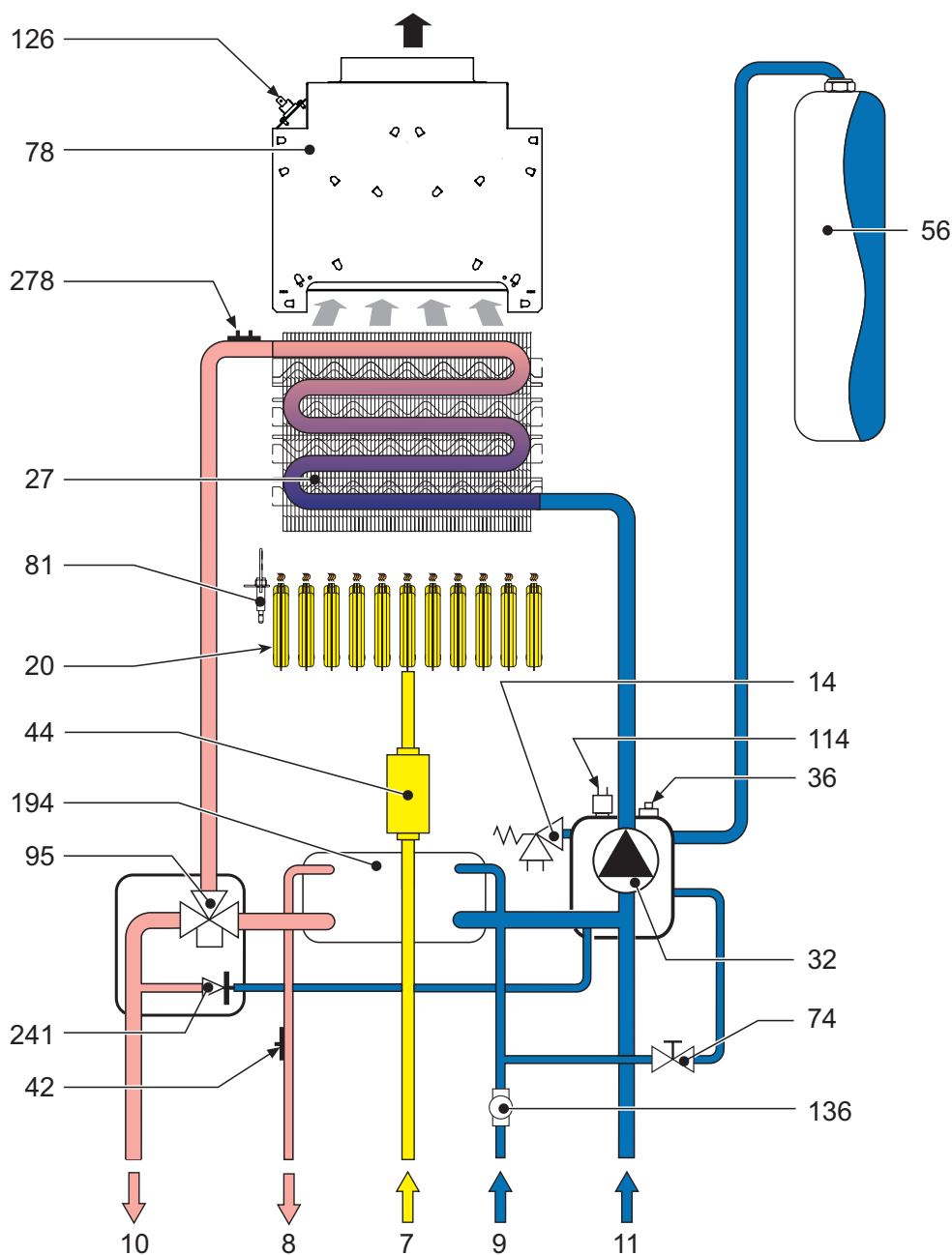
fig. 24 - Circuito idraulico
