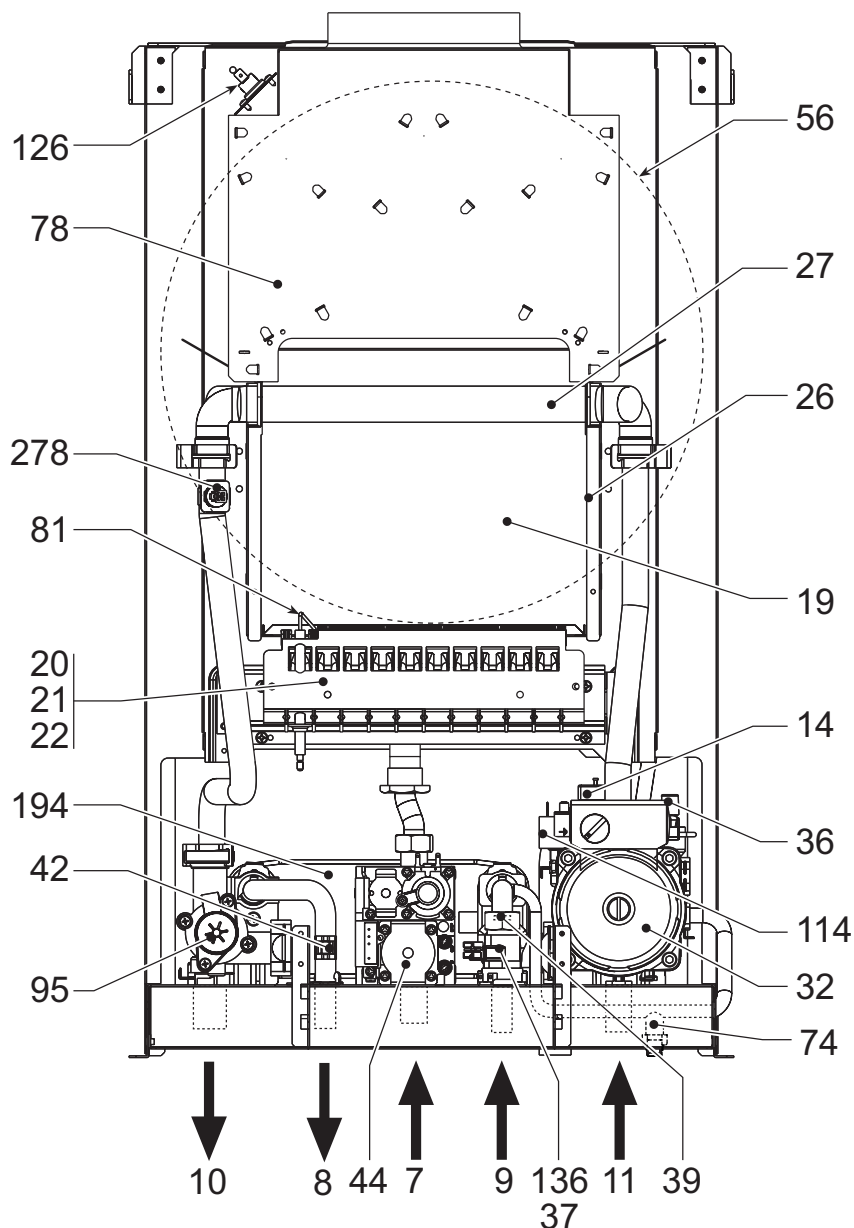
fig. 23 - Vedere generală
