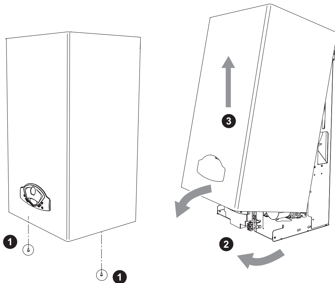
рис. 21 - Демонтаж кожуха
