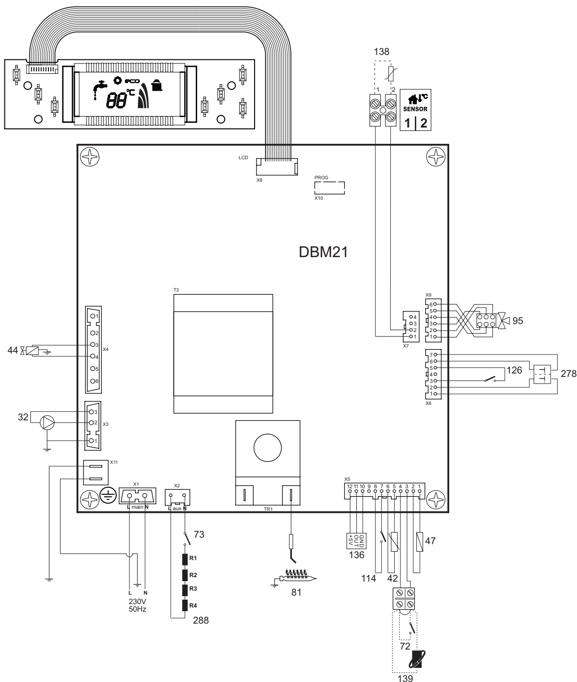
fig. 25 - Wiring diagram
