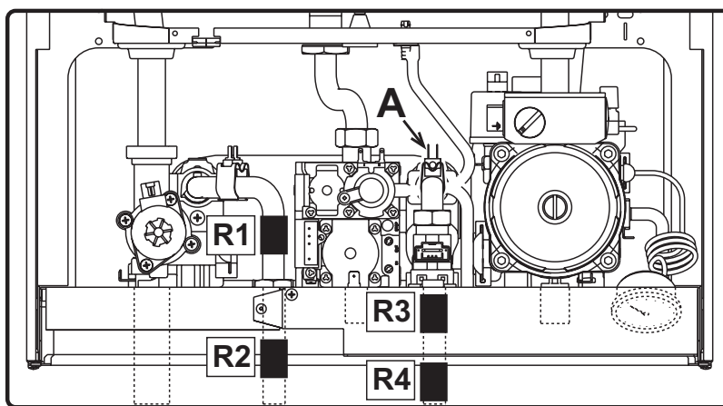
рис. 17 - Размещение нагревателей и морозозащитного термостата
