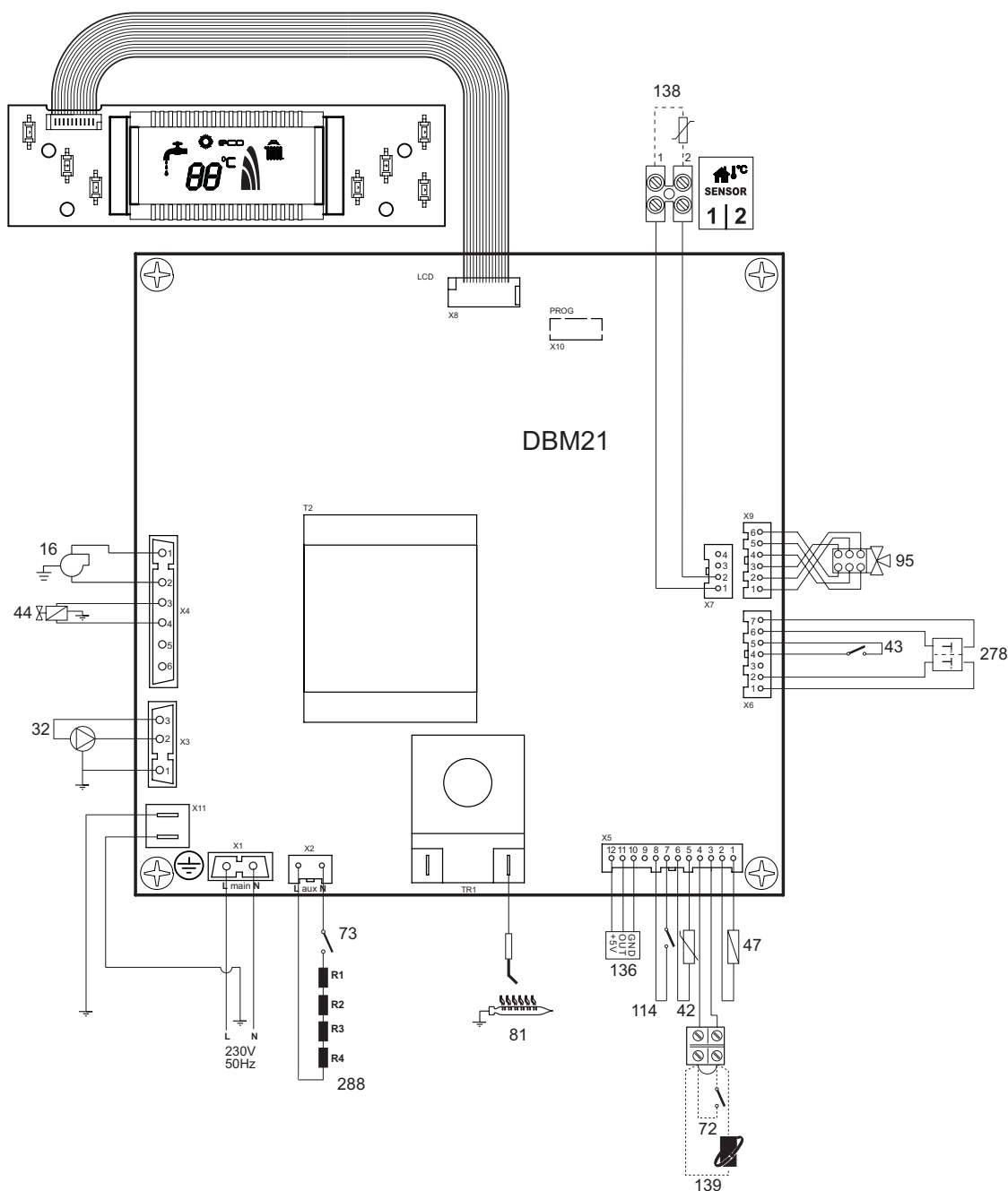
рис. 29 - Электрическая схема
