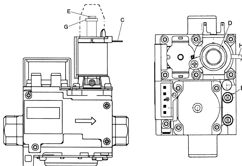
рис. 23 - Газовый клапан
