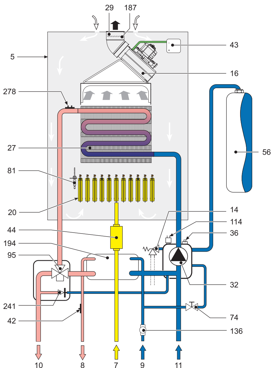
fig. 28 - Circuito idraulico
