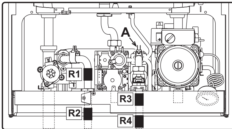
fig. 17 - Poziționarea încălzitoarelor și a termostatului antiîngheț
