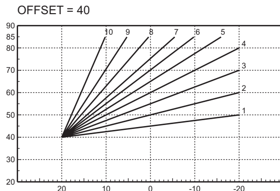
рис. 14 - Пример параллельного смещения компенсационных характеристик
