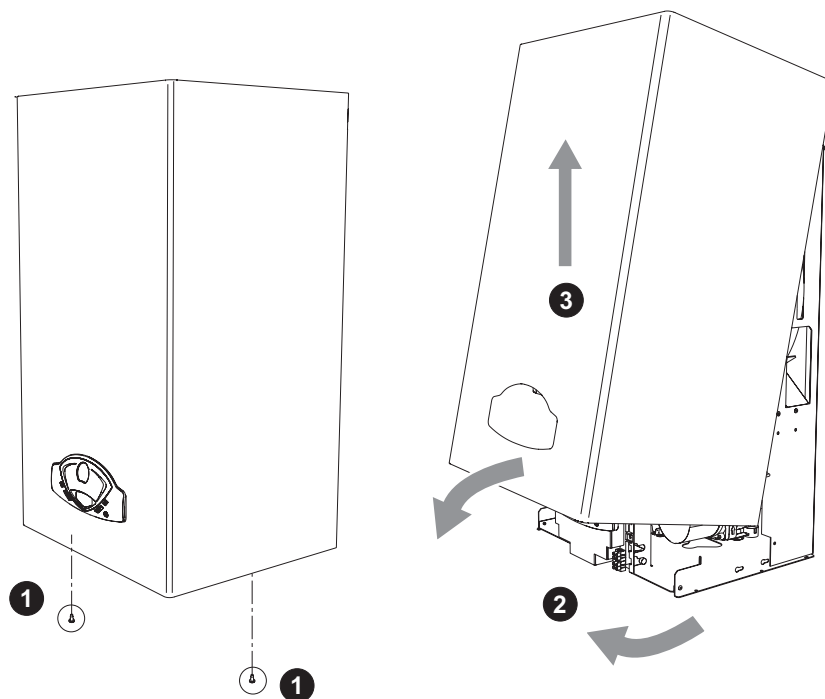
fig. 24 - Deschiderea carcasei
