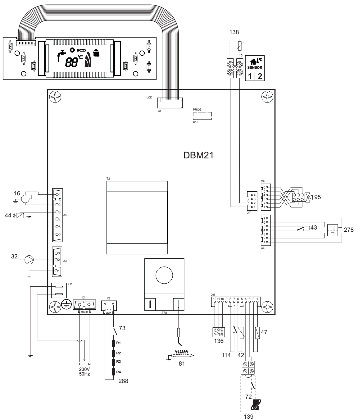
fig. 29 - Schemă electrică
