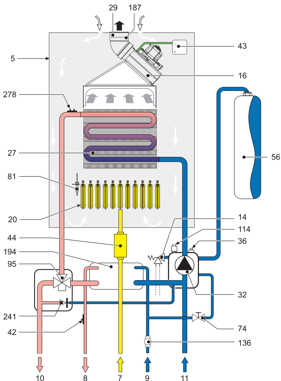
fig. 28 - Circuitul hidraulic
