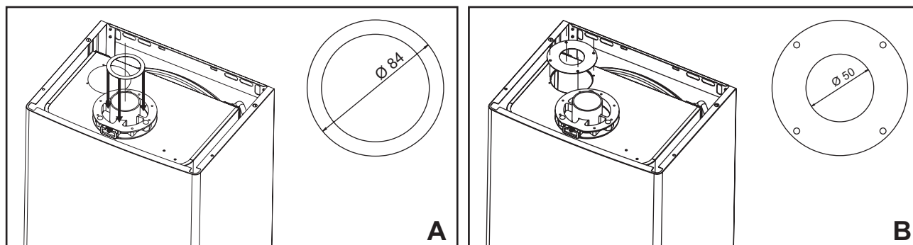
fig. 19 - Înlocuirea diafragmei
