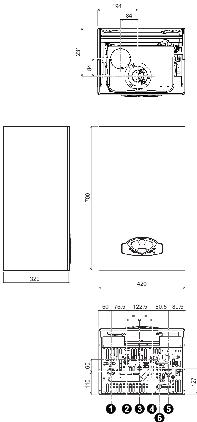
fig. 26 - Dimensiuni și racorduri
