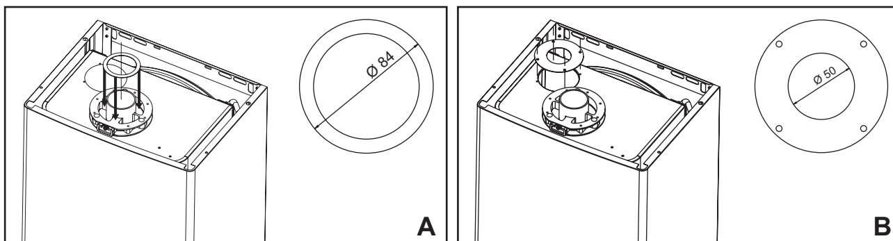
рис. 19 - Замена диафрагмы
