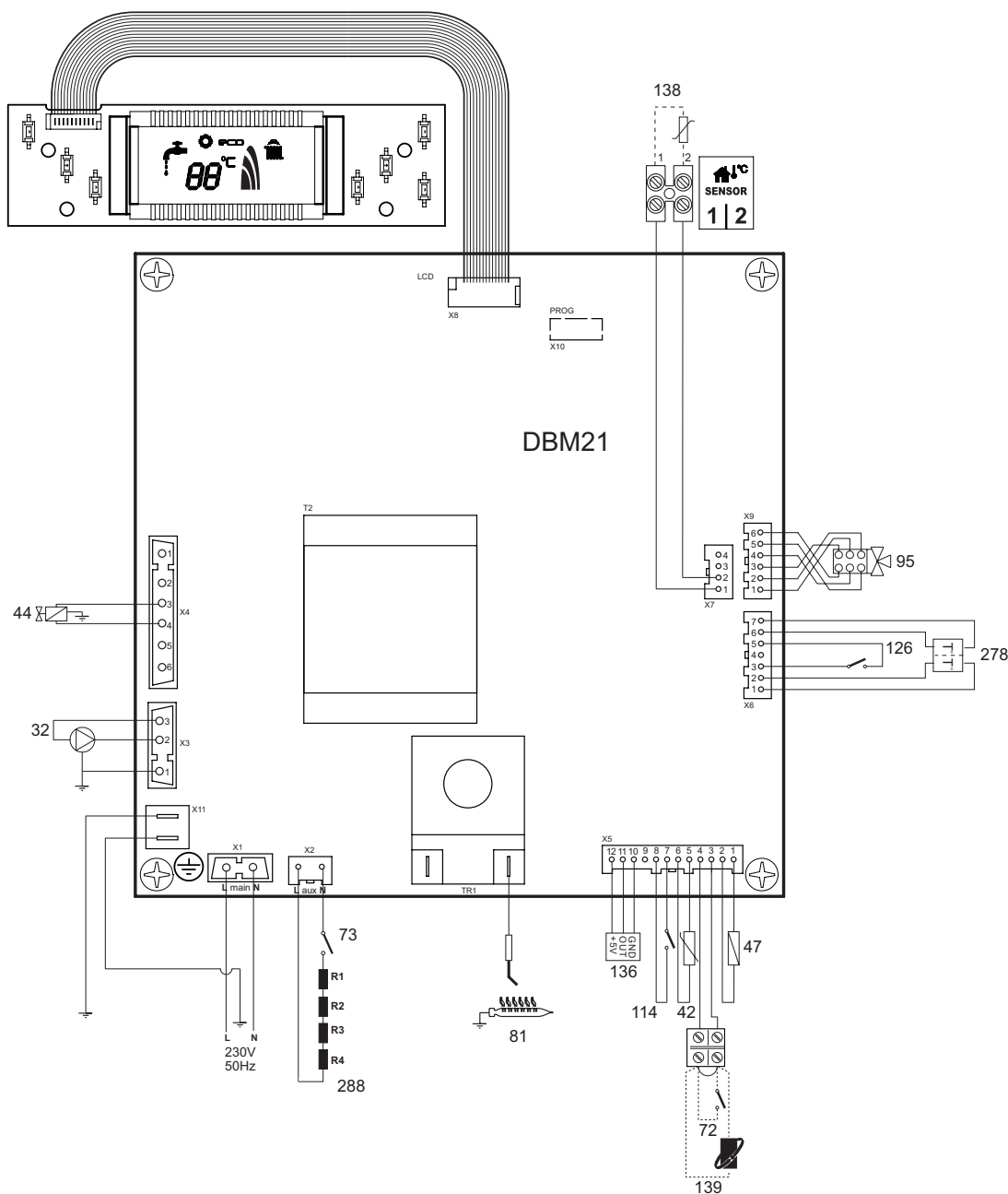
fig. 25 - Schema elettrico
