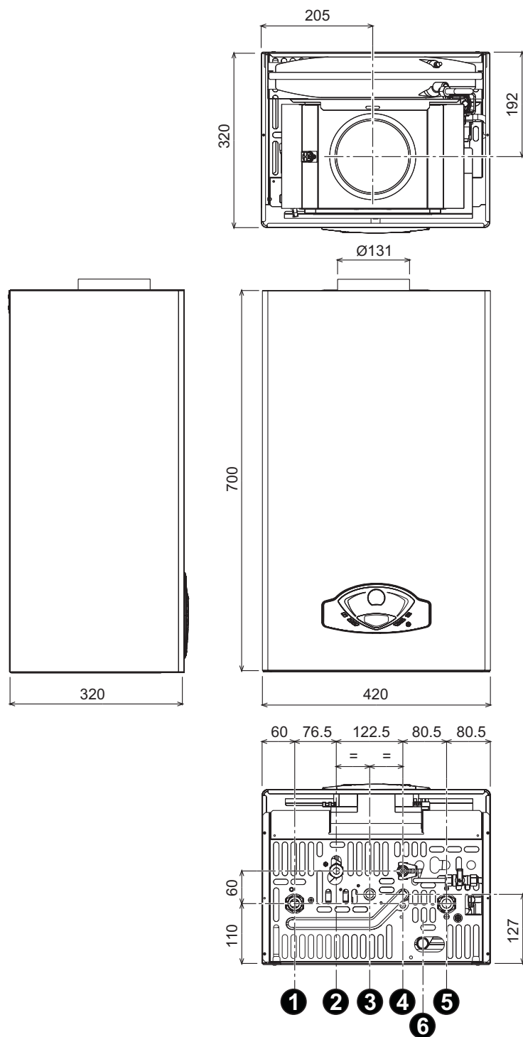
fig. 22 - Dimensioni e attacchi
