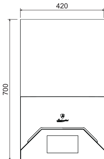
fig. 35 - Vista frontale
