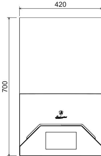
fig. 35- Vista frontal
