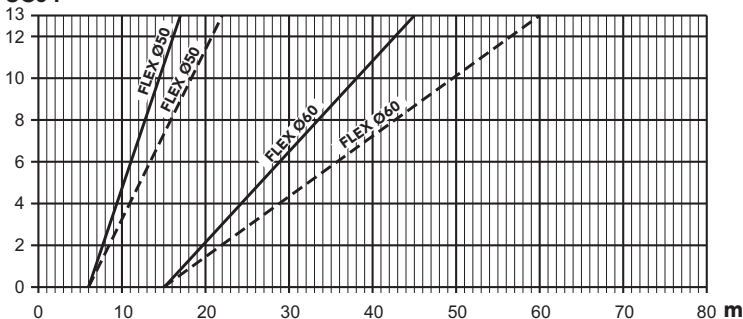
fig. 19- Grafic pentru alegerea parametrului pentru horn
