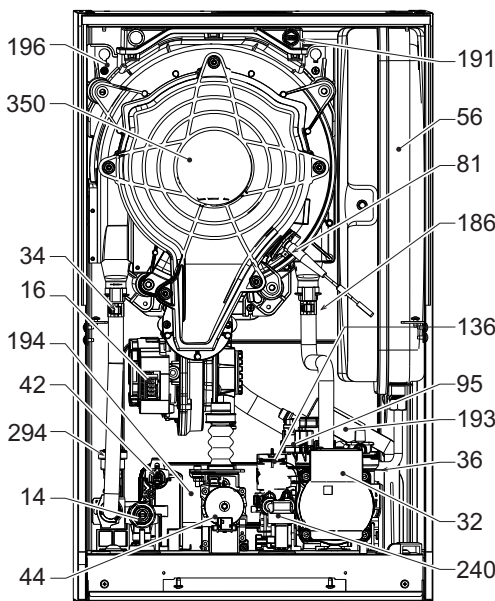
fig. 42 - Vista generale
