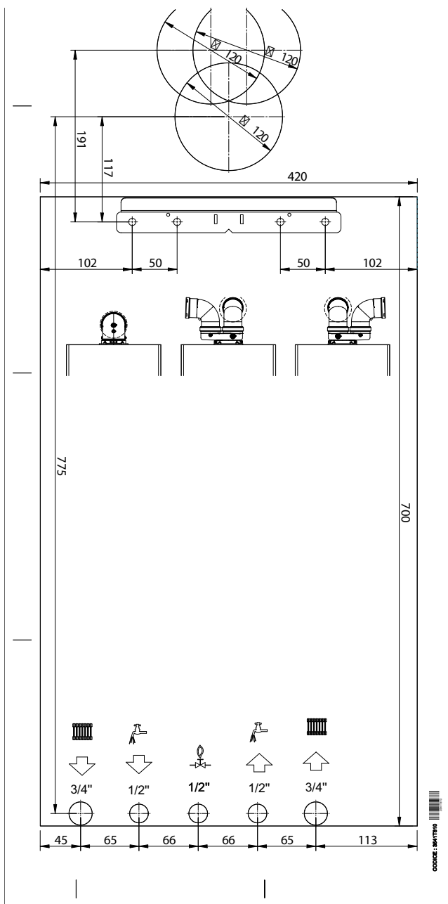
fig. 41 - Dima in carta
