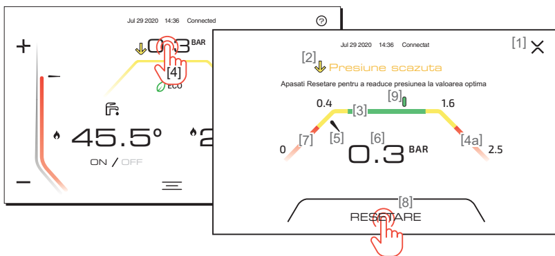
fig. 8 - Controllo pressione
