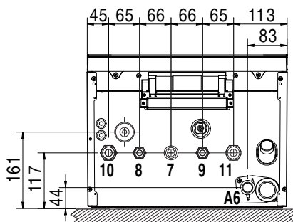
fig. 38 - Vista dal basso
