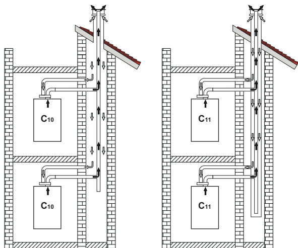
fig. 21- Exemple de racordare sistemul C10 și C11 (→ = Aer / → = Gaze arse)
