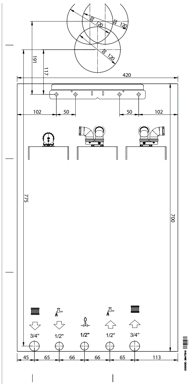
fig. 41- Plantilla de papel
