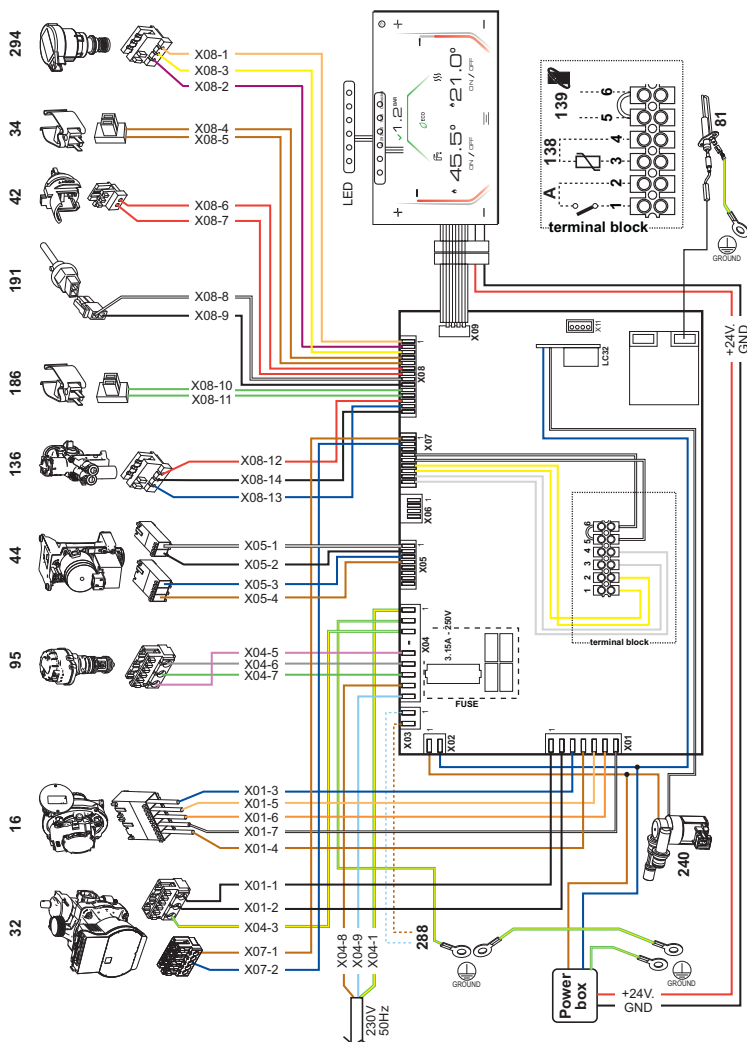
fig. 46- Esquema eléctrico
