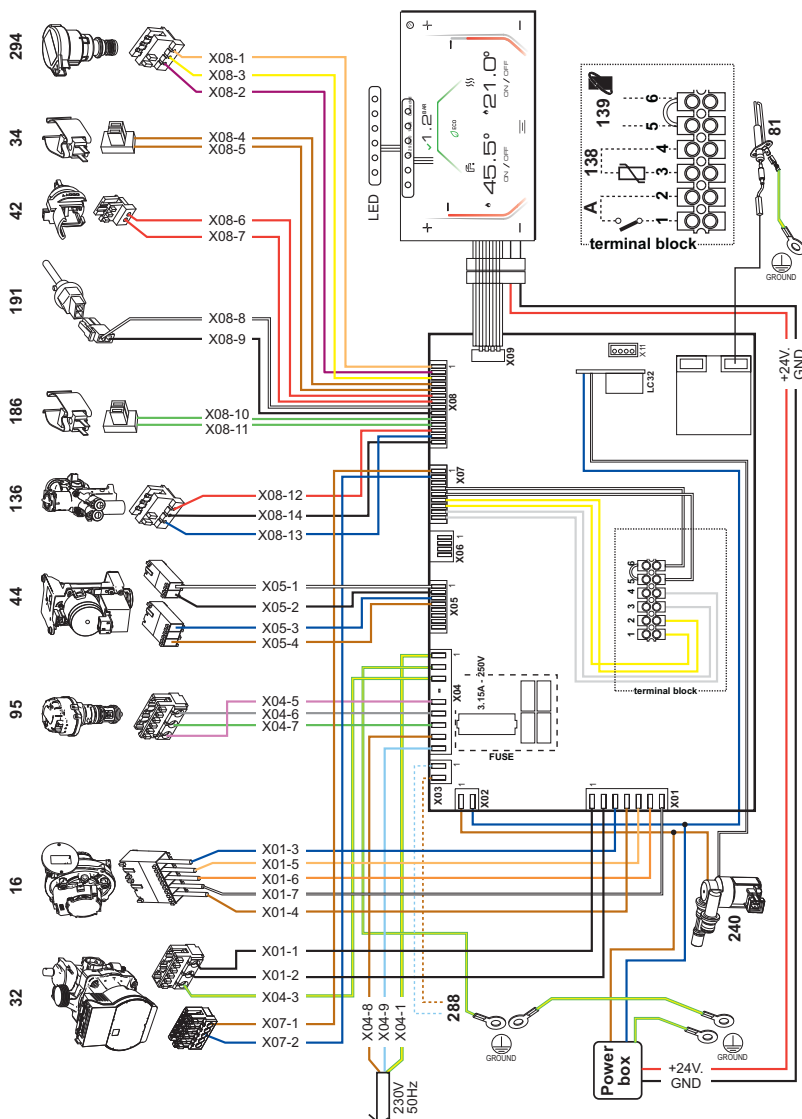
fig. 46- Wiring diagram
