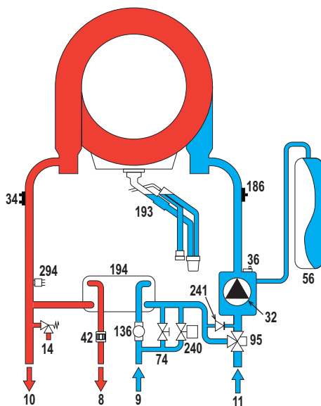
fig. 43- Circuitul hidraulic
