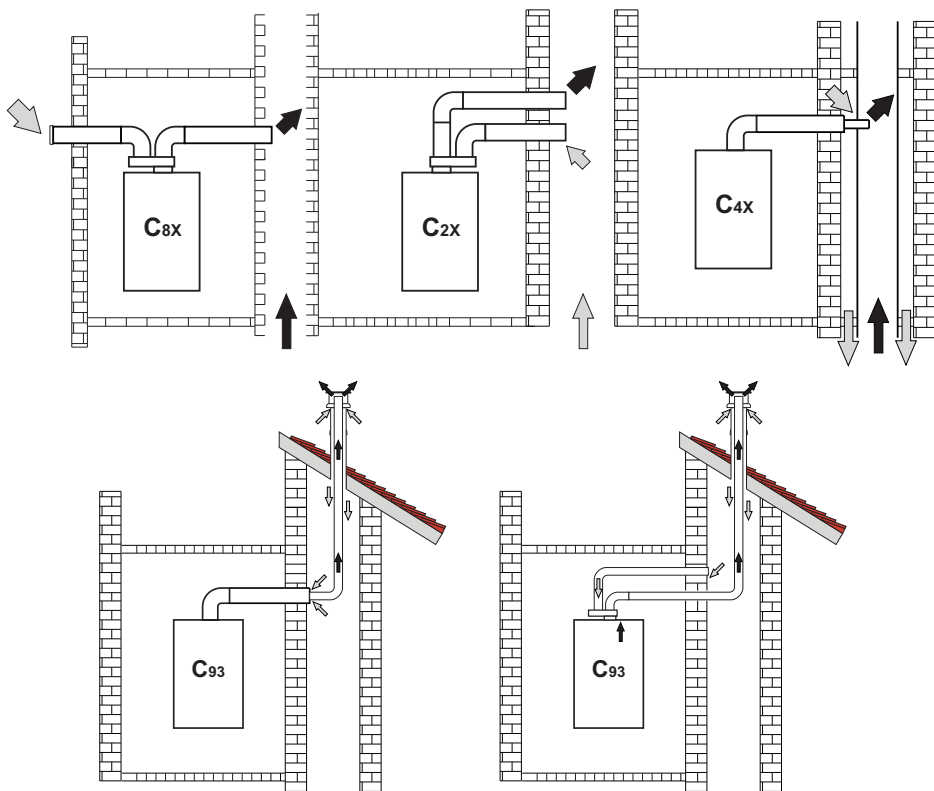
fig. 20- Ejemplos de conexión a chimeneas (⇐ = aire / ➡ = humos)
