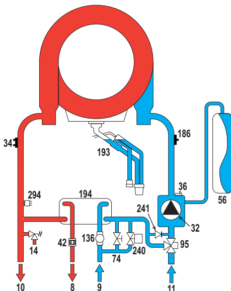
fig. 43 - Circuito idraulico
