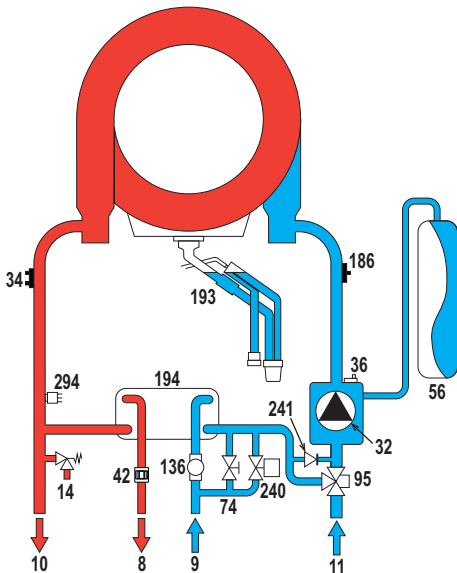
fig. 43- Circuito hidráulico
