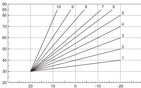
fig. 25 - Curve di compensazione
