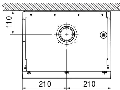
fig. 37 - Vista dall'alto
