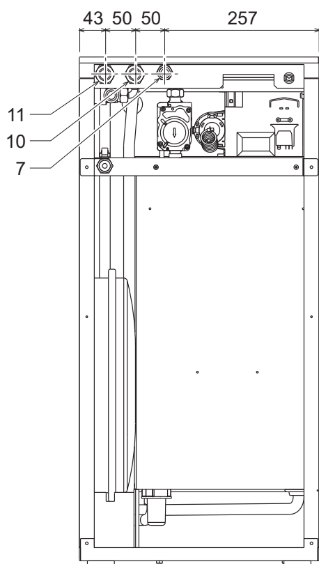
fig. 28 - Vista posteriore
