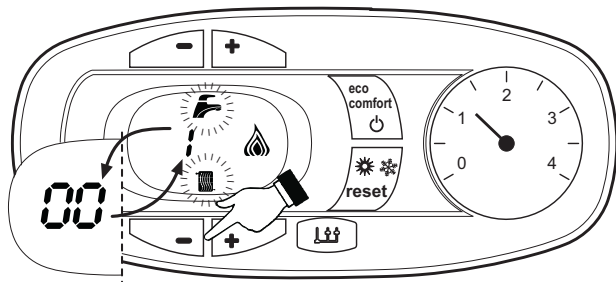
рис. 24 Режим TEST (мощность системы отопления = 100%)
