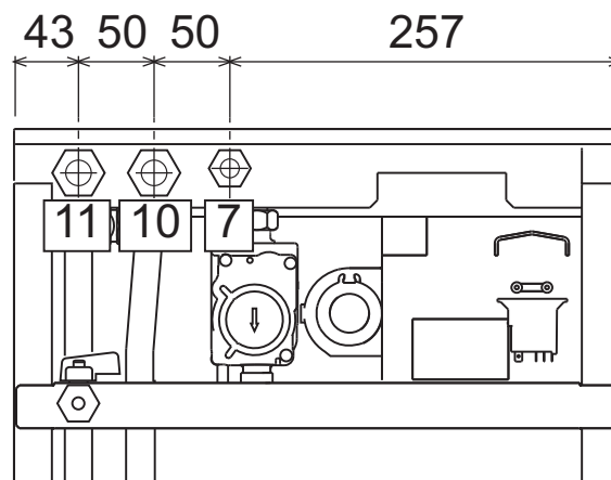
рис. 13 - Гидравлические штуцеры
