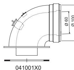
fig. 17 - Accessori di partenza per condotti coassiali
