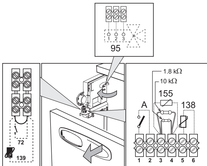
fig. 15 - Accesso alla morsettiera
