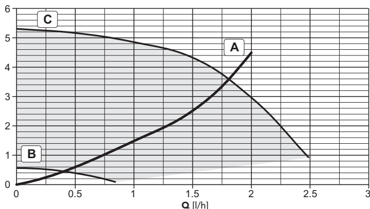
рис. 31 - Потеря напора/Напор циркуляционных насосов iXinox B 35
