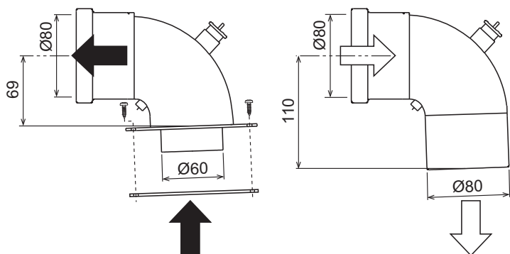
рис. 19 - Соединительный элемент для раздельных труб
