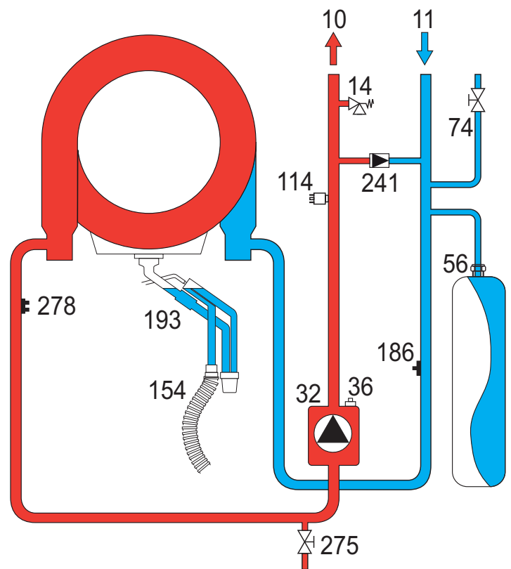
рис. 30 - Гидравлический контур
