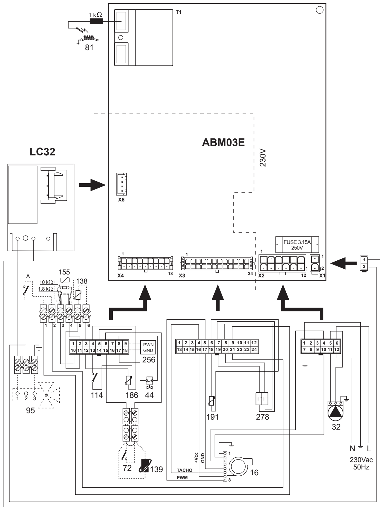
рис. 32 - Электрическая схема
