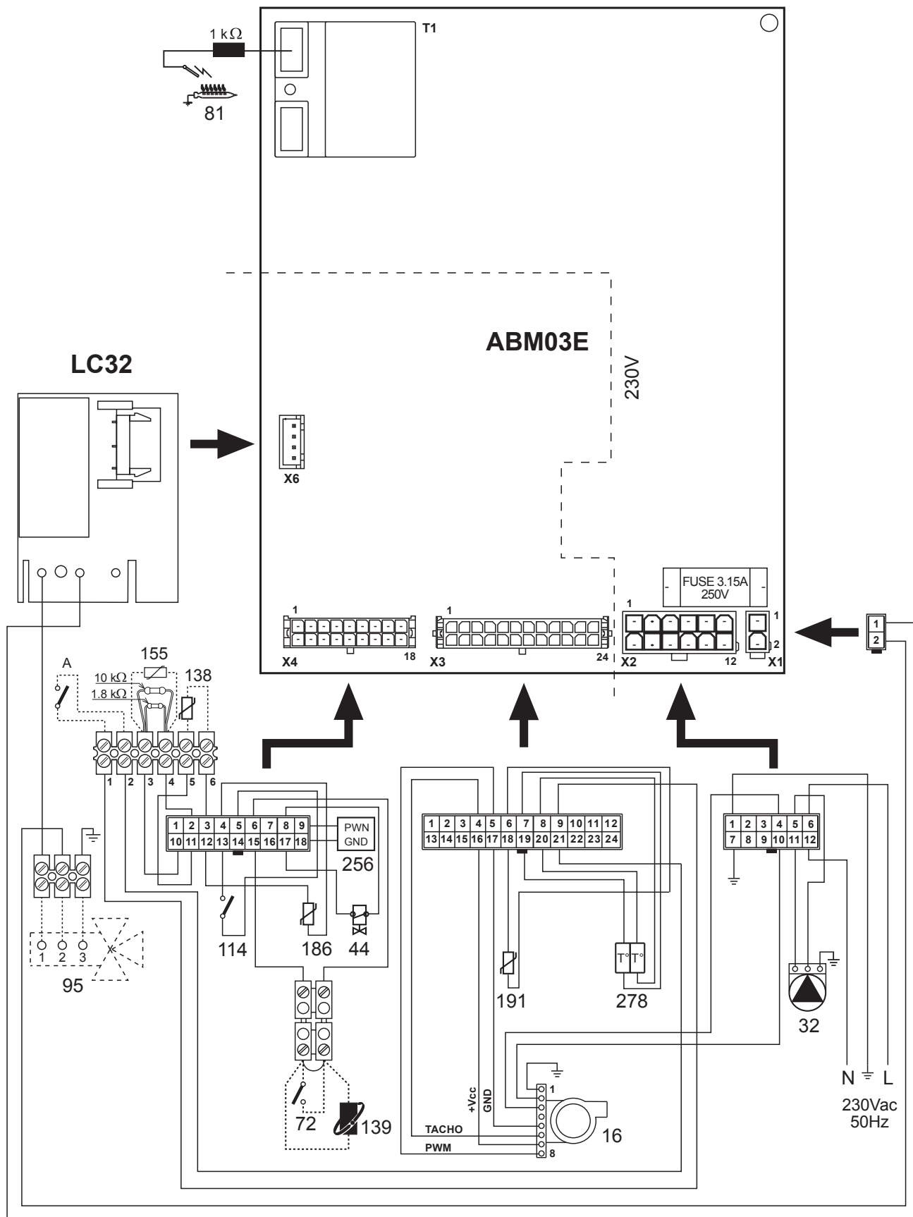
fig. 32 - Schema elettrico
