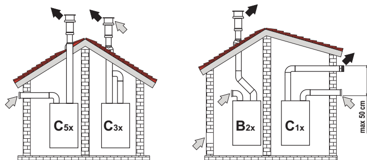
рис. 18 - Примеры подсоединения с помощью раздельных труб (⇨ = Воздух / ⇨ = дымовые газы)
