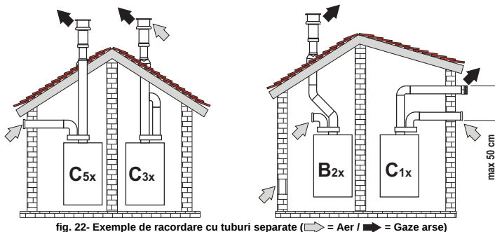
fig. 22- Exemple de racordare cu tuburi separate (⇨ = Aer / ⇨ = Gaze arse)
