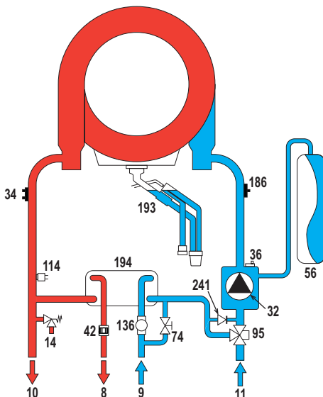
wygląd 41- Obieg wody
