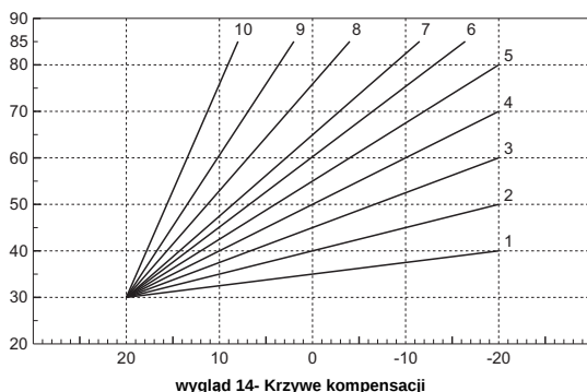
wygląd 14- Krzywe kompensacji
