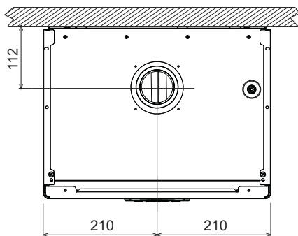
εικ. 38- Κάτωψη
