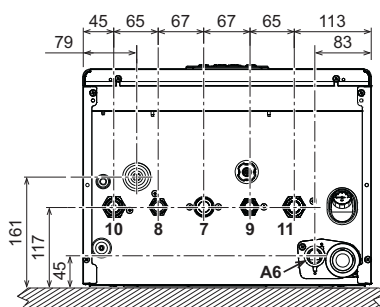
fig. 39 - Vista dal basso
