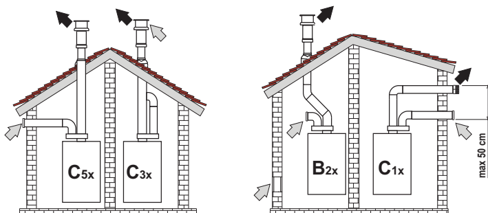
рис. 22- Примеры подсоединения с помощью раздельных труб (⇨ = Воздух/ ⇨ = Дымовые газы)
