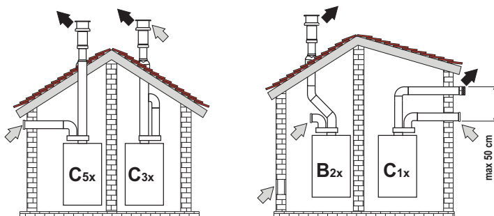
εικ. 22- Παραδείγματα σύνδεσης με ξεχωριστούς σωλήνες (⇨ = Αέρας / ⇨ = Καυσάεριο)
