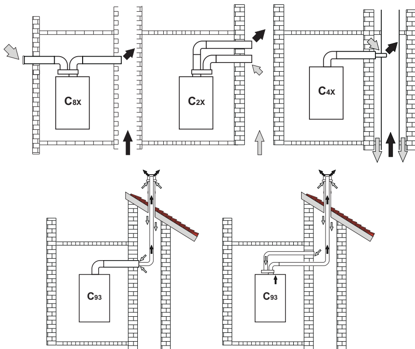
εικ. 26 Παραδείγματα σύνδεσης σε καπνοδόχους (↗ = Αέρας / ↘ = Καυσάερια)
