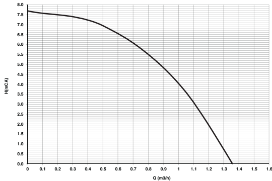
рис. 44- Остаточный напор, достигаемый в системе
