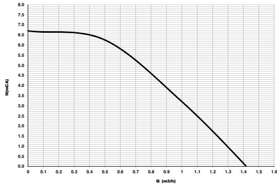
рис. 43- Остаточный напор, достигаемый в системе
