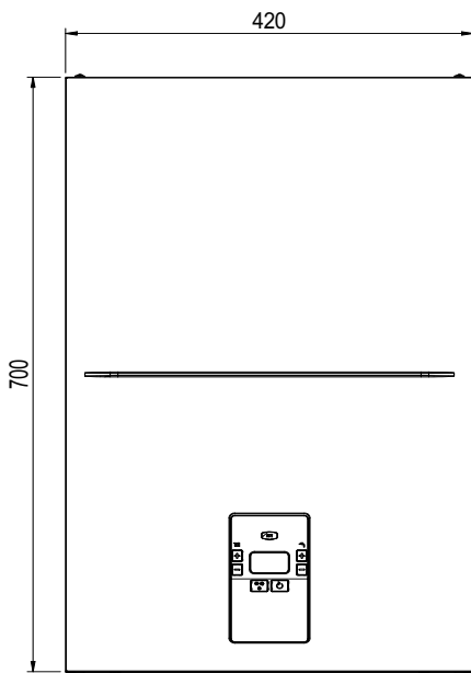
рис. 32- Вид спереди
