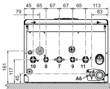
рис. 39- Вид снизу
