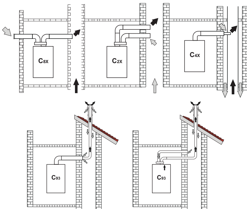
рис. 26- Примеры подсоединения к дымоходам (⇐ = Воздух / ➡ = Дымовые газы)
