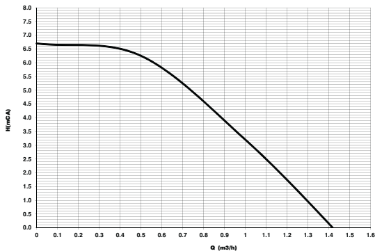
fig. 42- Carga hidrostática residual disponible en la instalación
