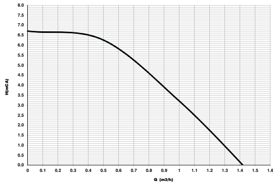
fig. 42 - Prevalenza residua disponibile all'impianto
