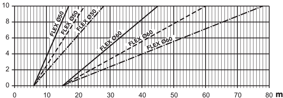
wygląd 25- Wykres wyboru parametrów przewodu spalinowego
