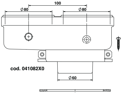
wygląd 23- Człon początkowy do montażu oddzielnych przewodów
