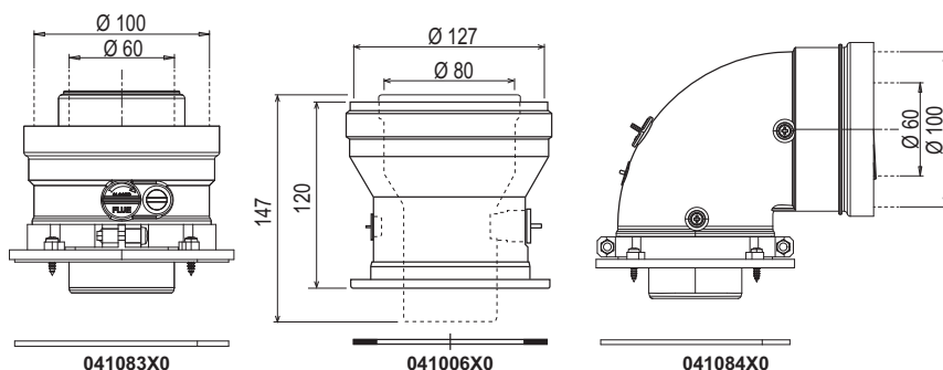
fig. 21 - Accessori di partenza per condotti coassiali
