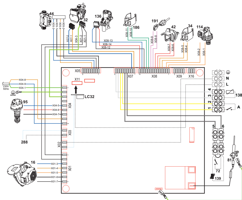
fig. 45- Esquema eléctrico
