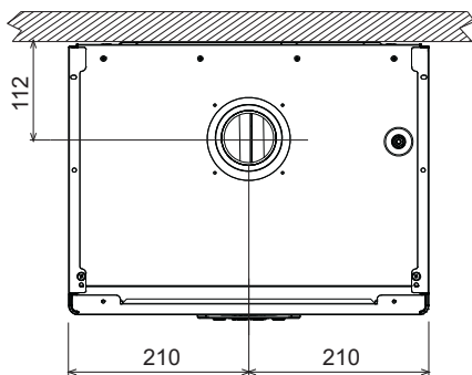
fig. 38 - Vista dall'alto
