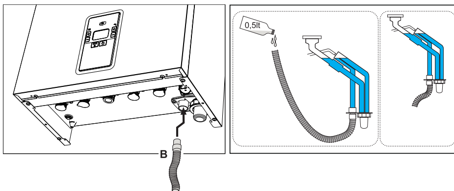
рис. 28- Подсоединение трубы для слива конденсата
