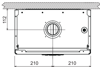
рис. 34- Вид сверху
