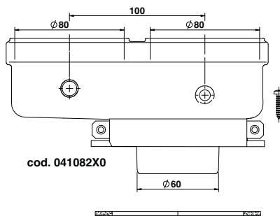
рис. 23- Исходная принадлежность для раздельных труб
