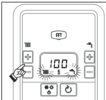
εικ. 29- Λειτουργία ΕΛΕΓΧΟΥ (ισχύς θέρμανσης = 100%)
