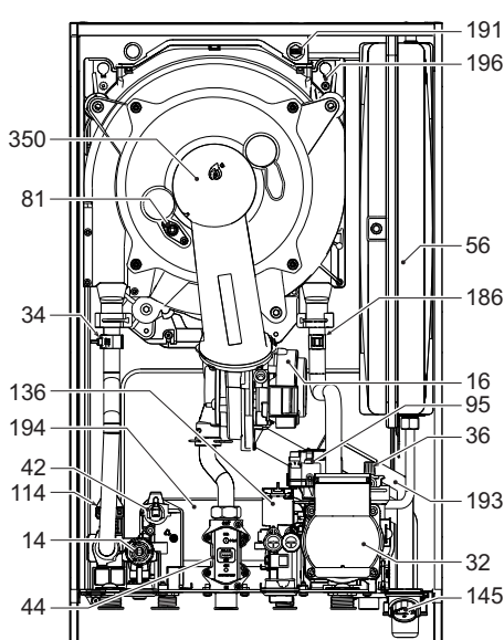
рис. 40- Общий вид
