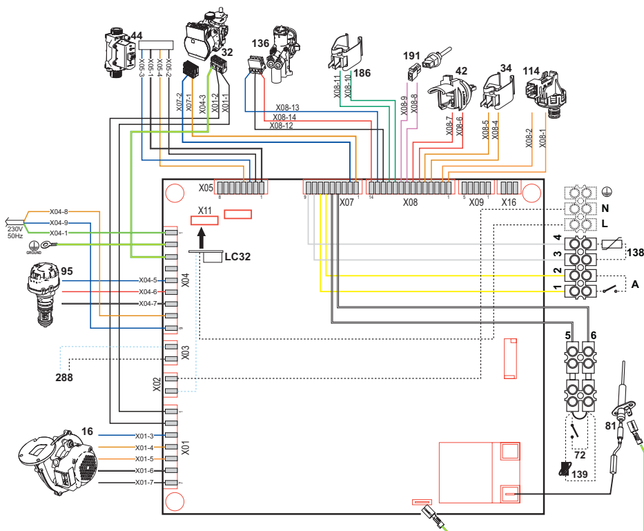
fig. 45- Schemă electrică
