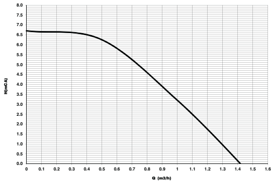
fig. 43- Carga hidrostática residual disponible en la instalación
