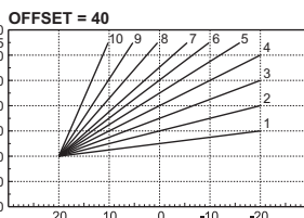
fig. 15- Exemplet de deplasare paralelă a curbelor de compensare
