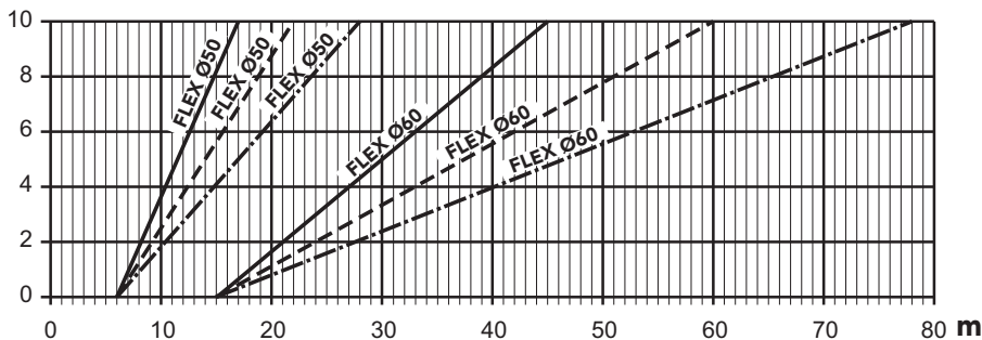
рис. 25- График выбора параметров дымохода
