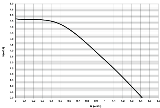
εικ. 43- Διαθέσιμο υπολειπόμενο μανομετρικό ύψος στην εγκατάσταση
