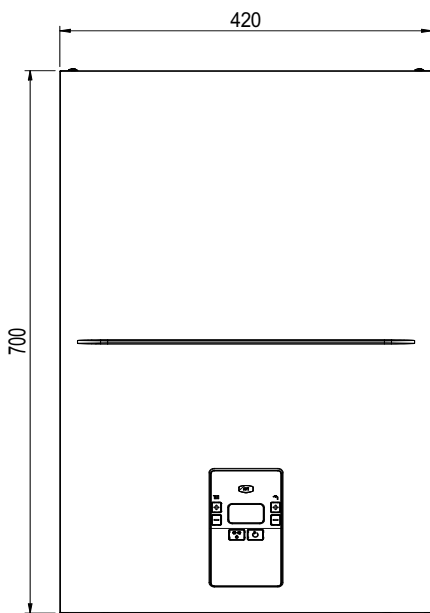
fig. 36 - Vista frontale
