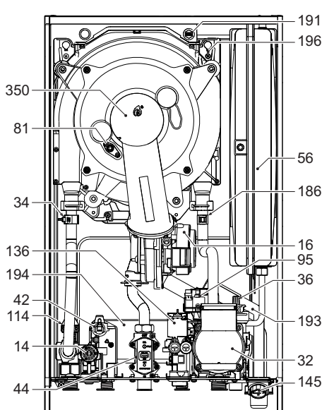
wygląd 40- Widok ogólny
