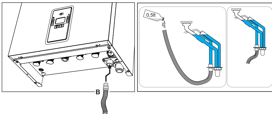
fig. 28- Racordarea evacuării condensului
