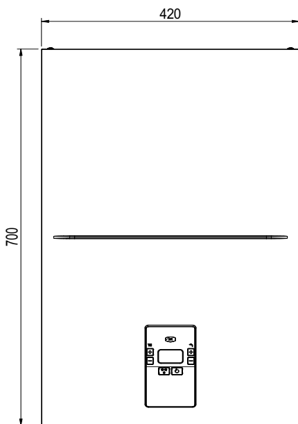
fig. 36- Vedere frontală
