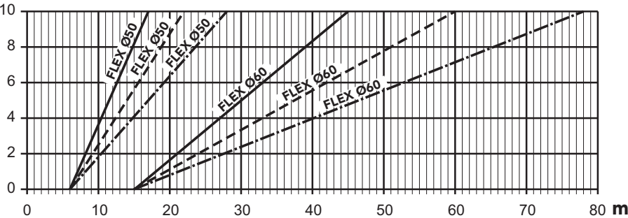
fig. 25- Chart for flue parameter choice
