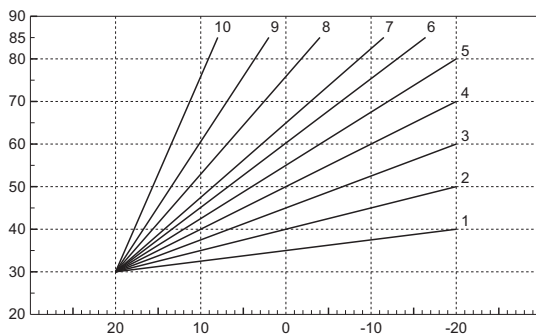
рис. 14- Компенсационные кривые
