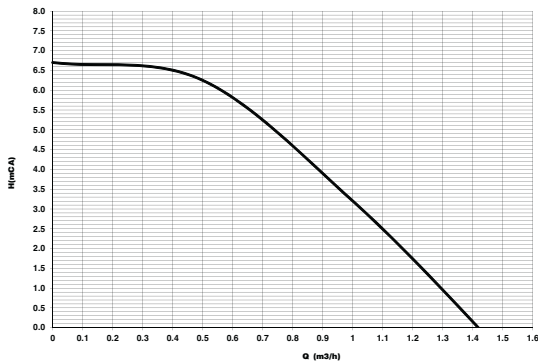
εικ. 42- Διαθέσιμο υπολειπόμενο μανομετρικό ύψος στην εγκατάσταση
