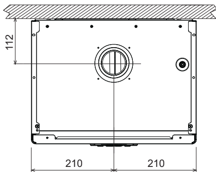
рис. 38- Вид сверху
