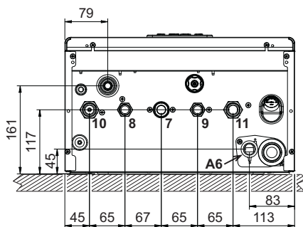
рис. 35- Вид снизу
