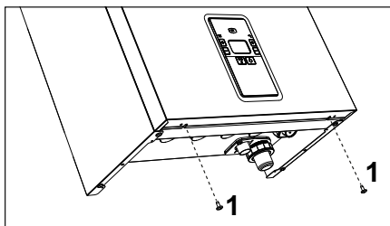
wygląd 30- Otwieranie panelu przedniego
