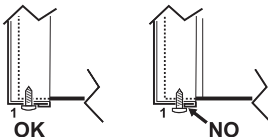
fig. 31 - Posizione corretta pannello frontale
