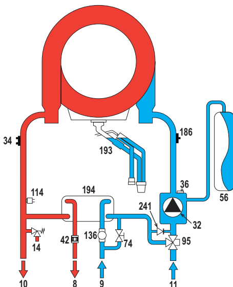
рис. 41- Гидравлический контур
