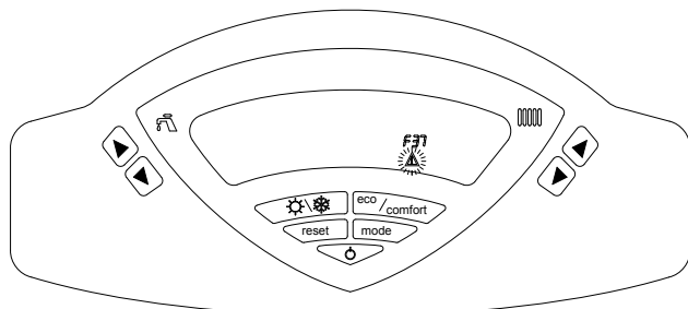
Fig.16 - Anomalia pressione impianto insufficiente
