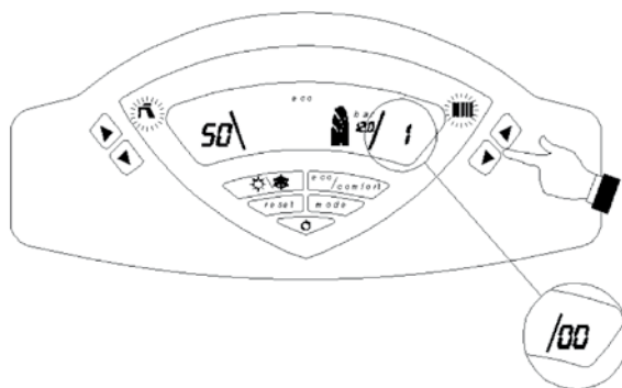
Modalità TEST (potenza riscaldamento 100%)
