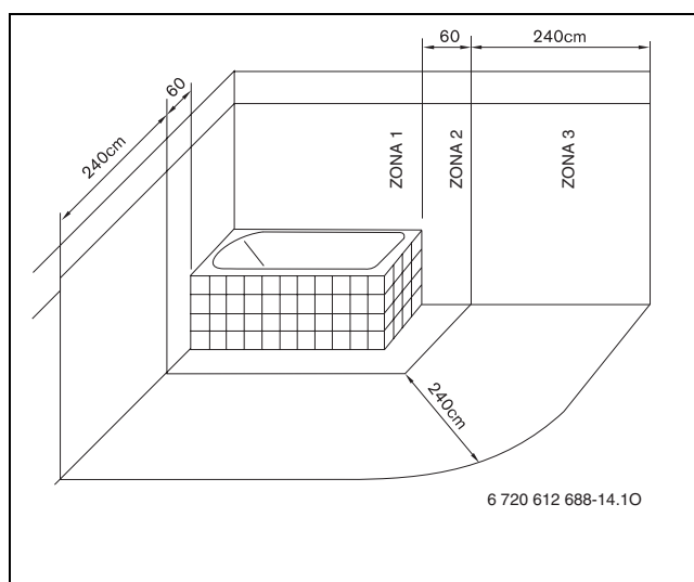
Fig. 16 Rappresentazione della Zona 3 (CEI 64-8)
