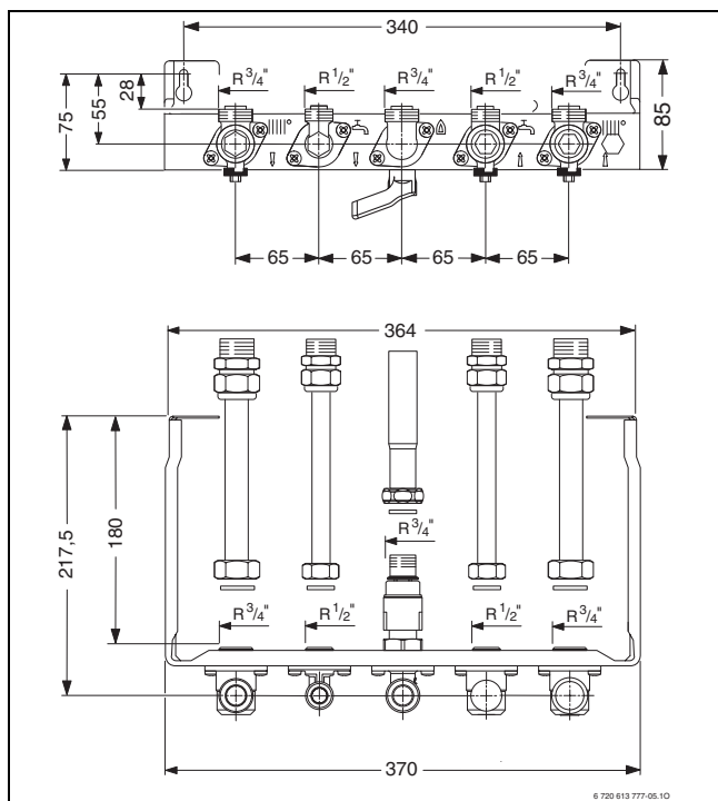
Fig. 7 Tubazioni a vista, realizzate in rame con brasatura placca rubinetteria DOS GA 5/18
