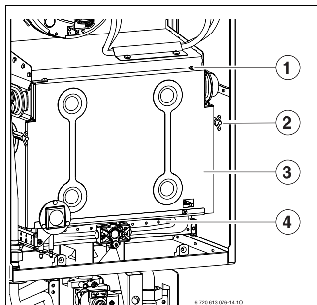
Fig. 37 Aprire il bruciatore
