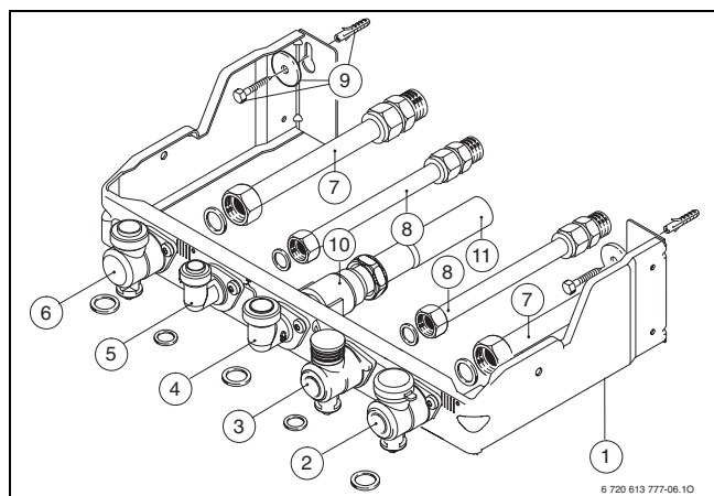
Fig. 9 Piastra d'installazione, accessorio DOS GA 5/18
