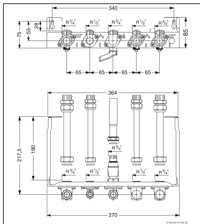
Fig. 8 Tubazioni a vista, realizzate in rame con brasatura piastra d'installazione accessorio DOS GA 5/18
