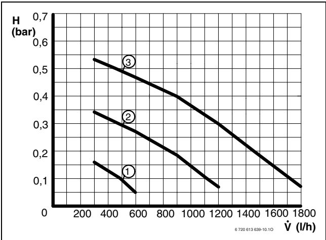
Fig. 29 La pompa curva
