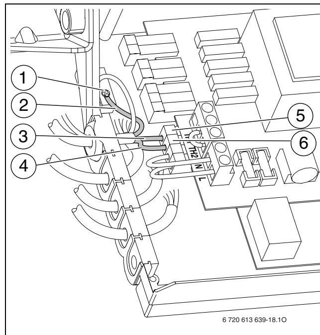
Fig. 19 Il collegamento di cavo principale 230 V AC
