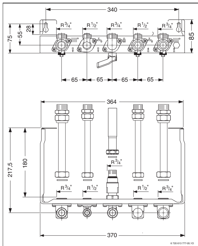
Fig. 9 Tubazioni a vista, realizzate in rame con brasatura placca rubinetteria, acc. DOS GA 5/18
