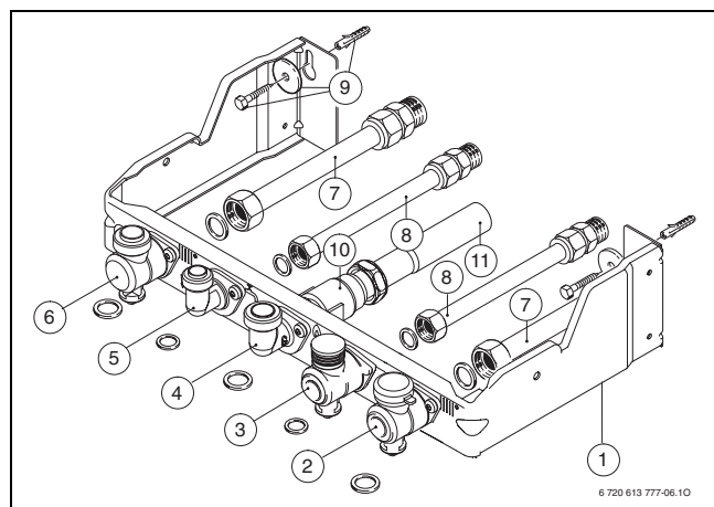
Fig. 10 Placca rubinetteria, accessorio DOS GA 5/18
