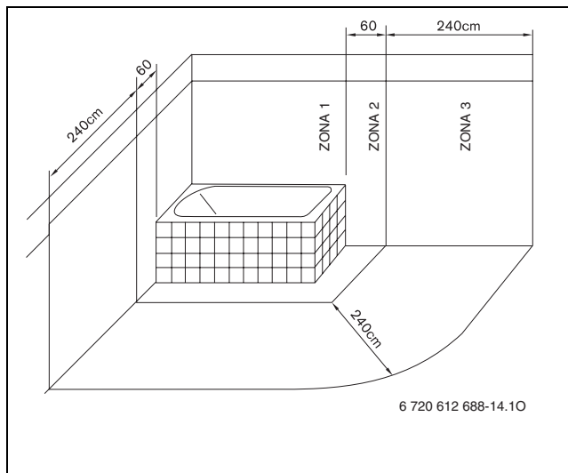
Fig. 20 Rappresentazione della Zona 3 (CEI 64-8)
