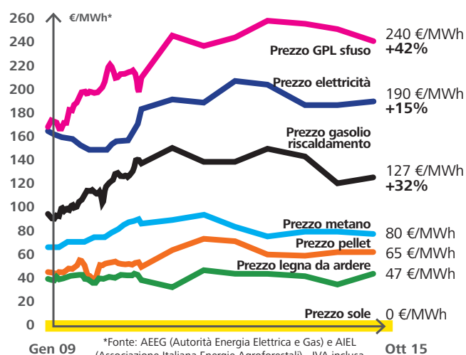
Andamento prezzi energia, 2009-2015* Costo combustibili a parità di energia prodotta
