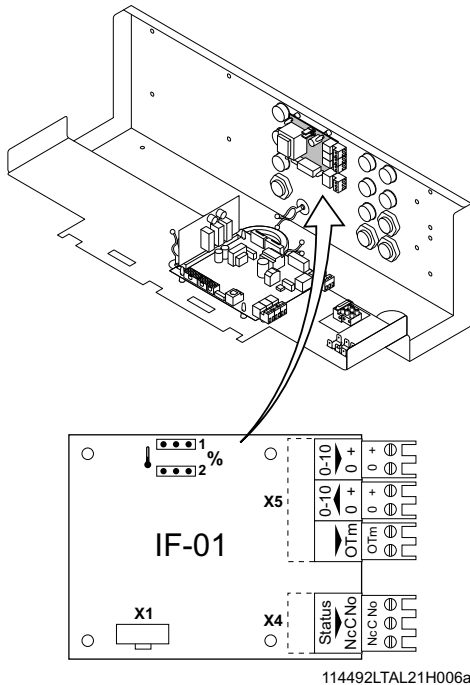
fig. 12 Scheda di gestione opzionale da 0 - 10 V (IF-01)
