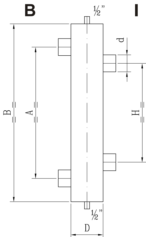
fig. 37 Figura del separatore idraulico
