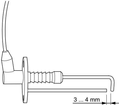
fig. 31 Controllo dell'elettrodo di accensione
