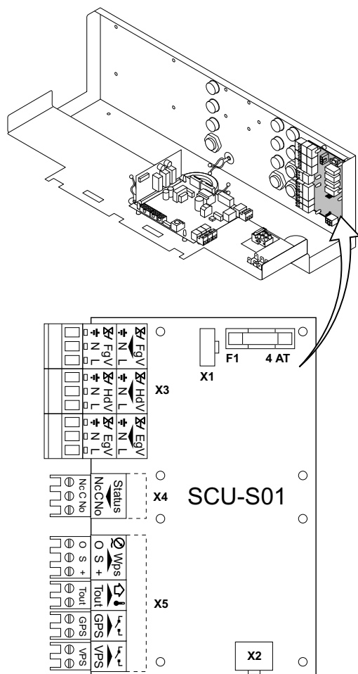
fig. 15 Scheda ampliamento di gestione/ protezione opzionale (SCU-S01).
