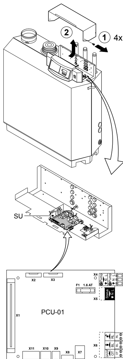
fig. 10 Scheda di gestione standard (PCU-01)
