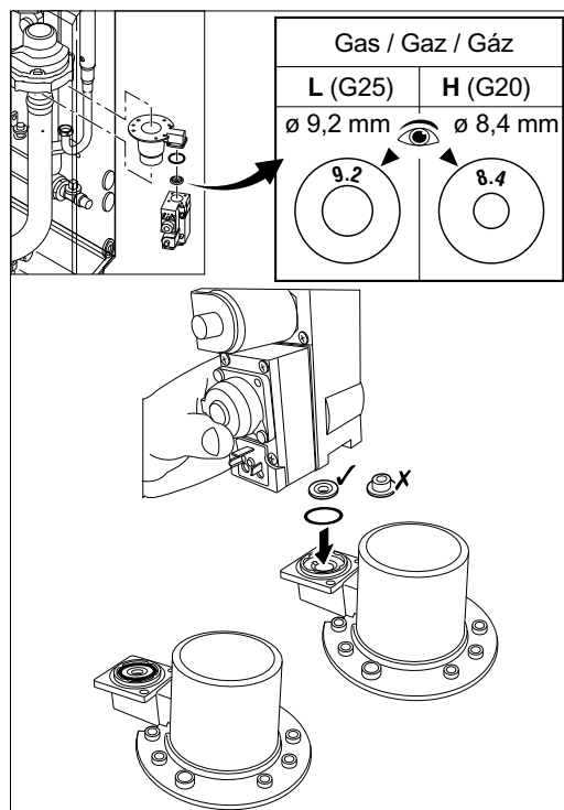
fig. 26 Controllare le dimensioni e la posizione del limitatore
