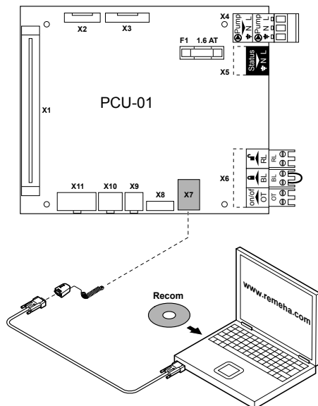
fig. 11 Allacciamento PC
