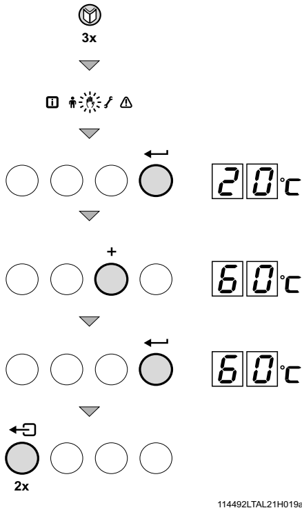
fig. 22 Impostazione della modalità di funzionamento manuale
