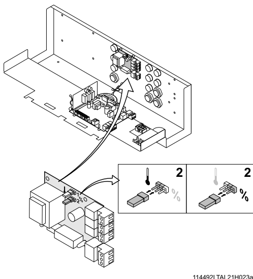
fig. 13 Ponticello 2: posizione a sinistra per la regolazione della temperatura; posizione di destra per la potenza.
