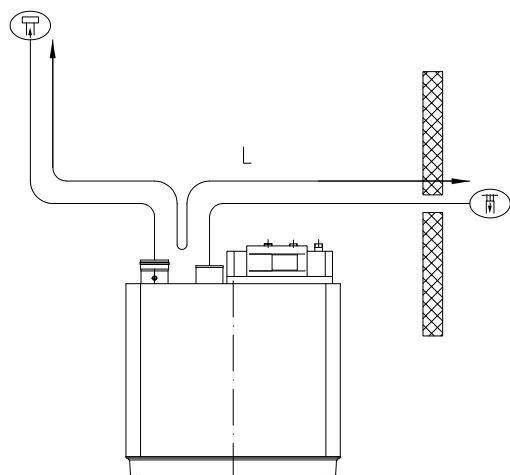
fig. 08 Uscita in varie zone di pressione
