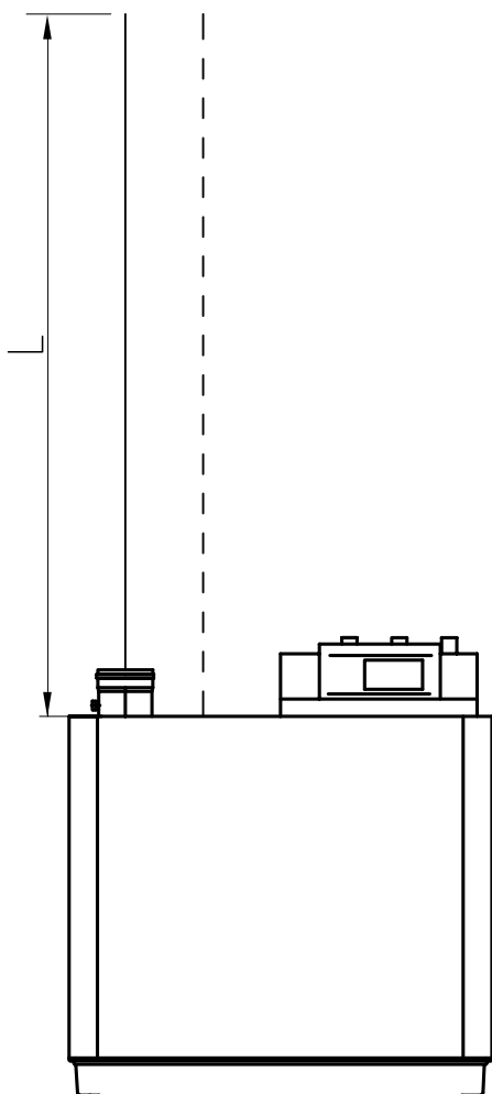
fig. 06 Versione stagna
