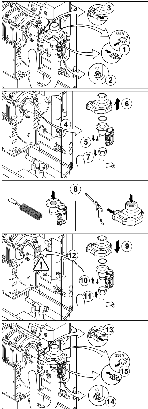
fig. 27 Pulizia della ventola ModuPower 210-113
