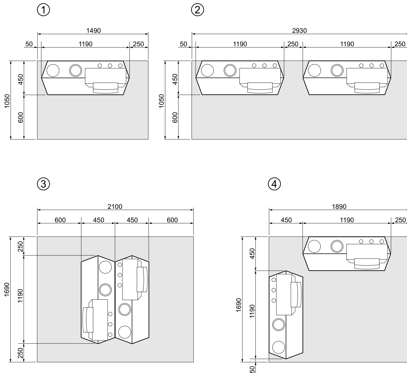
fig. 02 Possibilità di ubicazione
