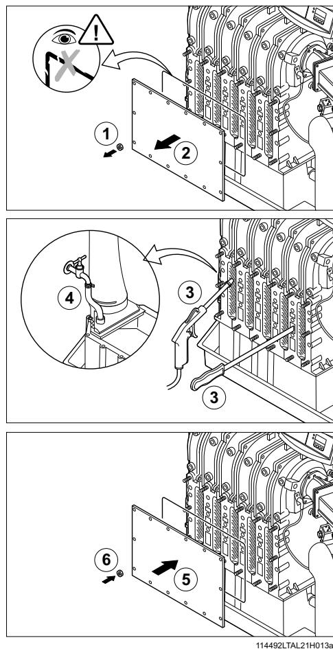
fig. 29 Pulizia dello scambiatore
