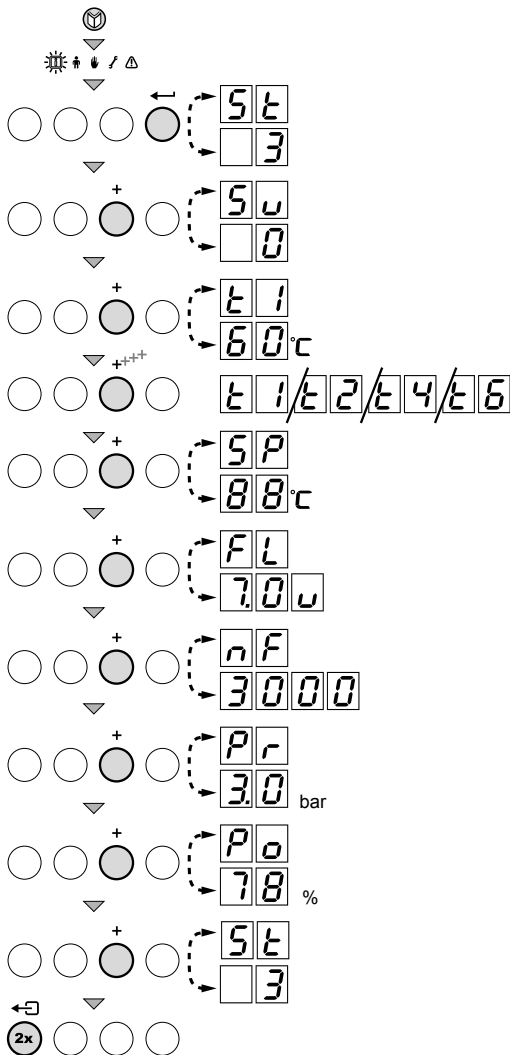
fig. 18 Lettura dei valori attuali
