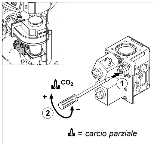
fig. 24 Regolazione CO 2 carico parziale ModuPower 210-160 e 200
