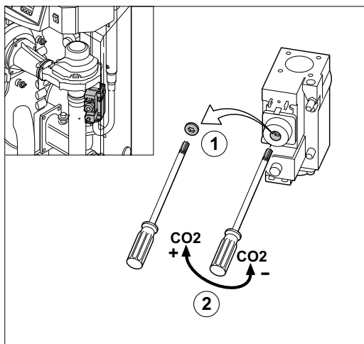
fig. 25 Regolazione CO 2 carico parziale ModuPower 210-113
