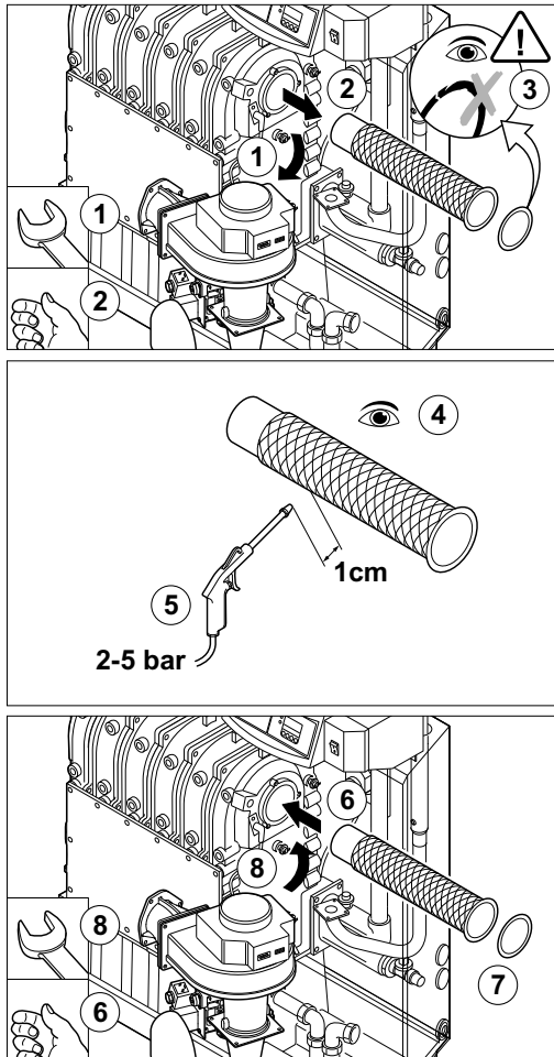
fig. 30 Pulizia del bruciatore
