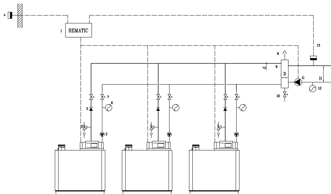
fig. 36 Esempio di schema idraulico di installazione a cascata
