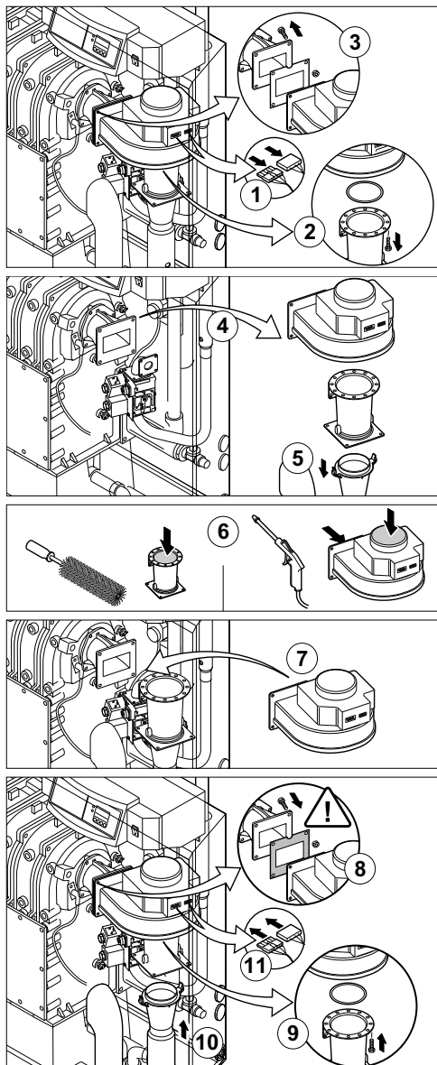
fig. 28 Pulizia della ventola ModuPower 210-160 e ModuPower 210-200:
