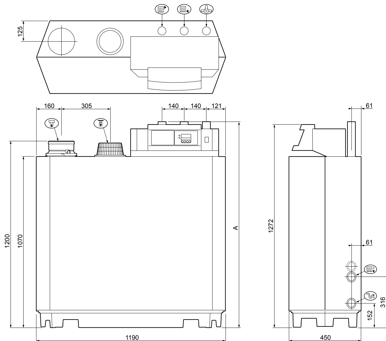
fig. 01 Dimensioni
