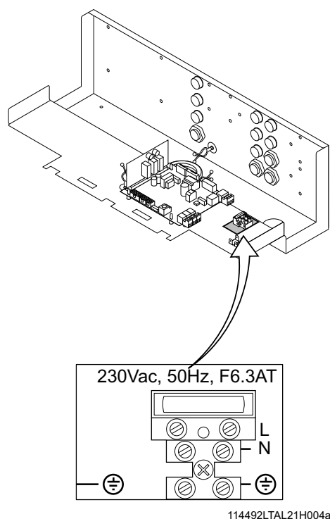
fig. 09 Collegare il cavo di rete
