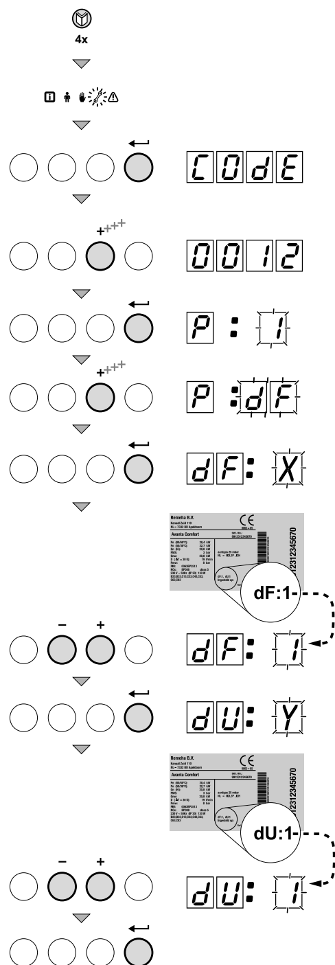
fig. 21 Ripristino dell'impostazione di fabbrica
