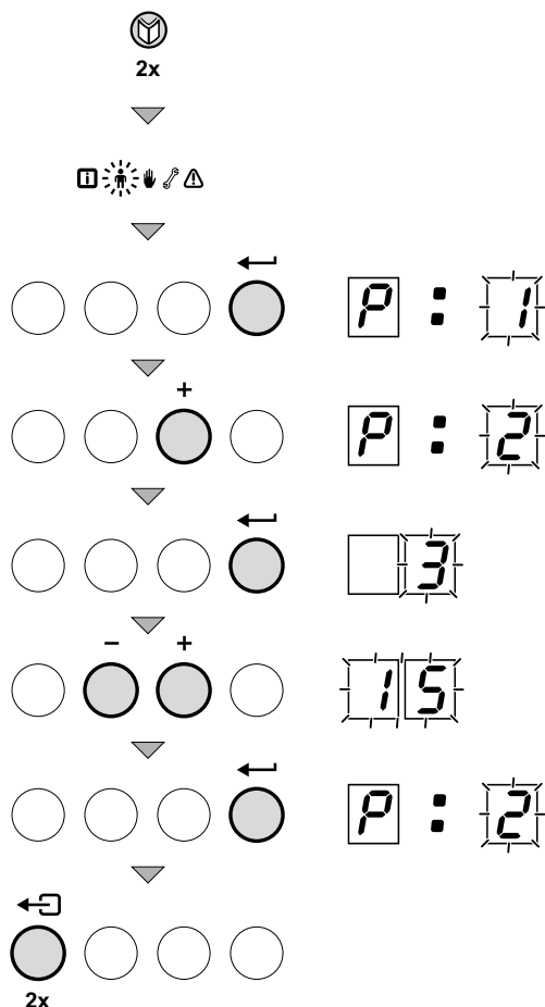
fig. 19 Modifica dei parametri
