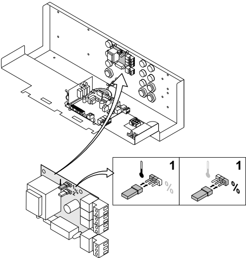
fig. 14 Ponticello 1 114492LTAL21H024
