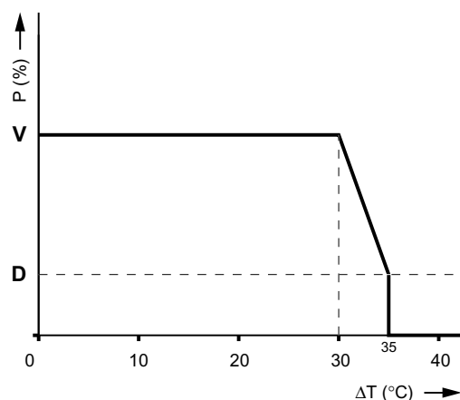
fig. 03 Caratteristiche della potenza erogata
