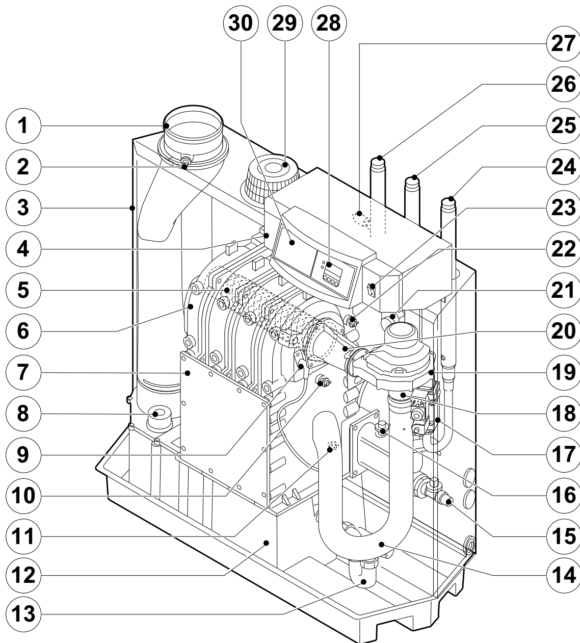
fig. 35 Sezione
