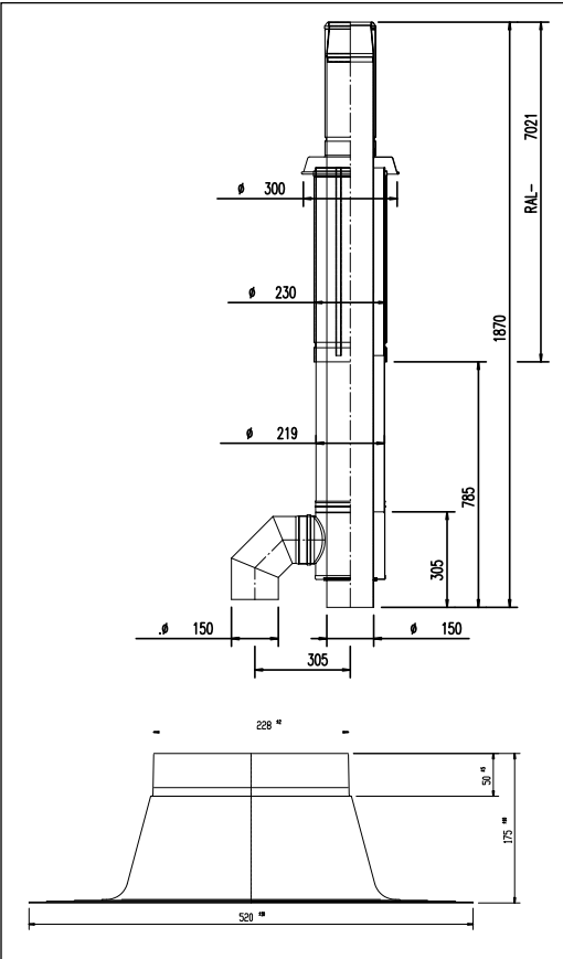
fig. 07 Attraversamento verticale per versione stagna
