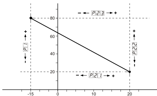
fig. 16 Grafico della curva climatica
