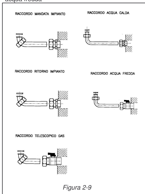
Kit raccordi a gomito telescopici con rubinetti gas e acqua fredda
