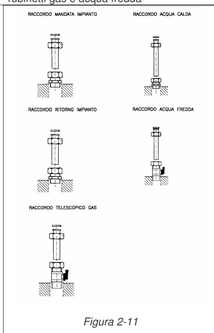
Kit raccordi verticali telescopici con rubinetti gas e acqua fredda
