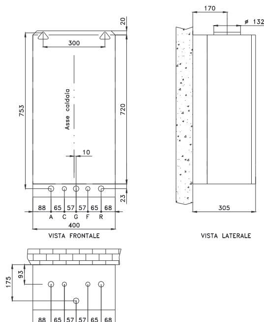
Figura 2-1 – Dima Millennium E
