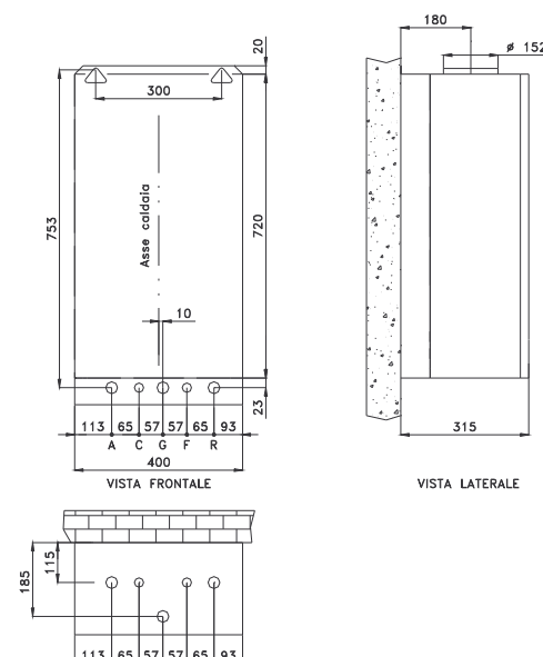
Figura 2-1 – Dima Millennium E
