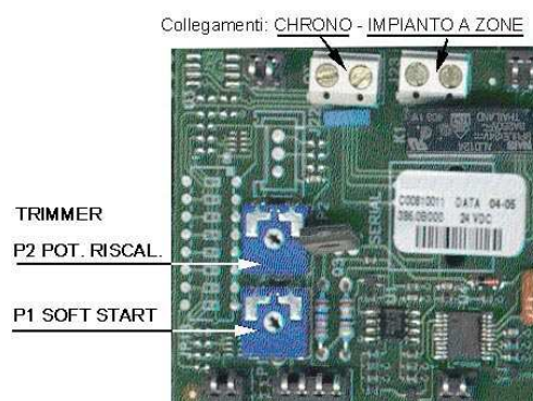
Figura 2-23 Scheda Modulino
