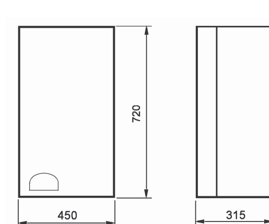
Figura 1-2 – Serie Millennium 26 E
