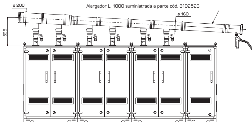
DEWY EQUIPE 360 BOX - Kit colector humos salida lado izquierdo y box contenedor separador hidráulico/kit seguridades
