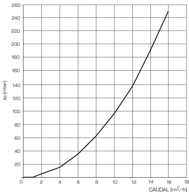
Separador hidráulico "DEWY EQUIPE 60-120-180-240 BOX/P60-P120 BOX"
