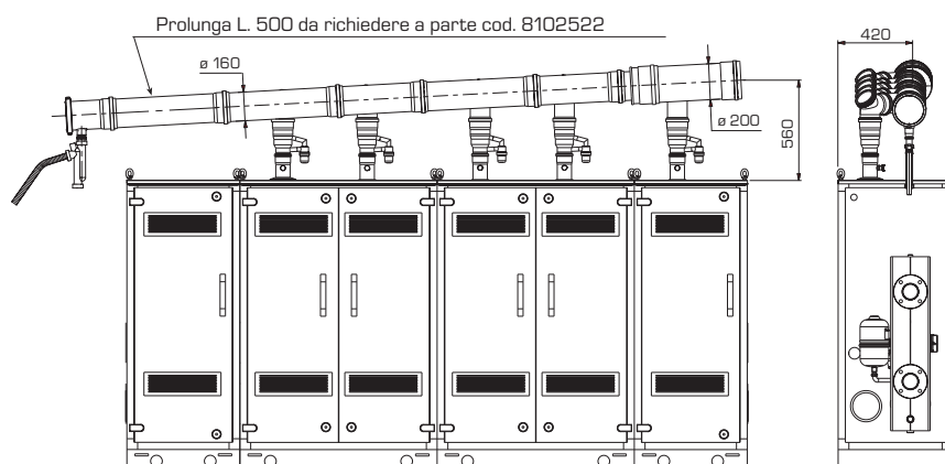
DEWY EQUIPE 300 BOX - Kit collettore fumi uscita lato dx e box contenitore separatore idraulico/kit sicurezze ISPESL
