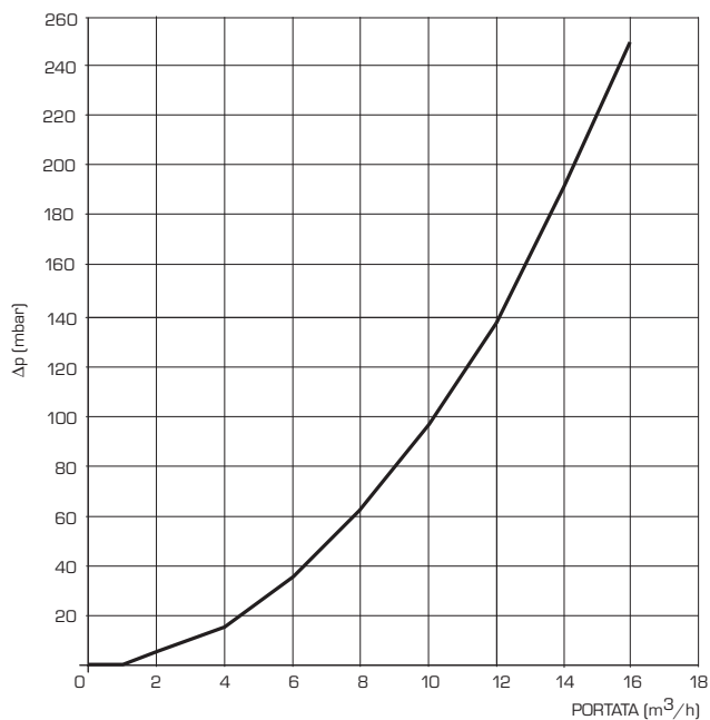
Compensatore idraulico "DEWY EQUIPE 60-120-180-240 BOX/P60-P120 BOX"
