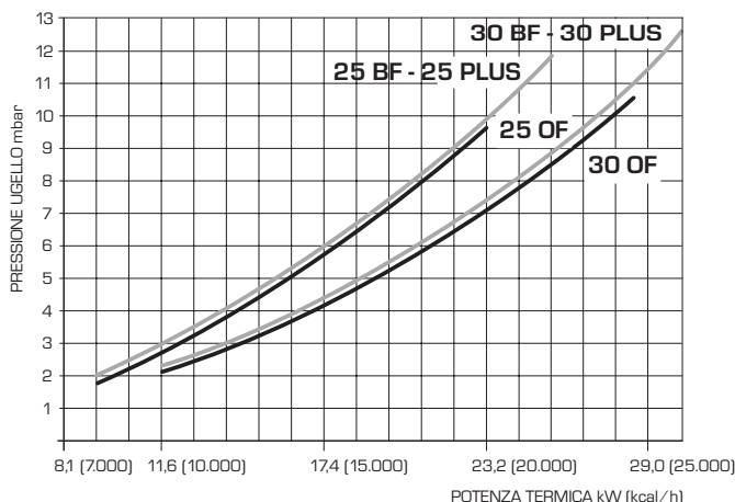
Diagramma pressione/potenza resa per gas naturale (G20)
