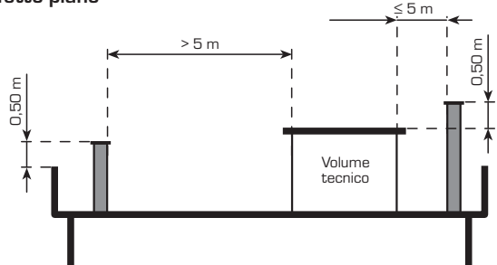
Tetto piano
