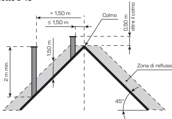
Tetto a 45°
