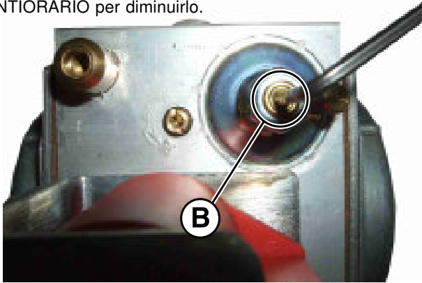
VITE DI REGOLAZIONE POTENZA MINIMA
