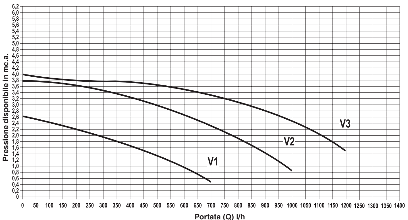
DIAGRAMMA PORTATA/PRESSIONE DISPONIBILE PER L'INSTALLAZIONE
