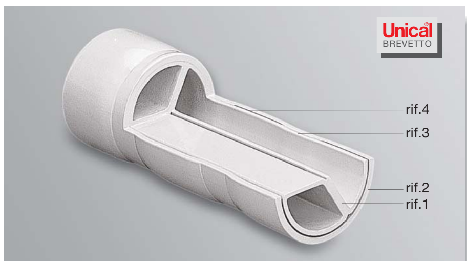
Tubo blindato a conduzione frenata (sez.)
