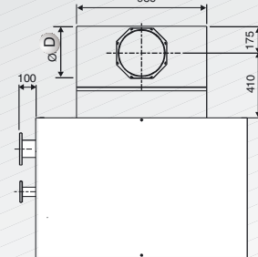
Vista superiore
