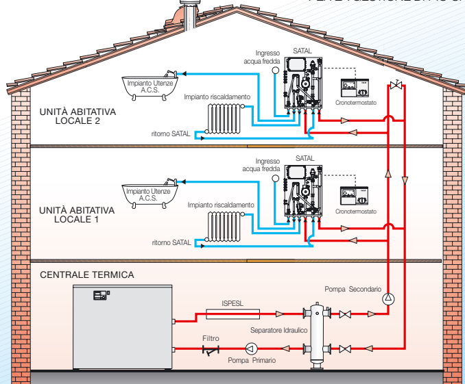
IMPIANTO CENTRALIZZATO CON MODULEX e SATAL PER LA GESTIONE DI PIÙ UNITÀ ABITATIVE
