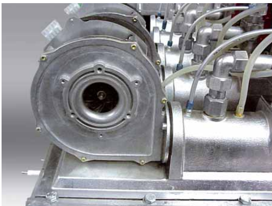
Particolare del ventilatore per la premiscelazione.
