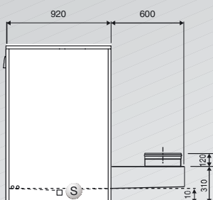
Vista laterale destra
