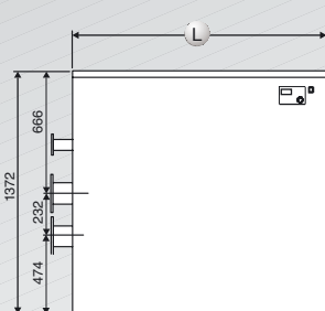
Vista frontale
