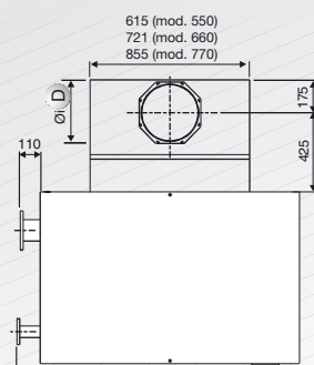
Vista superiore
