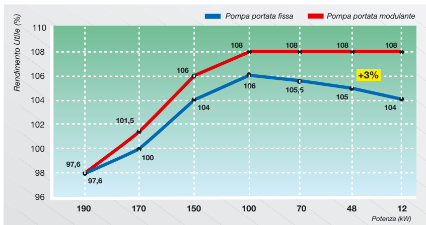
RAFFRONTO DEL RENDIMENTO CON POMPA MODULANTE E POMPA A PORTATA FISSA IN UNA MODULEX 190 AL VARIARE DELLA POTENZA RICHIESTA.
