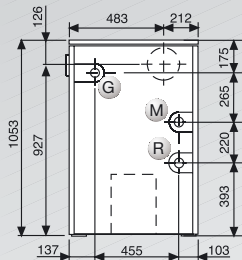
Vista laterale destra
