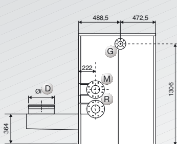
Vista laterale sinistra
