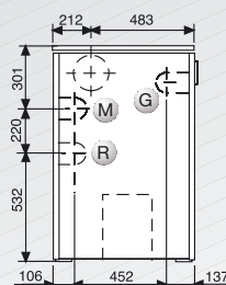
Vista laterale sinistra
