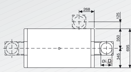
Vista superiore
