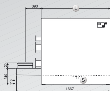
Vista frontale
