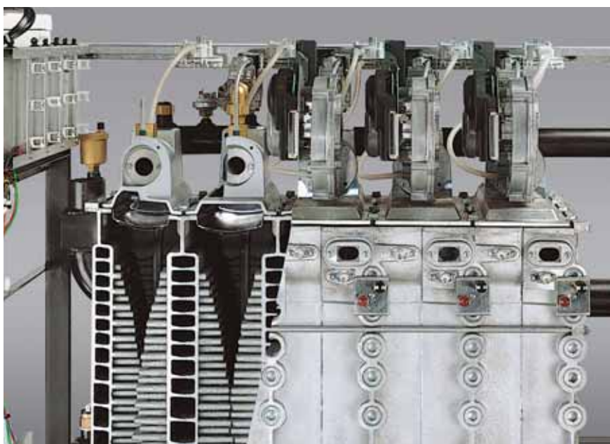
Vista frontale del sistema moduli con sezione della parte idraulica
