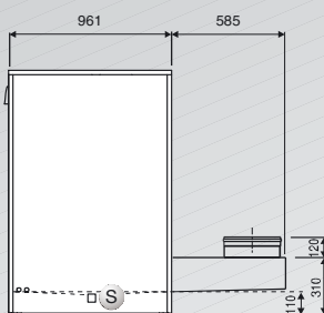
Vista laterale destra
