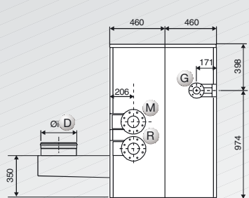
Vista laterale sinistra
