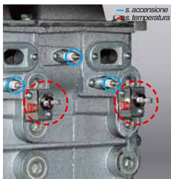
SICUREZZE ACCENSIONE E TEMPERATURA
