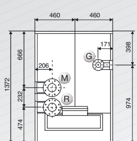
Vista laterale sinistra
