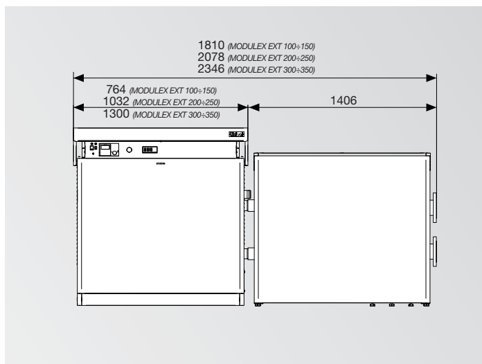
OGNITEMPO con SEPARATORE IDRAULICO
