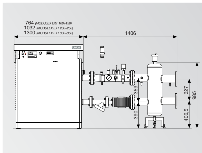
SEPARATORE IDRAULICO
