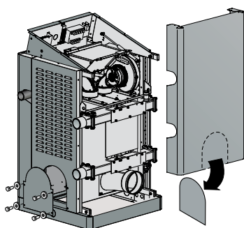
KIT CHIUSURA PRETRANCIO per MODULEX EXT 100÷200 Cod. 00362154
