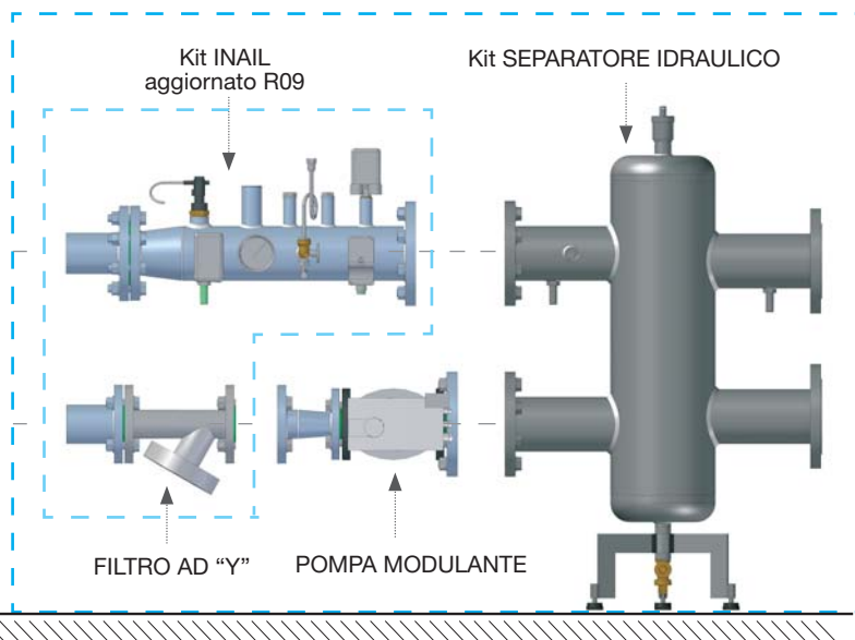
Composizione ANELLO PRIMARIO
