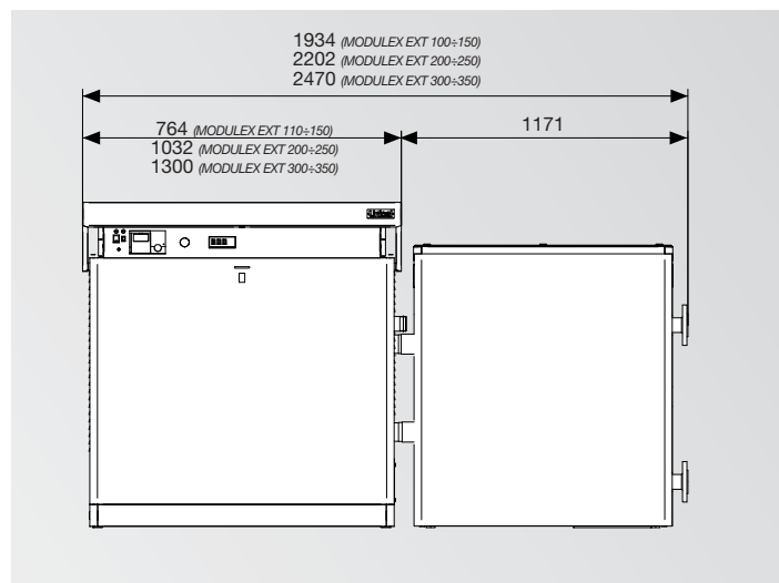
OGNITEMPO con SCAMBIATORE A PIASTRE
