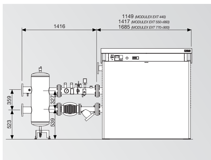
SEPARATORE IDRAULICO
