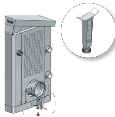
KIT SUPPORTO TERMINALE FUMI Cod. 00362075
