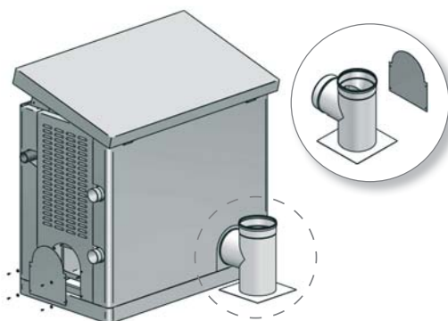
KIT SCARICO FUMI POSTERIORE per MODULEX EXT 250÷350 Cod. 00362076
