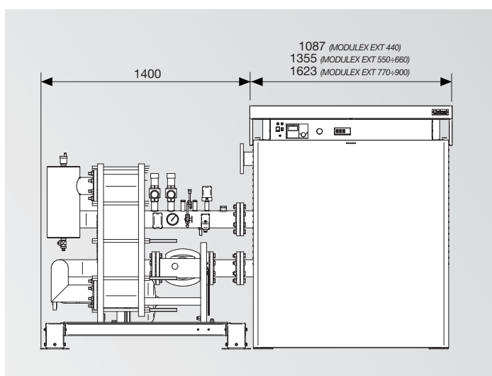
SCAMBIATORE A PIASTRE
