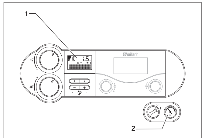
Fig. 4.15 Controllo della pressione di riempimento dell'impianto di riscaldamento
