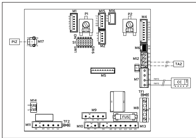
Fig. 4.8 Scheda elettronica caldaia
