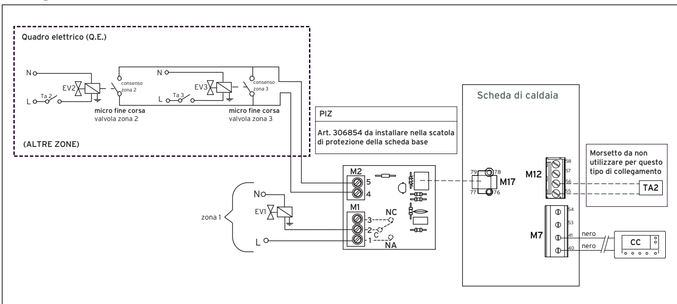
Fig. 4.5 Schema elettrico con scheda kit impianto a zone
