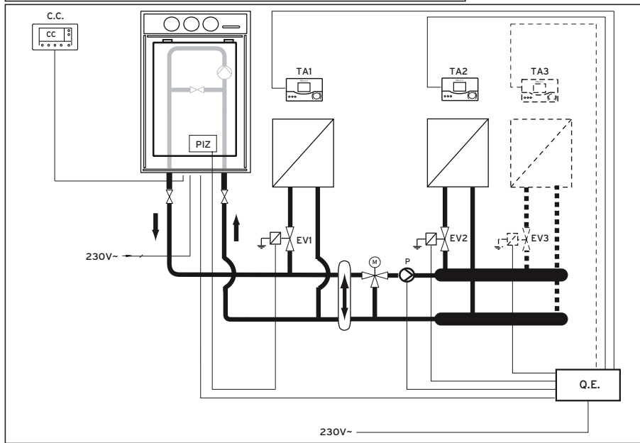
Fig. 4.9 Scheda idraulico di riferimento
