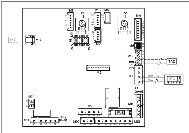
Fig. 4.3 Scheda elettronica caldaia
