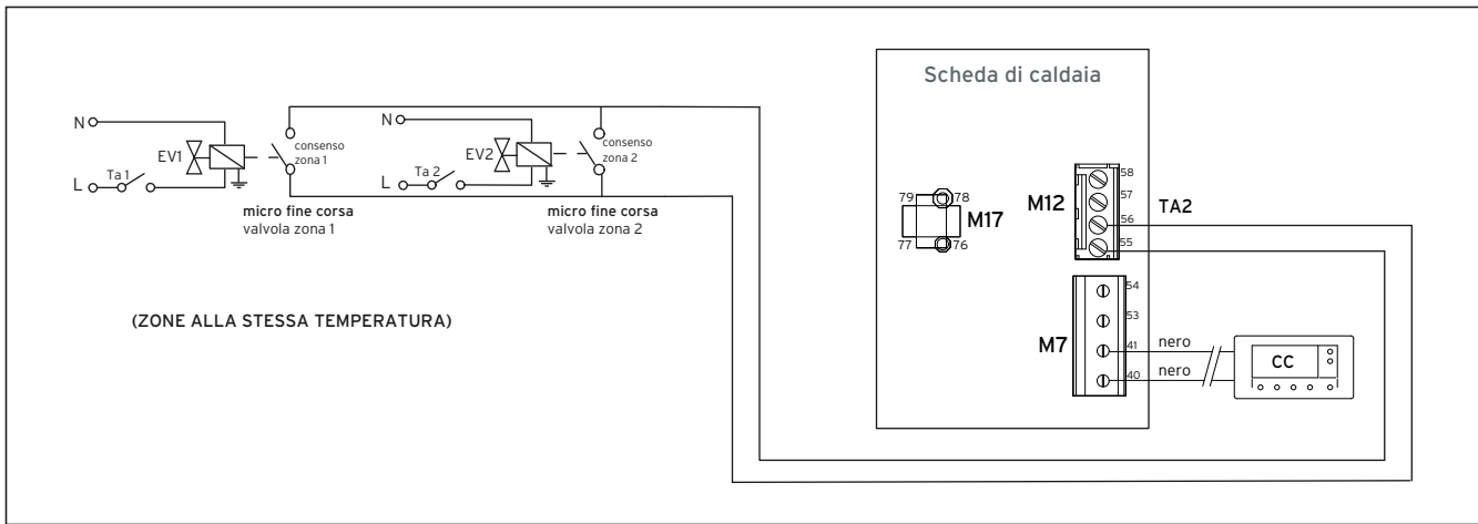
Fig. 4.6 Schema elettrico senza scheda kit impianto a zone
