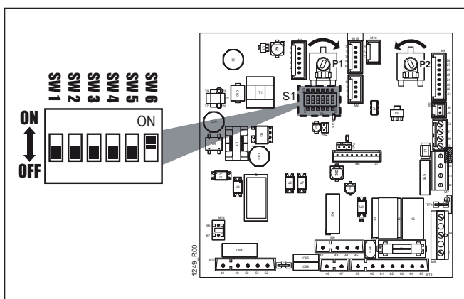
Fig. 4.12 Scheda di modulazione
