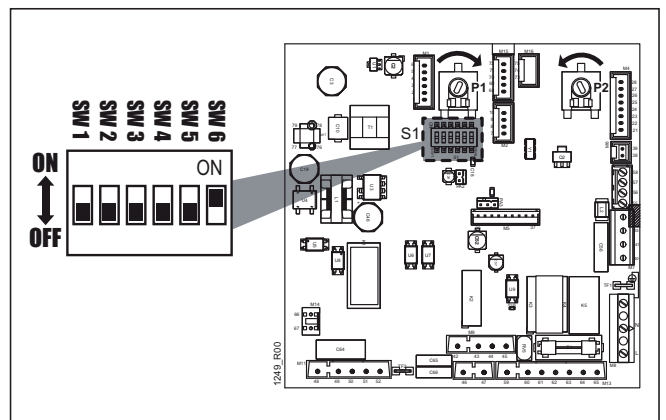
Fig. 4.7 Scheda di modulazione
