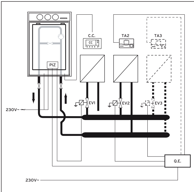
Fig. 4.4 Schema idraulico di riferimento
