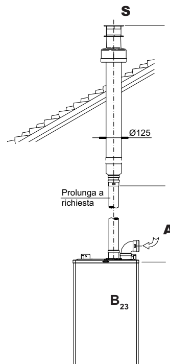
SISTEMA TUBI SEPARATI SCARICO VERTICALE (ASPIRAZIONE DIRETTA)
