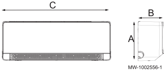
Fig.87 Unidade interior
