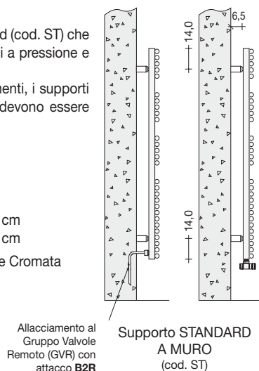
Interasse l=L+13,8 cm
