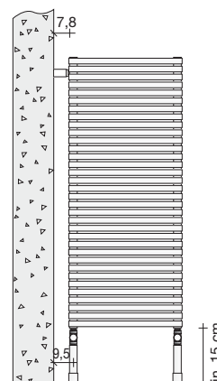
Supporto Bandiera A MURO (cod. MD muro DX cod. MS muro SX)
