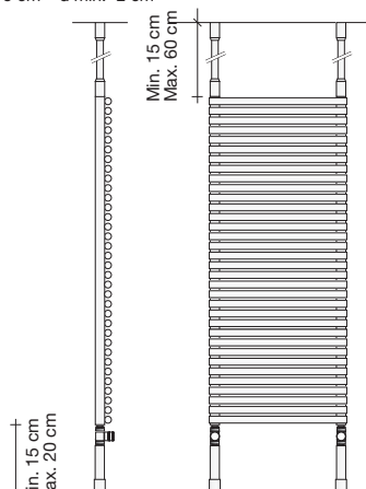
Supporto Bandiera A SOFFITTO (cod. SO)
