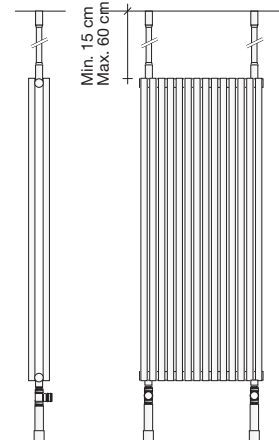
Supporto Bandiera A SOFFITTO (cod. SO)
