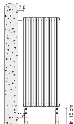
Supporto Bandiera A MURO (cod. MD muro DX cod. MS muro SX)
