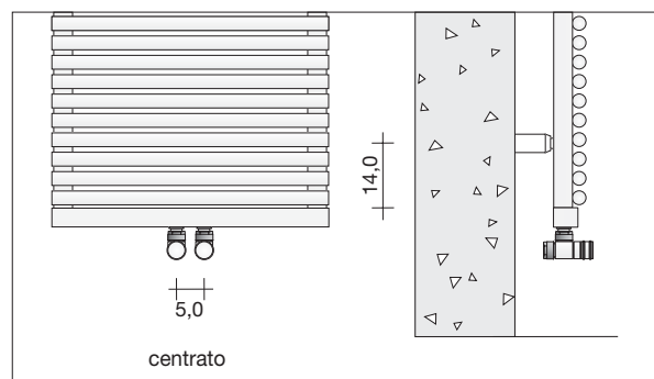
Schema tecnico allacciamento BA25 i5
