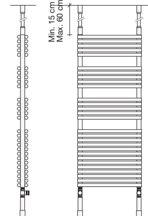
Supporto Bandiera A SOFFITTO (cod. SO)
