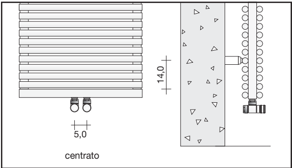
Schema tecnico allacciamento BA25D i5
