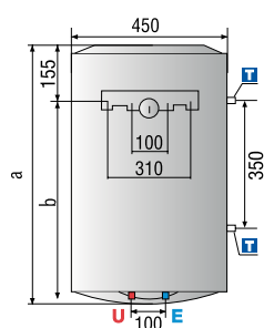
Versione VERTICALE
