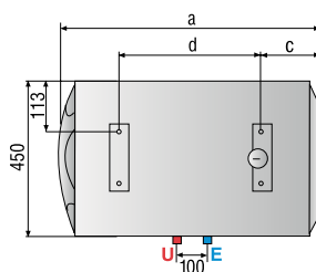
Versione ORIZZONTALE
