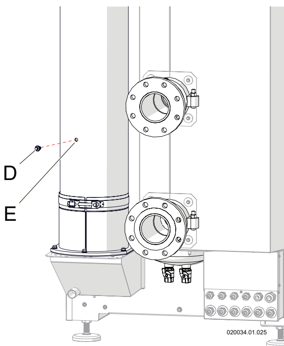
Figura 6-7 - Foro per analisi combustione
