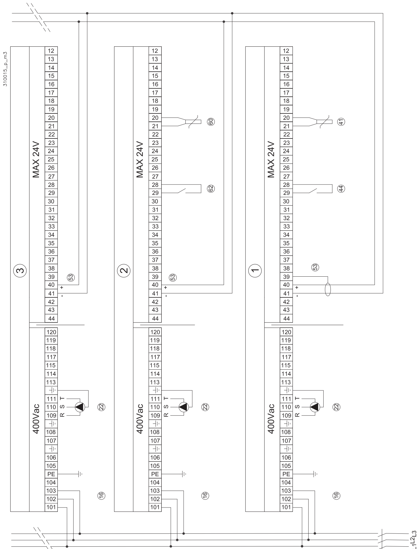
Figura 5-27 - Esempio di collegamento elettrico della cascata con due MASTER (modelli 1100) (per i modelli 495 e 750 occorre aggiungere il cavo di neutro)
