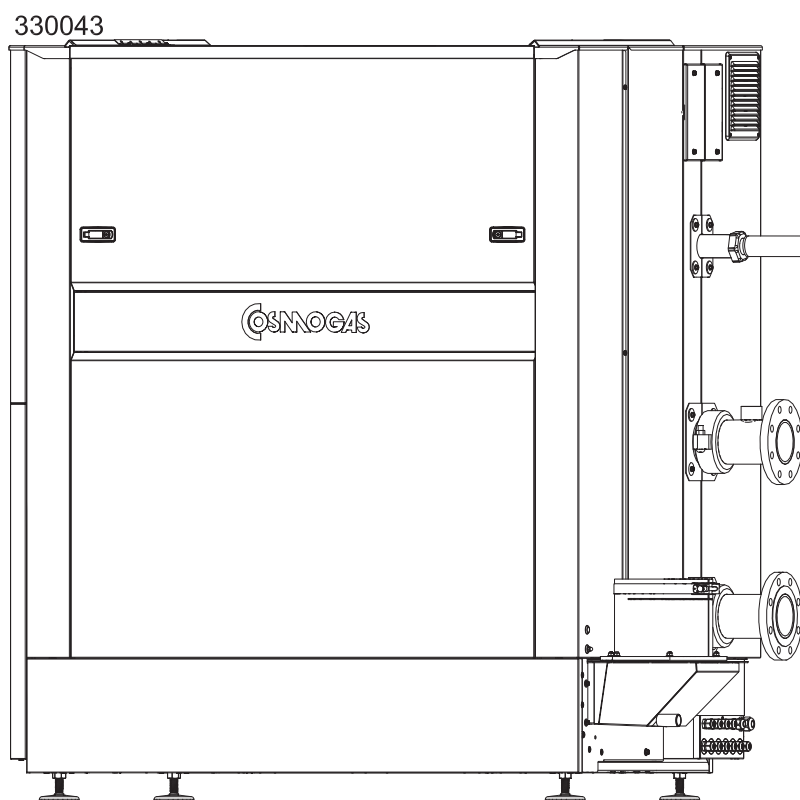
Figura 5-7 - Collegamento gas
