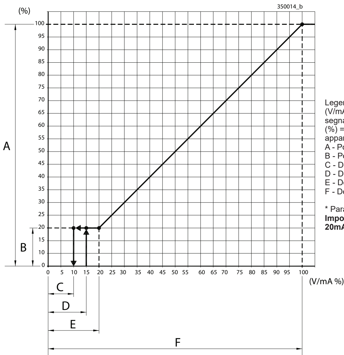
Figura 5-22 - Grafico del controllo della potenza del bruciatore in funzione del segnale 0-10Vdc o 4-20mA
