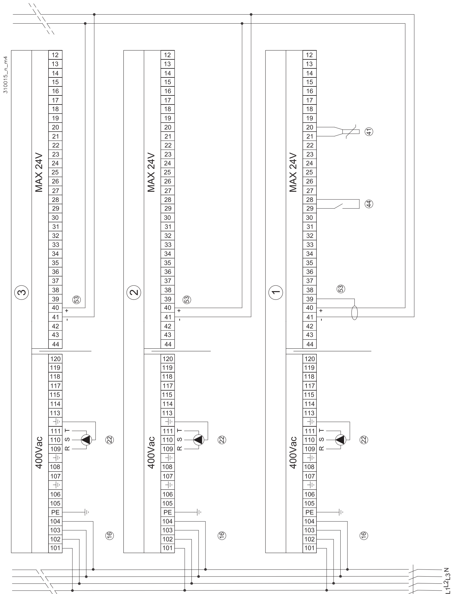
Figura 5-25 - Esempio di collegamento elettrico della cascata con un MASTER (modelli 495 e 750) (per modelli 1100 non è necessario collegare il neutro)
