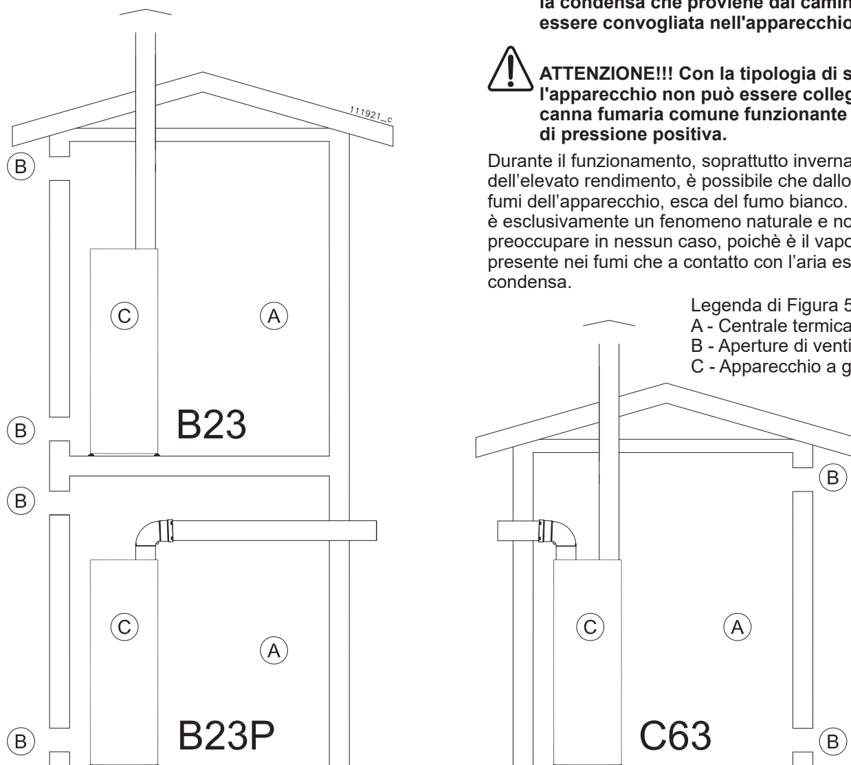
Figura 5-29 - Sistemi di aspirazione/scarico
