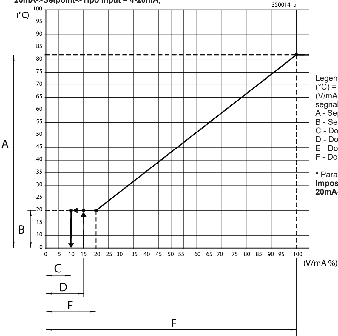
Figura 5-20 - Grafico del controllo della temperatura di setpoint in funzione del segnale 0-10Vdc o 4-20mA
