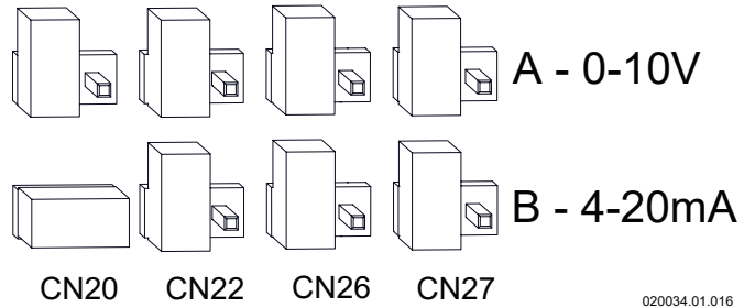
Figura 5-21 - Posizione jumper per segnale esterno 0-10V / 4-20mA (jumper nel quadro elettrico, Figura 3-4)
