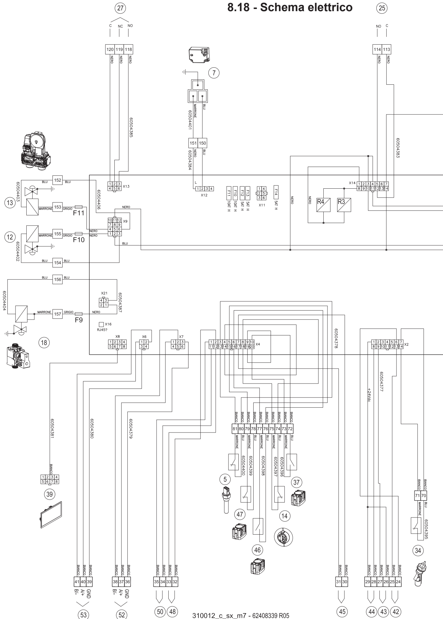
Figura 8-26 - Schema elettrico
