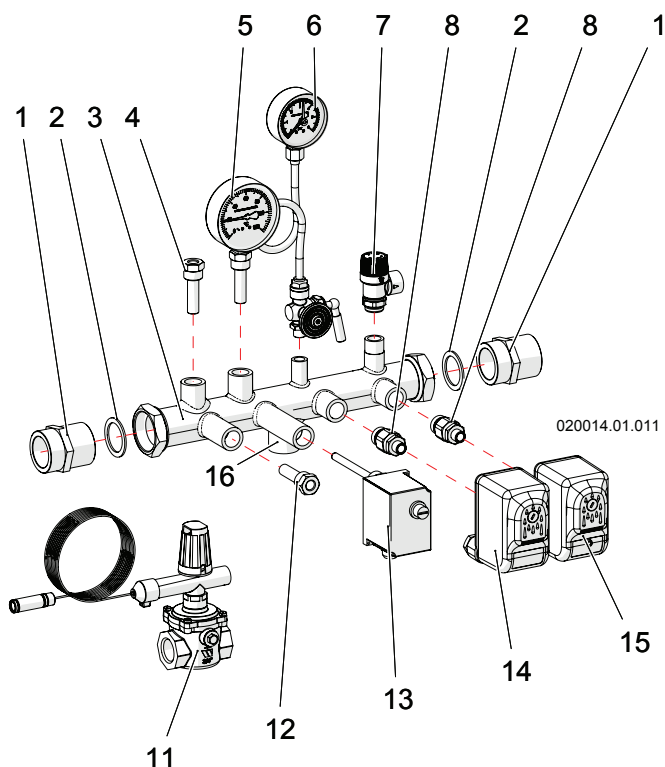
Figura 5-17 - Kit per modelli 60T-70T-100T-115T-140T
