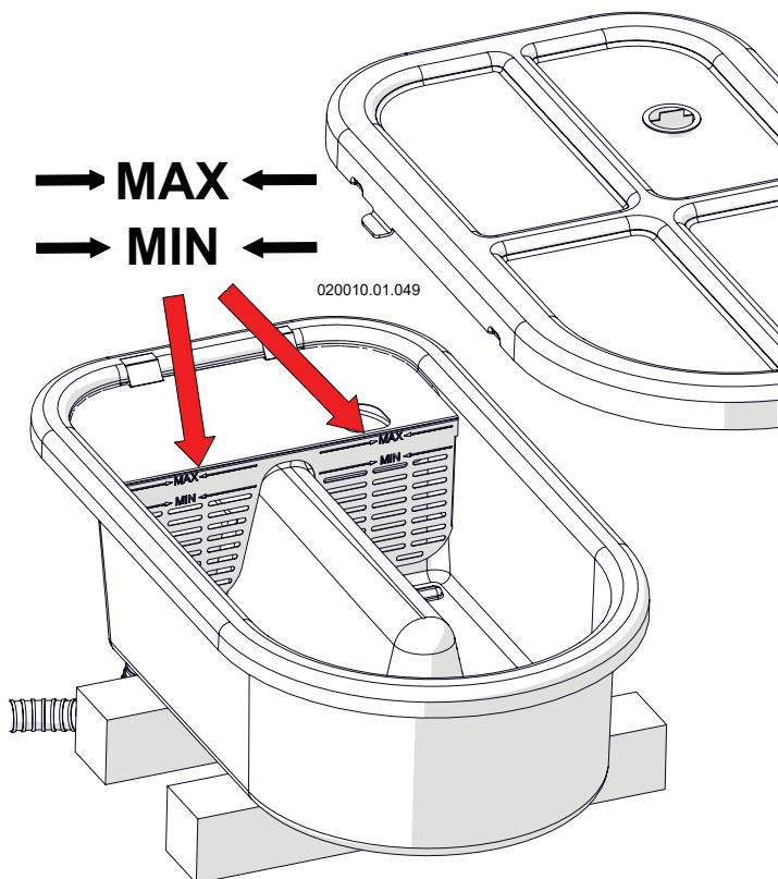
Figura 6-1 - Riempimento box con sali di neutralizzazione
