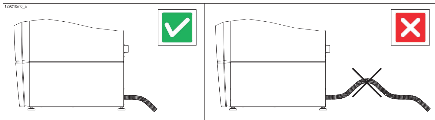
Figura 5-24 - Corretta pendenza del tubo di scarico
