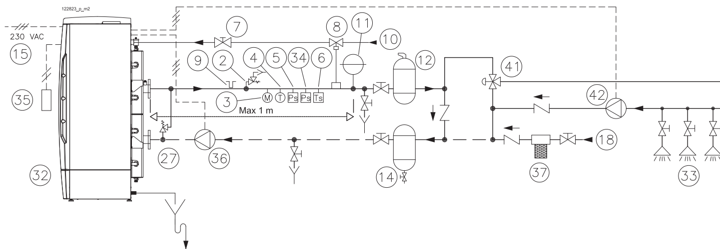
Figura 5-15 - Esempio di schema di collegamento per produzione istantanea
