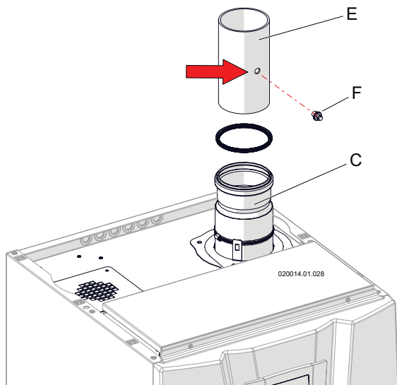
Figura 5-31 - Collegamento scarico fumi
