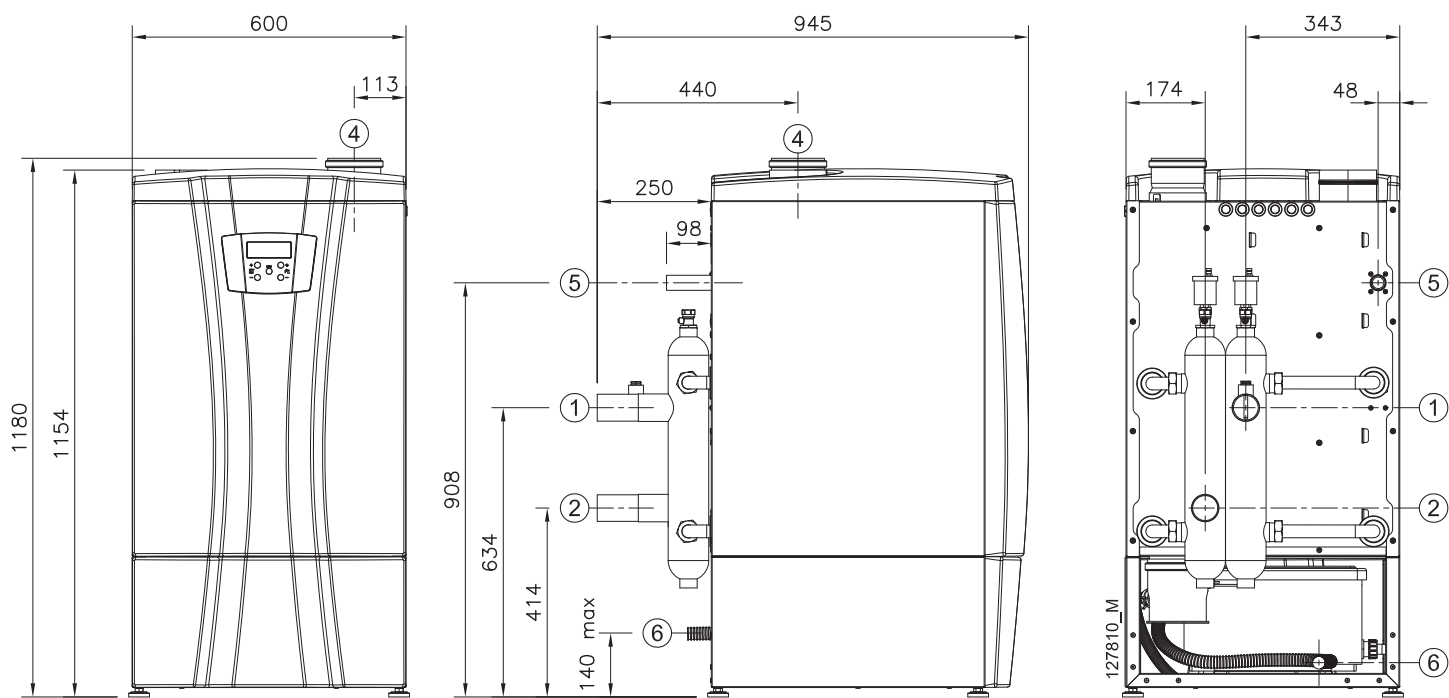
Figura 5-10 - Dimensioni modelli 60T-70T-100T-115T-140T (riferimenti in tabella Figura 5-12)
