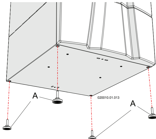
Figura 5-6 - Piedini regolabili
