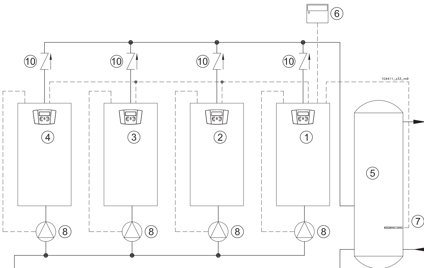
Figura 5-29 - Collegamento in cascata
