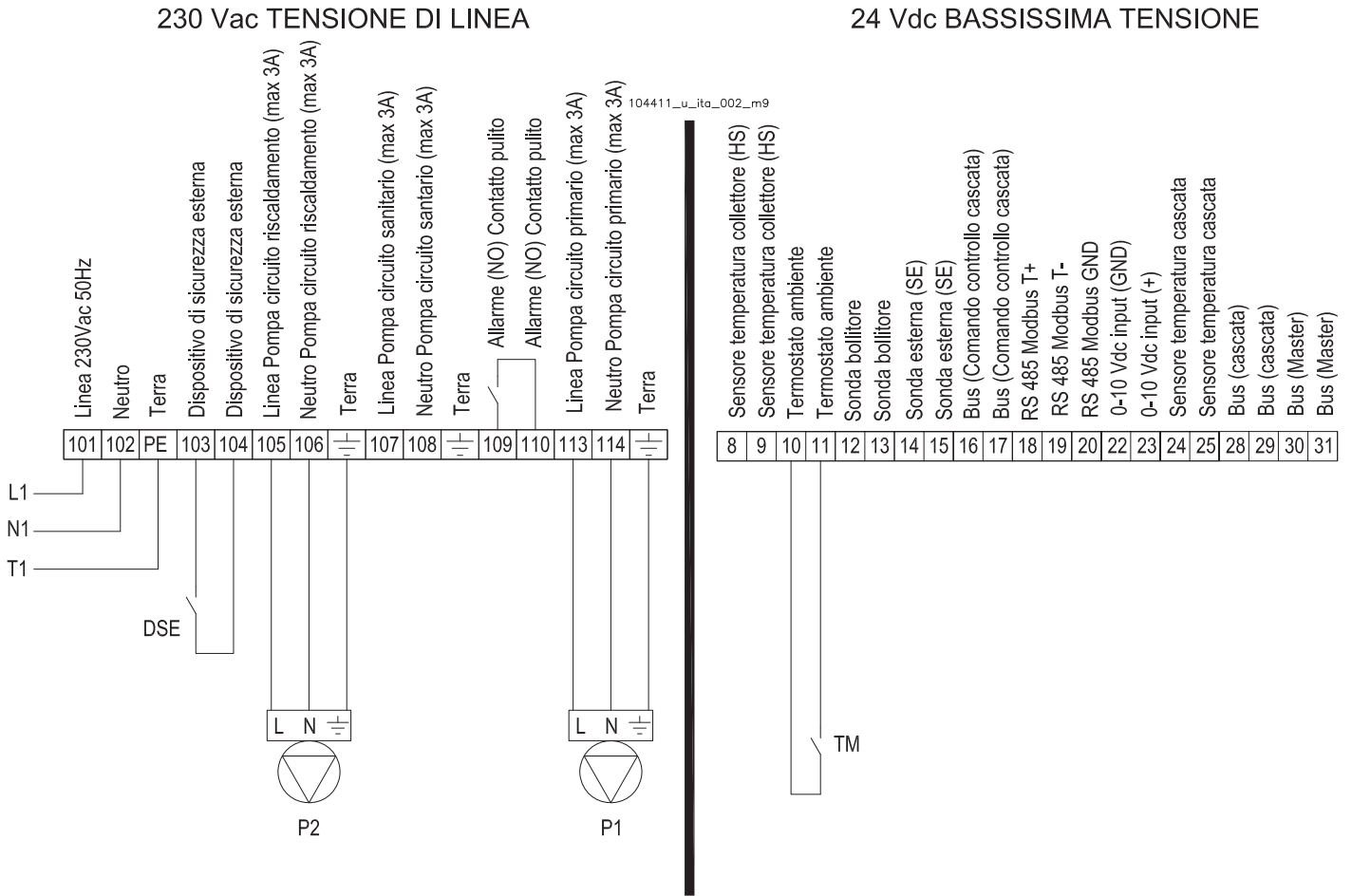
Figura 5-27 - Collegamento per produzione istantanea (vedi Figura 5-15)
