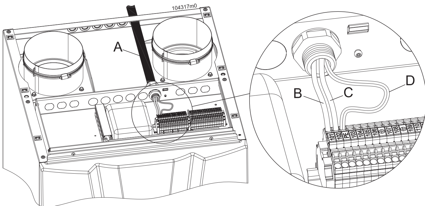
Figura 5-25 - Allacciamento alimentazione elettrica
