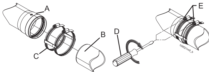
Figura 5-33 - Fissaggio dei condotti di scarico
