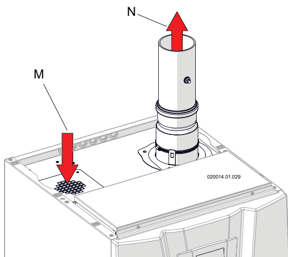
Figura 5-32 - Collegamento scarico fumi
