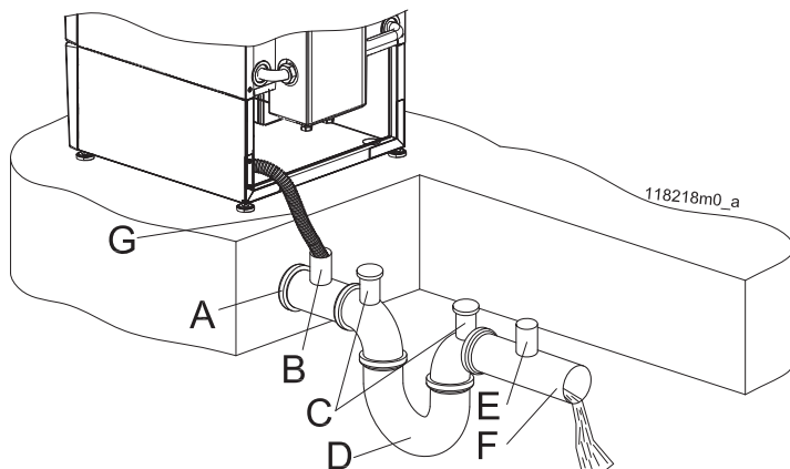
Figura 5-23 - Installazione scarico condensa
