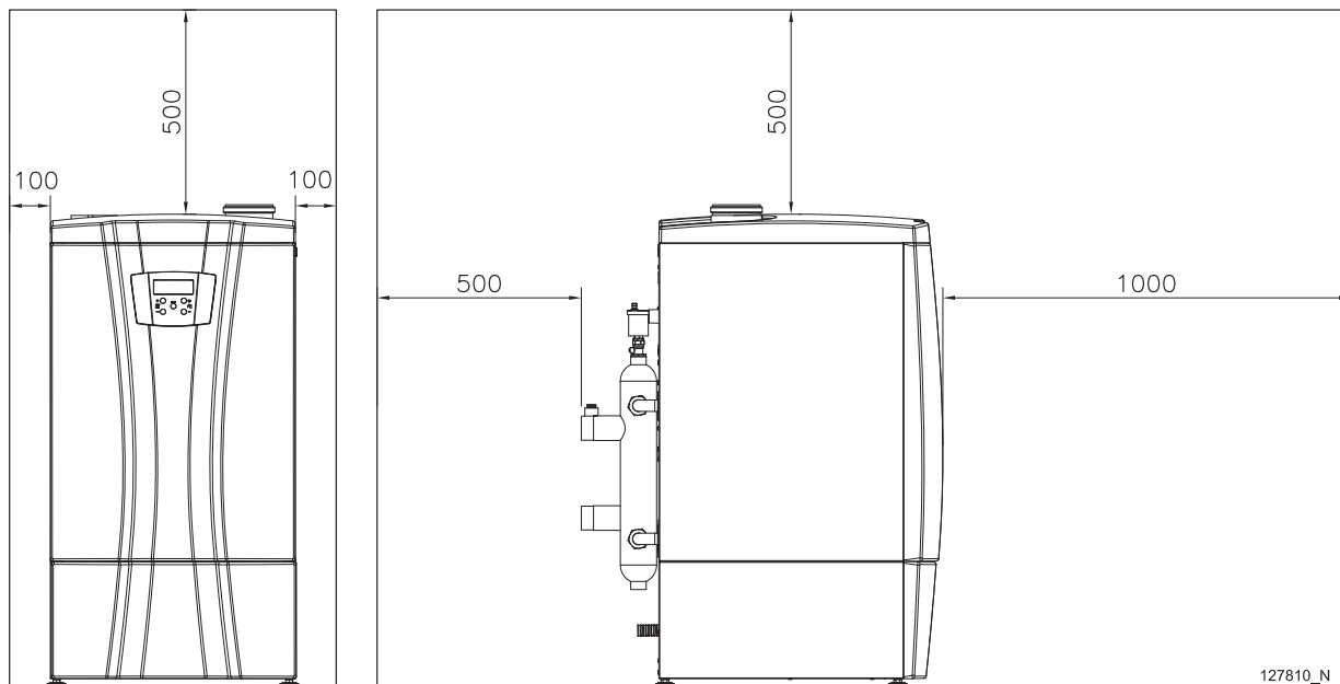
Figura 5-8 - Distanze minime di rispetto modelli 60T-70T-100T-115T-140T
