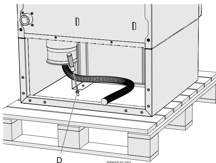
Figura 5-4 - Rimozione del bancale
