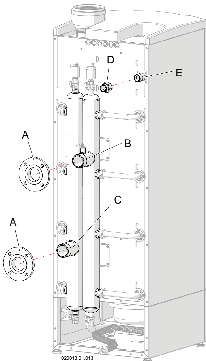
Figura 5-14 - Modelli 180T-210T-280T
