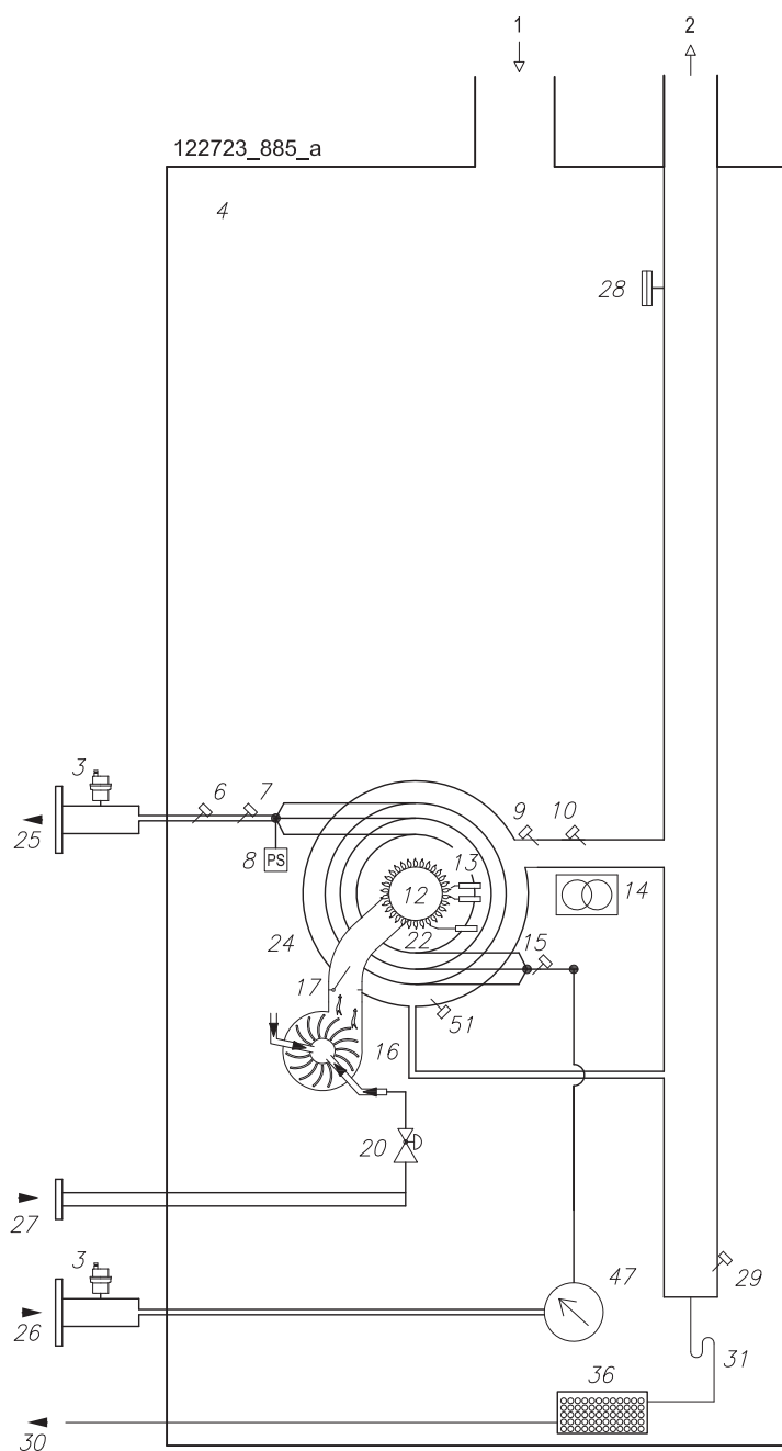
Figura 4-1 - Modelli 60T-70T
