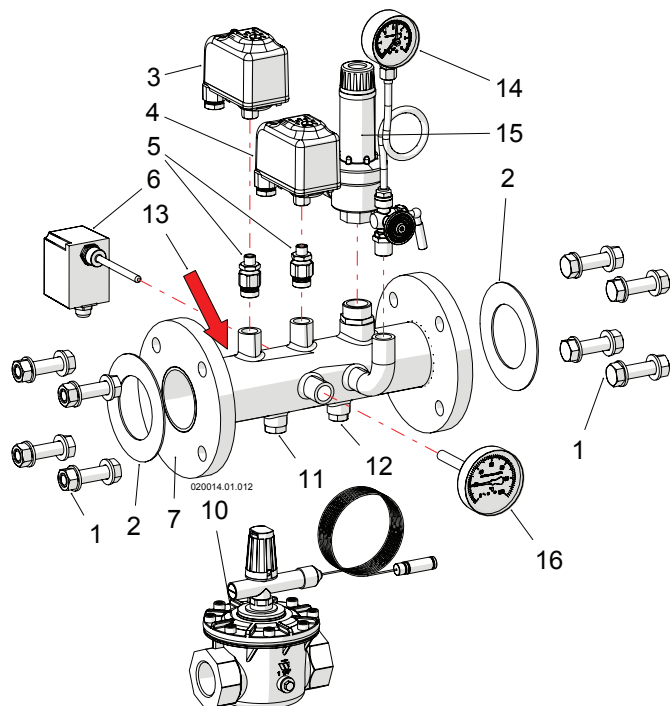
Figura 5-18 - Kit per modelli 180T-210T-280T
