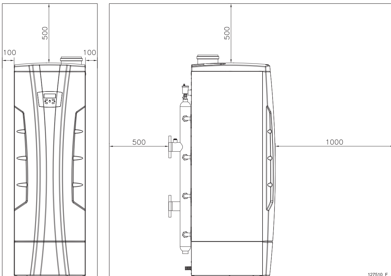
Figura 5-9 - Distanze minime di rispetto modelli 180T-210T-280T
