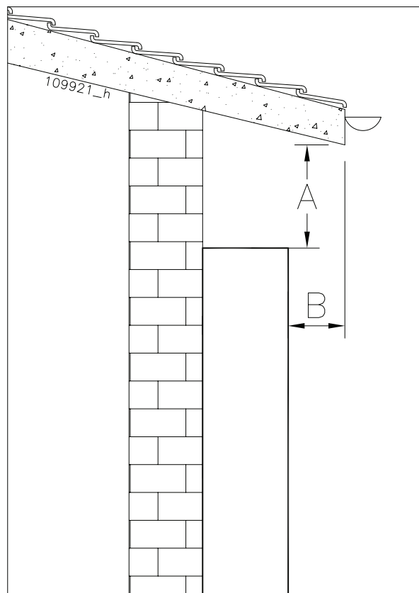
Figura 5-1 - Esempio di luogo parzialmente protetto
