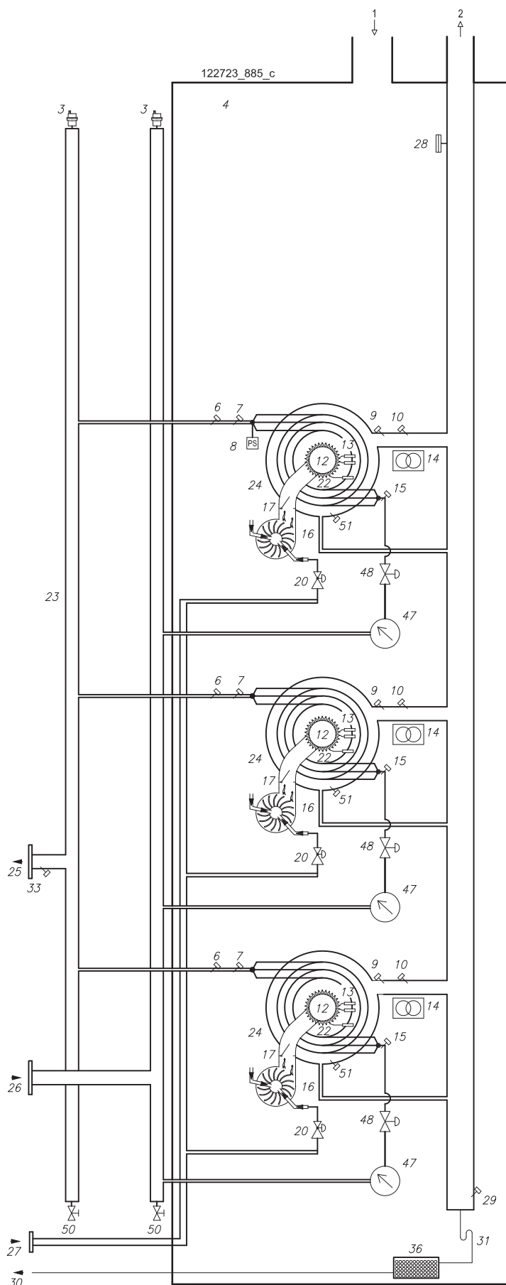
Figura 4-3 - Modelli 180T-210T
