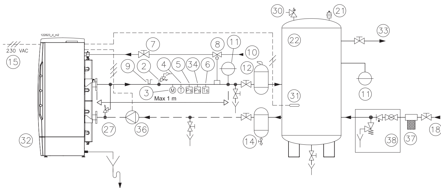
Figura 5-16 - Esempio di schema di collegamento con bollitore
