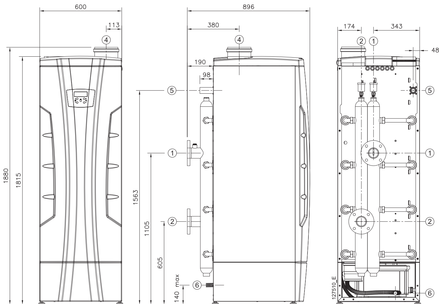
Figura 5-11 - Dimensioni modelli 180T-210T-280T (riferimenti in tabella Figura 5-12)
