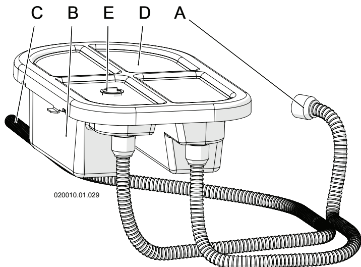
Figura 5-22 - Box neutralizzazione condensa
