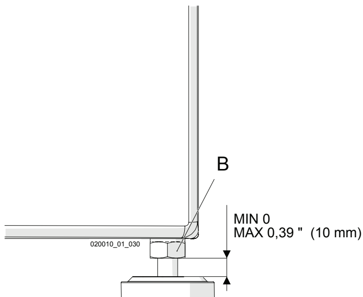
Figura 5-7 - Piedini regolabili
