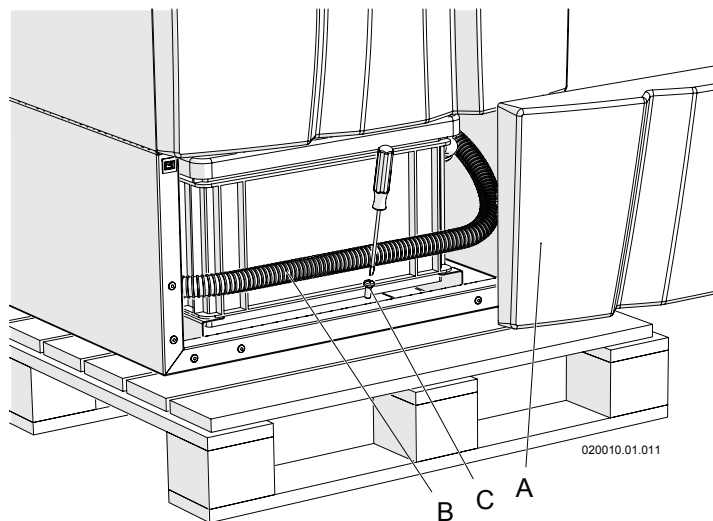
Figura 5-3 - Rimozione del bancale
