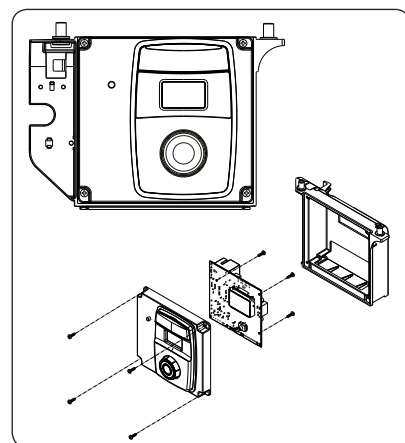
Fig. 15 - Accessibilità alla scheda elettronica
