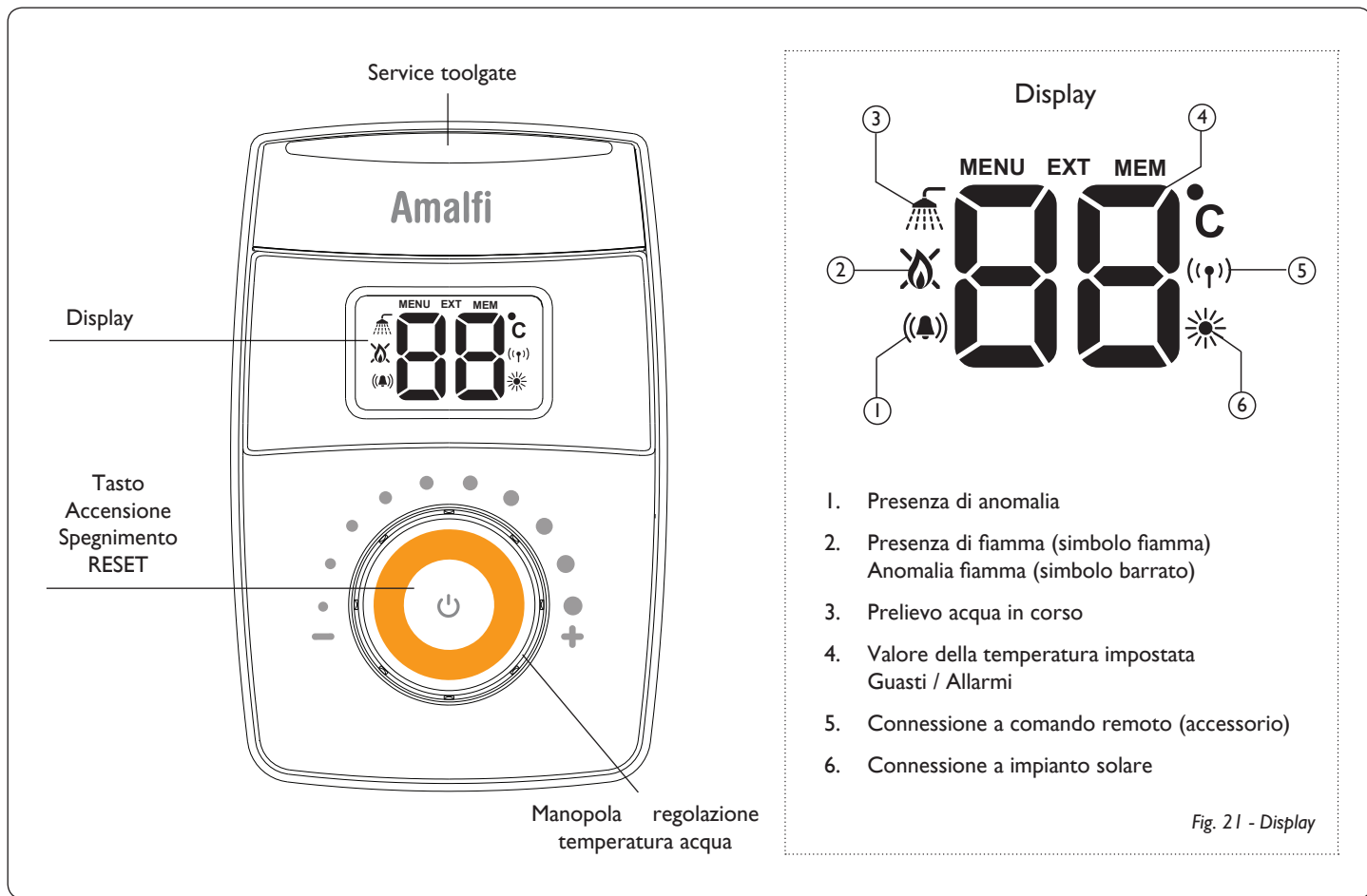
Fig. 20 - Pannello comandi e display
