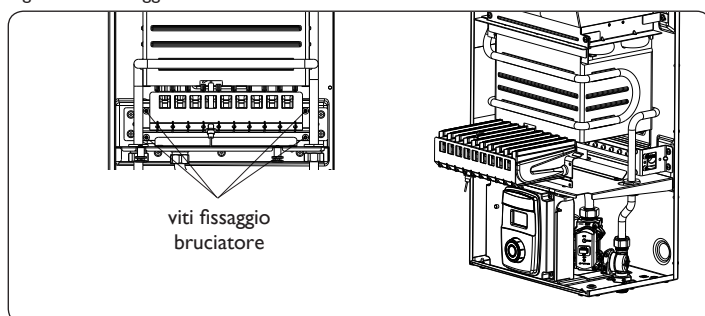
Fig. 19 - Smontaggio bruciatore
