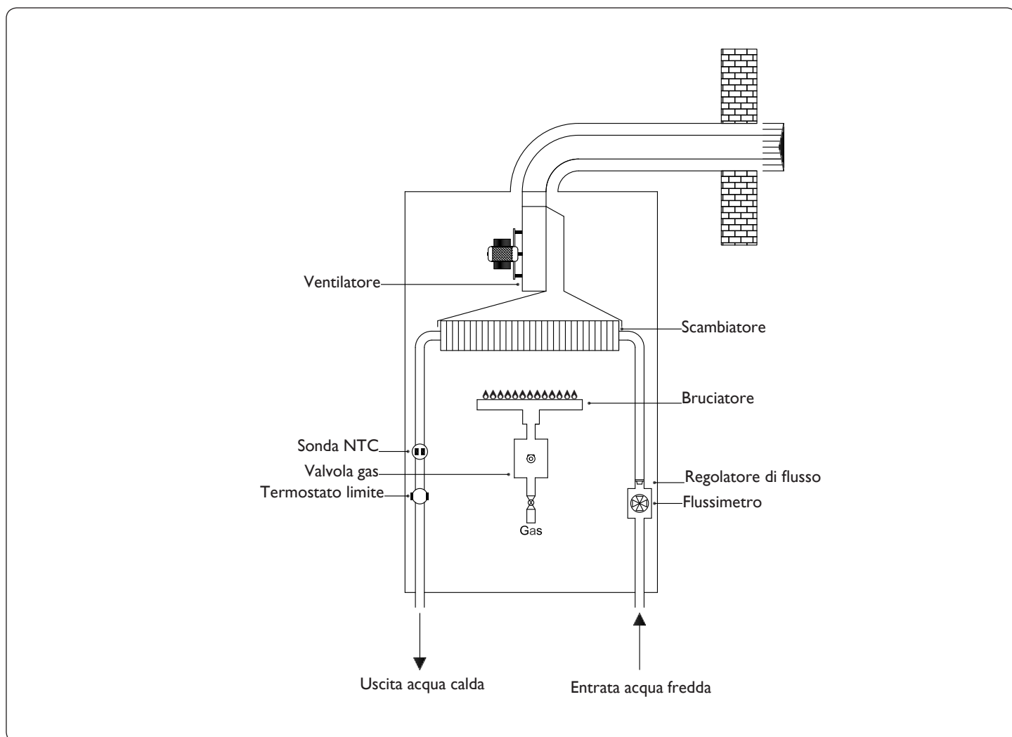
Fig. 3 - Circuito idraulico
