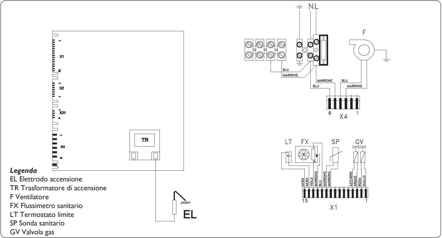
Fig. 4 - Schema elettrico
