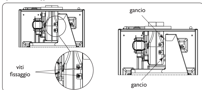
Fig. 18 - Smontaggio scambiatore
