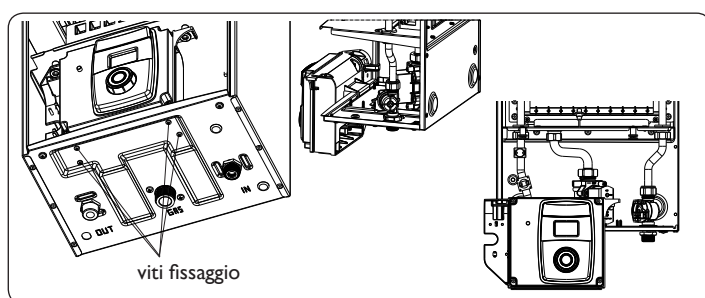
Fig. 17 - Smontaggio ventilatore
