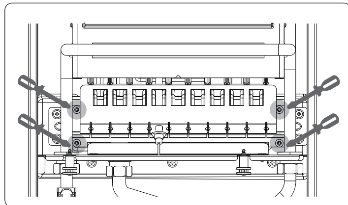
Fig. 12 - Smontaggio bruciatore
