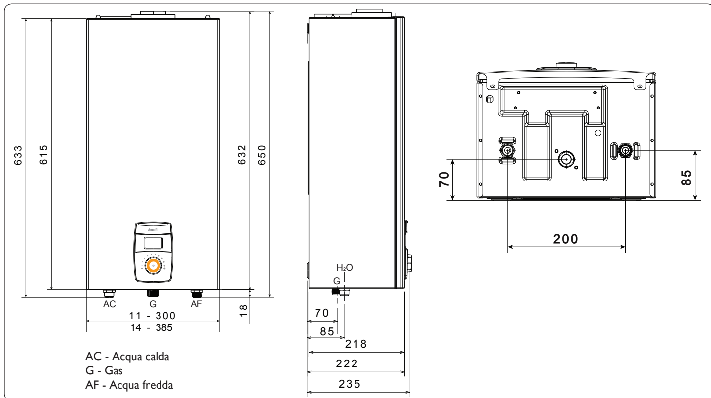
Fig. 2 - Dimensioni d'installazione - Misure in mm
