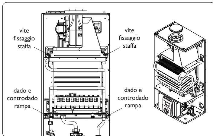
Fig. 19 - Smontaggio bruciatore
