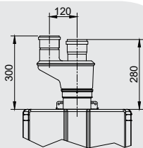
INGOMBRO SDOPPIATORE ø80/80 Dimensioni in mm
