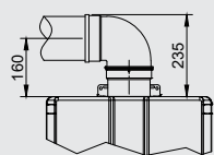
INGOMBRO SCARICO A PARETE ø80/125 Dimensioni in mm
