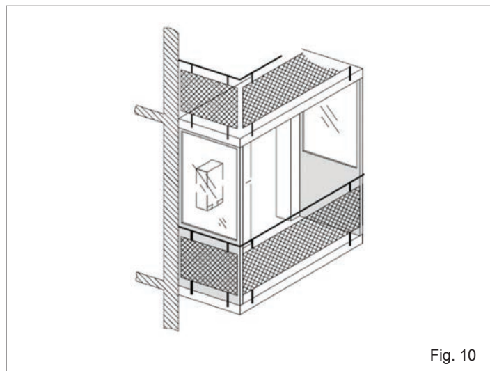
Fig. 10: exemple d'évacuation INCORRECTE des produits de la combustion à l'intérieur d'un balcon fermé sur cinq côtés.
