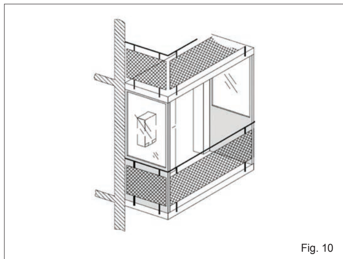
Fig. 10: ejemplo de evacuación INCORRECTA de los productos de la combustión dentro de un balcón cerrado en cinco lados.
