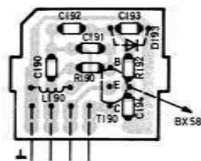
Submodul Submodule 592.974 TCB 5000 Sub-module Lötseite - Lato saldature - Soldered side
