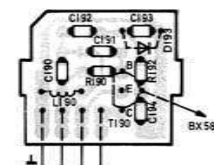
Submodul Submodulo 592.974 TCB 5000 Sub-module Lötseite - Lato saldature - Soldered side
