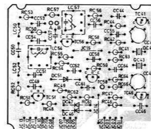
NTSC-Modul Modulo NTSC 592.970 NTSC-Module Lötseite - Lato saldature - Soldered side
