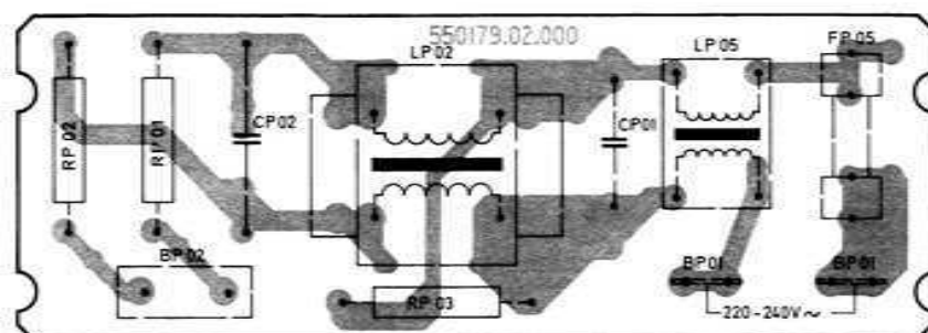
Leiterplatte Netzfilter Piastra bobina d'arresto 527.436 P.C.B. Mains filter Lötseite - Lato saldature - Soldered side
