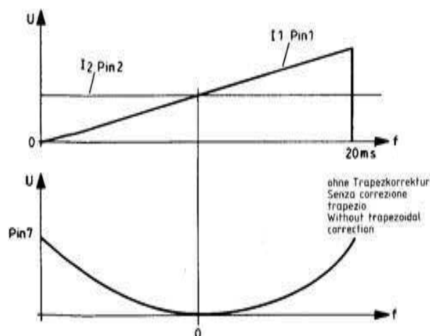
Fig. 15 Vertikalparabel-Aufbereitung Preparazione parabola verticale Preparation of vertical parabola
