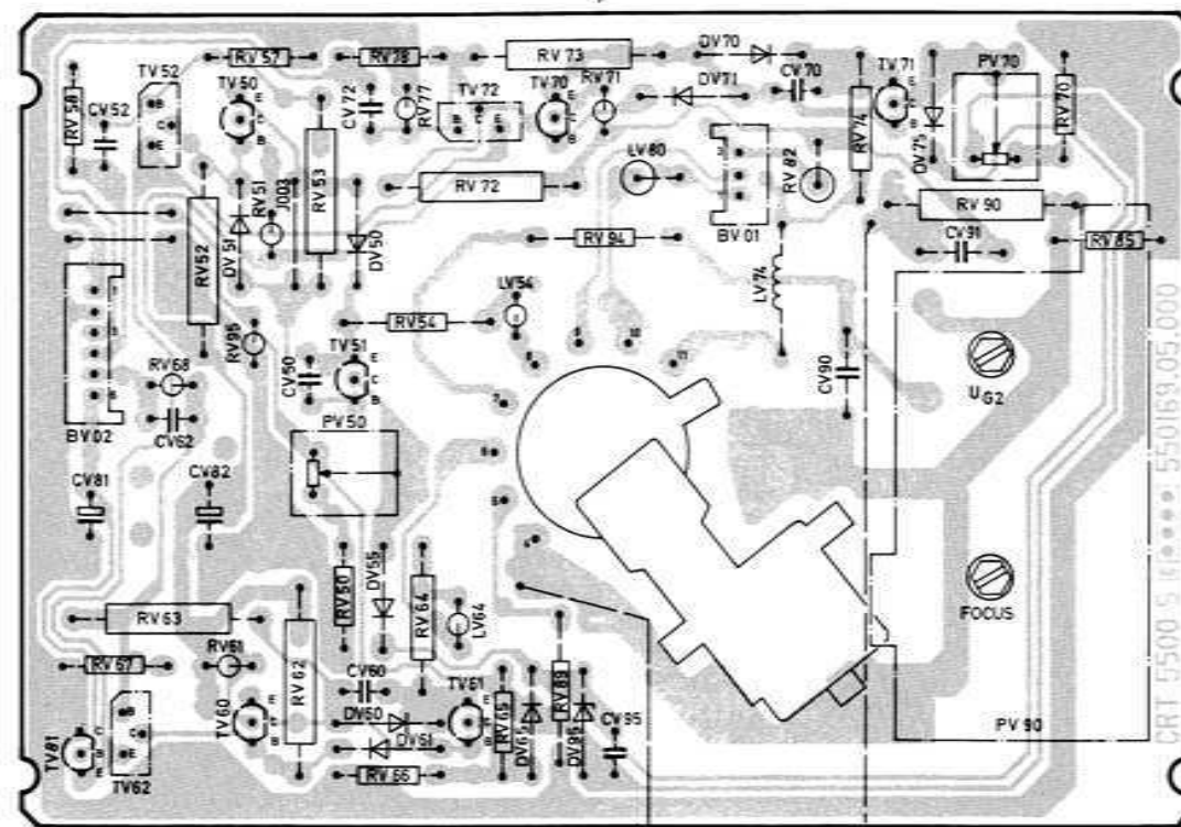
Bildrohranschluß-Platine Piastra zoccolo cinescopio 592.977 P.C.B. CRT socket Lötseite - Lato saldature - Soldered side
