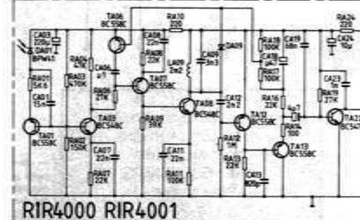
RIR4000 RIR4001 Infrarot-Vorverstärker Preamplificatore infrarossi 583.521 B Infra-red pre-amplifier
