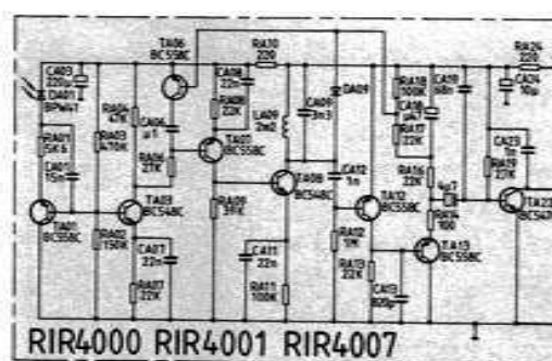
Infrarot-Vorverstärker Preamplificatore infrarossi Infra-red pre-amplifier 583.521 C
