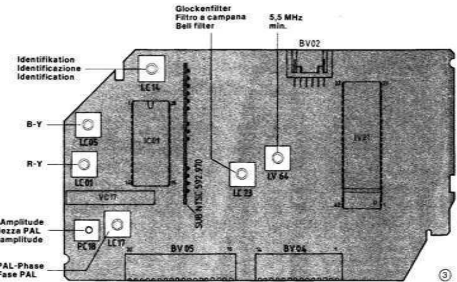
Chroma-Video-Modul Modulo crominanza video Chroma video module 592.963 Bestückungsseite - Lato componenti - Component side
