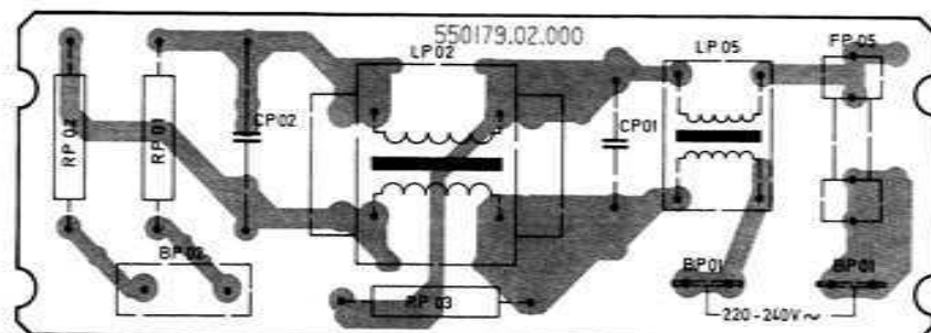
Leiterplatte Netzfilter Piastra bobina d'arresto P.C.B. Mains filter 527.436
