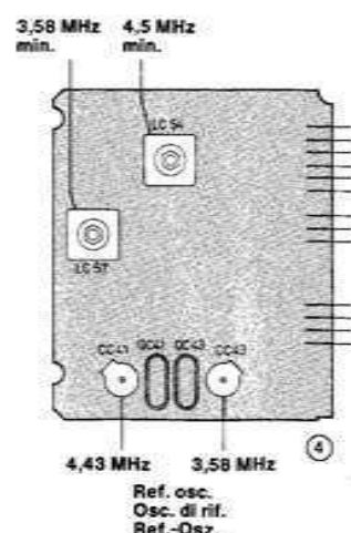
NTSC-Modul Modulo NTSC NTSC-Module Bestückungsseite - Lato componenti - Component side
