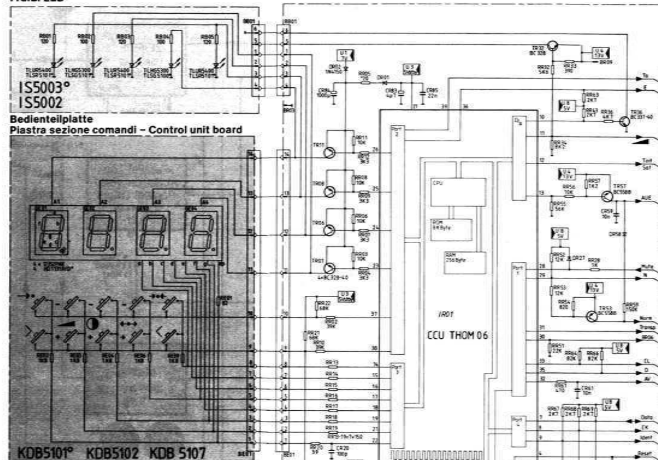
Bedienteilplatte Piastra sezione comandi - Control unit board
