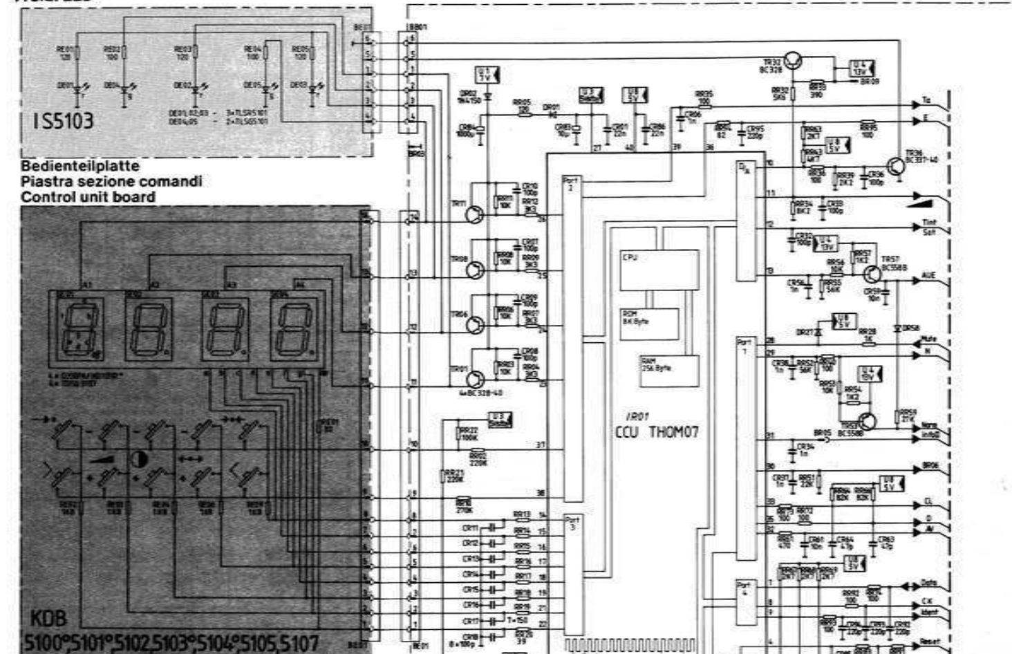
Bedienteilplatte Piastra sezione comandi Control unit board KDB 5100°5101°5102°5103°5104°5105°5107
