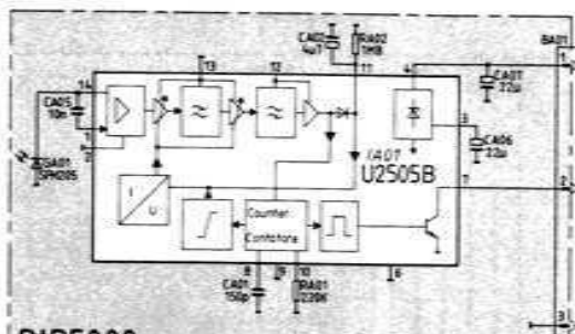
Infrarot-Vorverstärker Preamplificatore infrarossi Infra-red pre-amplifier 583.557
