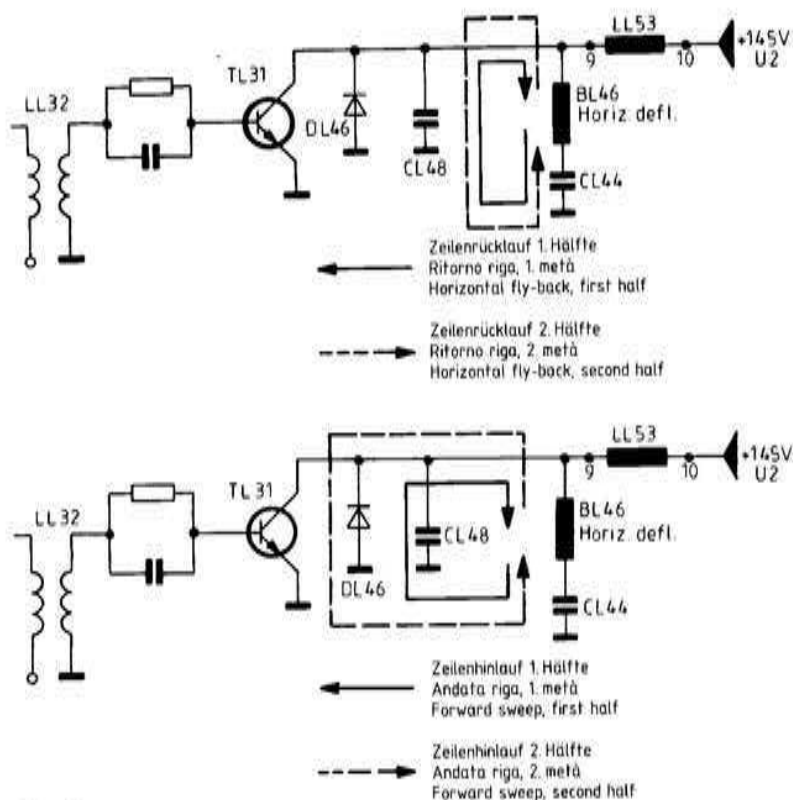
Fig. 13 Principalschaltbild H-Ablenkstufe Schema di principio stadio deflessione orizzontale Schematic circuit diagram of horizontal deflection stage
