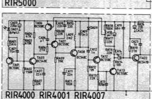
Infrarot-Vorverstärker Preamplificatore infrarossi Infra-red pre-amplifier 583.521 B/C
