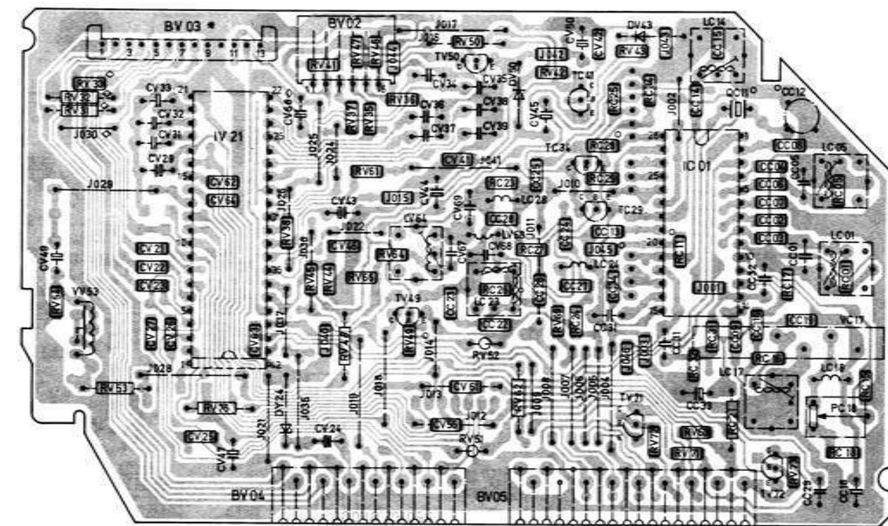
Chroma-Video-Modul Modulo crominanza video Chroma video module Lötseite - Lato saldature - Soldered side
