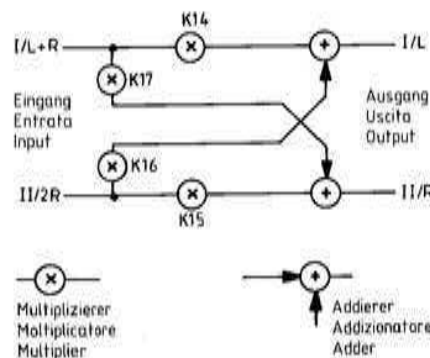
Fig. 8 Dematrixierung Dematrixazione Dematrixing
