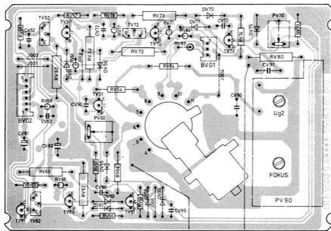
Bildrohrranschluß-Platine Piastra zoccolo cinescopio P.C.B. CRT socket 592.908 Lötseite - Lato saldature - Soldered side
