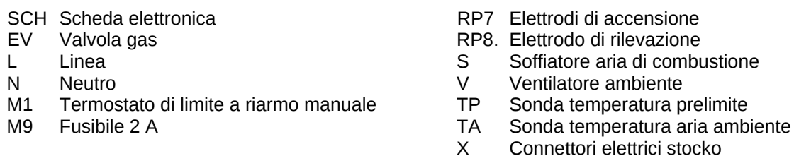
Figura 14 – Schema elettrico
